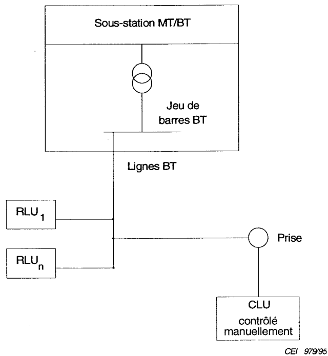
Figure 8 – Lecture locale via le secteur
