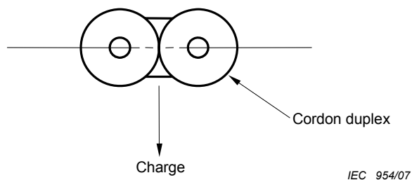
Figure 2 – Application de la charge dans le cas d'un cordon double
