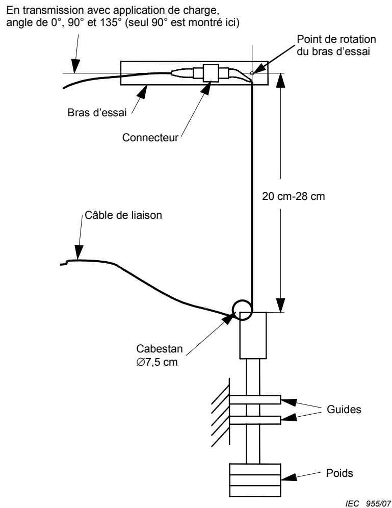
Figure 1 – Appareillage d'essai en transmission lorsqu'une charge de traction est appliquée
