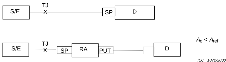
Figure 3 – Méthode d'essai
