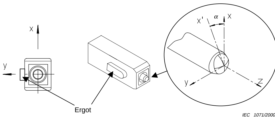
Figure 2 – Orientation préférentielle du secteur d'ajustement pour certaines constructions – Exemple de schéma de connecteur angulaire
