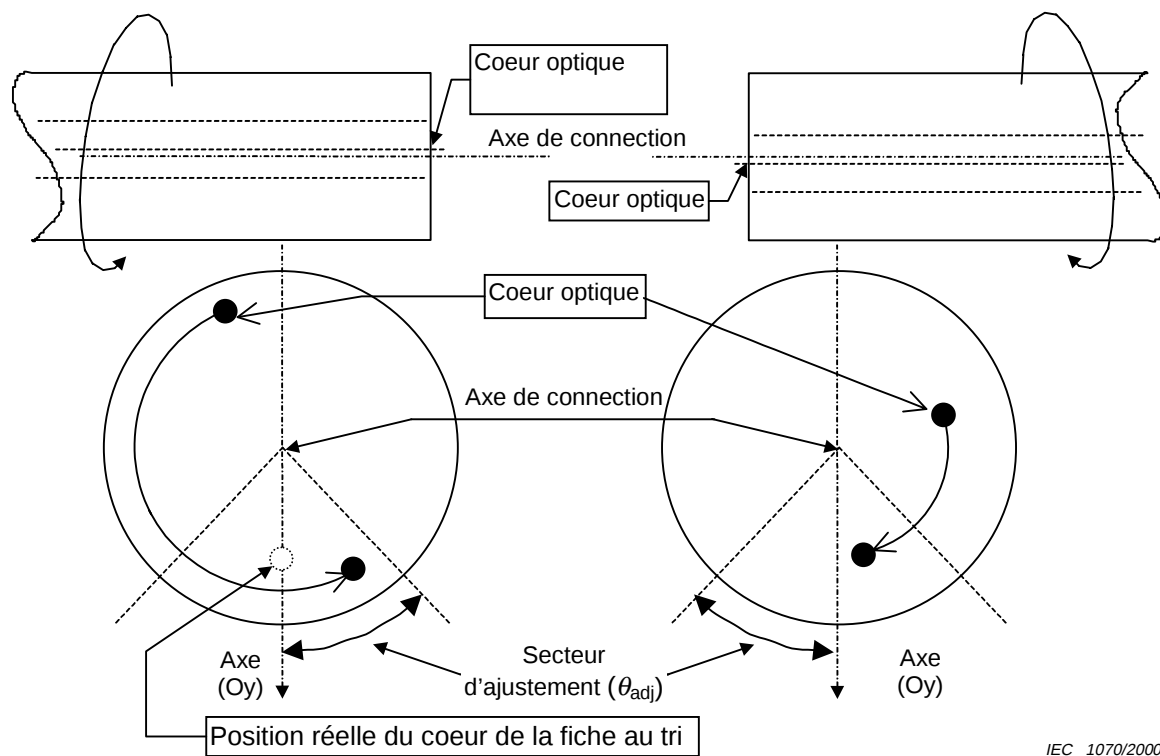
Figure 1 – Secteur d'ajustement et position réelle de la fiche de référence
