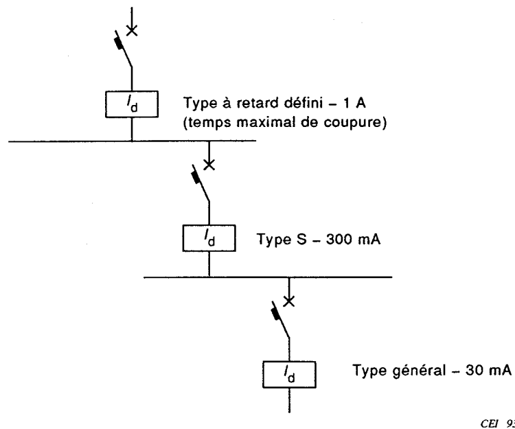
Figure 3 – Exemple de circuits avec deux niveaux de sélectivité
