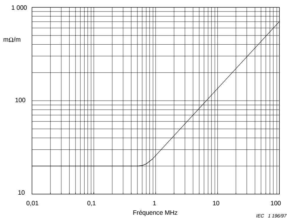
Figure 1 – Impédance de transfert maximale
