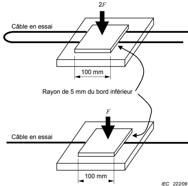
Figure 1 – Equipement pour l'essai d'écrasement
