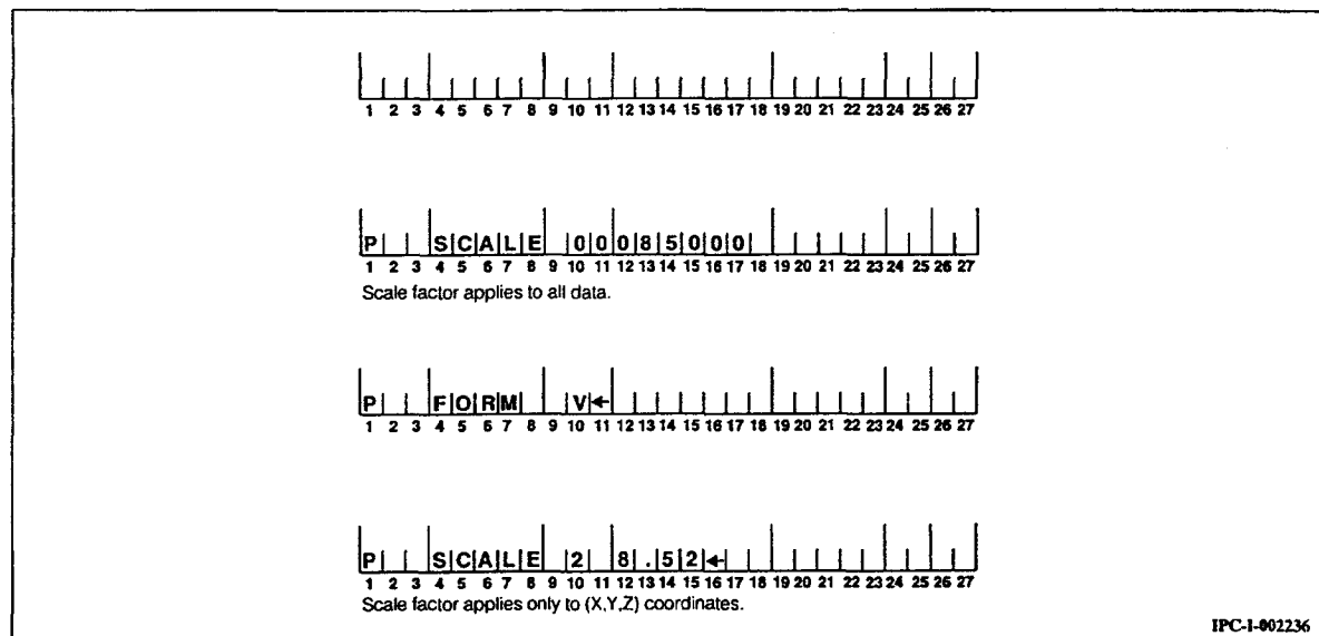
Figure 5-9 - Parameter SCALE
