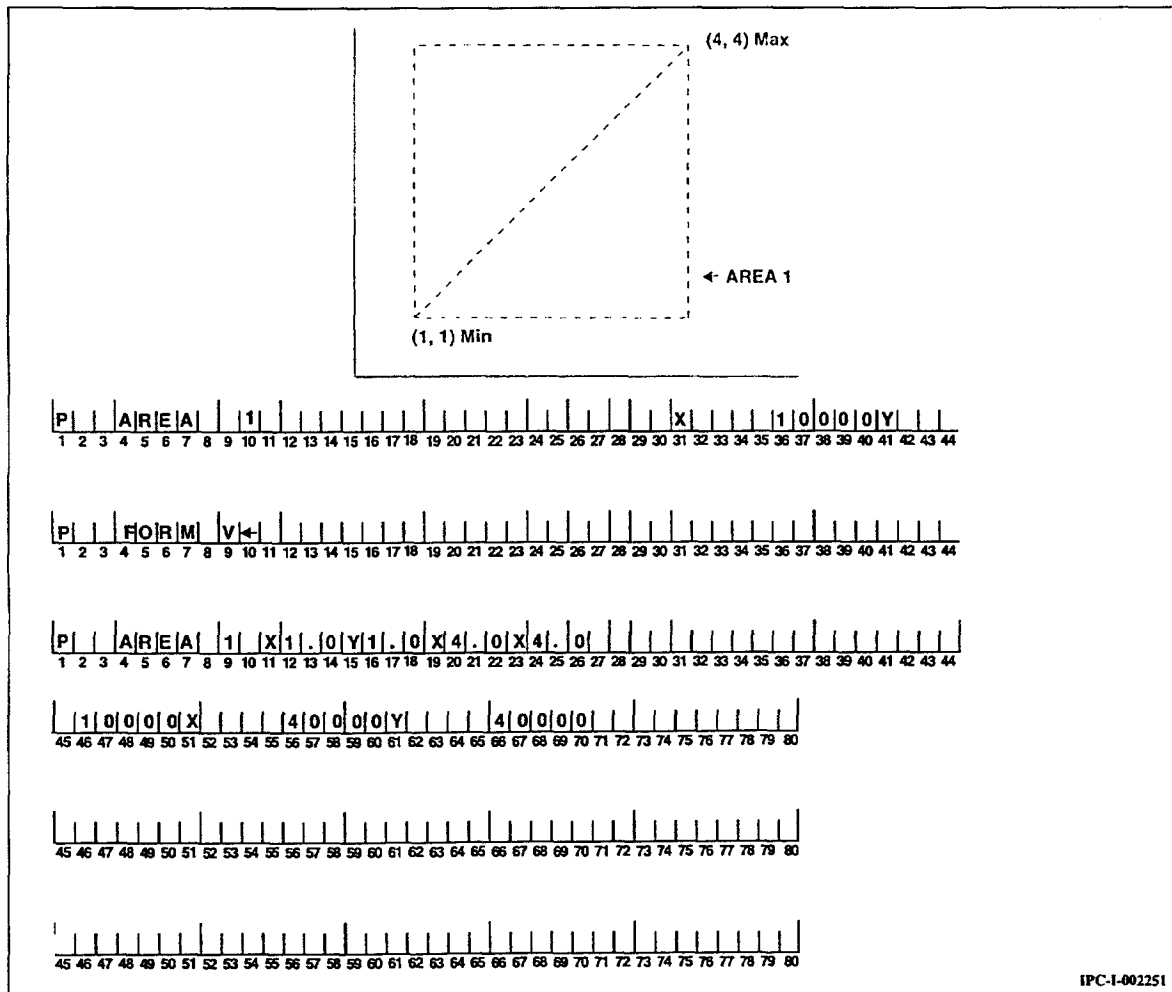
Figure 5-11 - Parameter AREA
