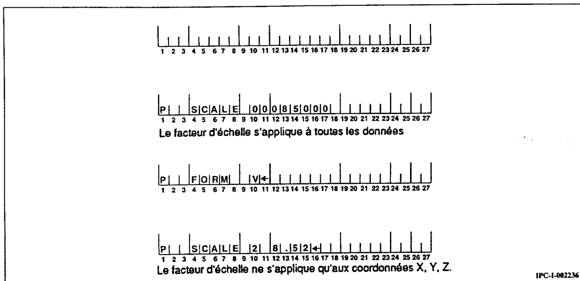
Figure 5-9 - Paramètre SCALE
