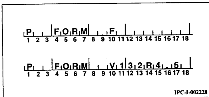
Figure 5-2 - Paramètre FORM
