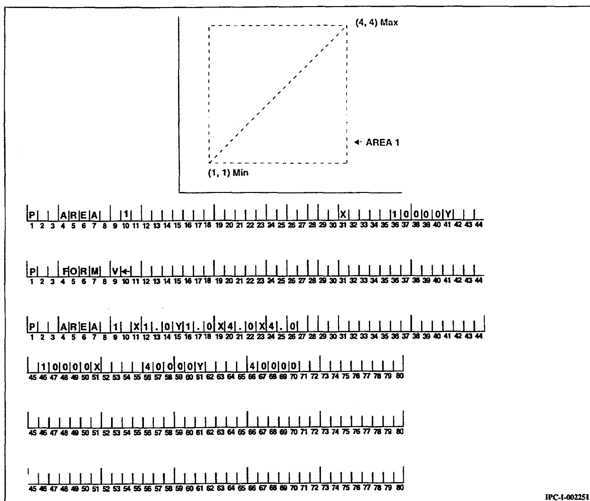
Figure 5-11 - Paramètre AREA
