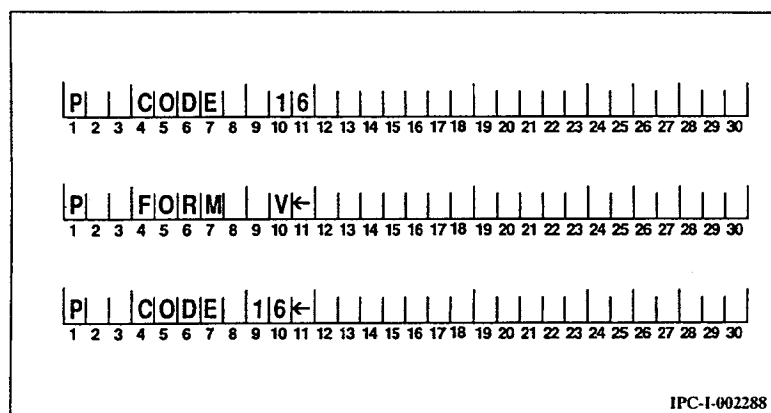
Figure 5-3 - Parameter CODE
