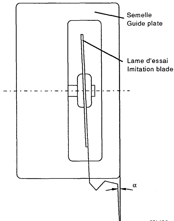
Figure 2 – Précision de coupe Cutting accuracy
