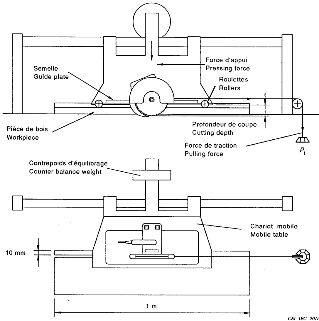
Figure 7 – Montage d'essai Test rig
