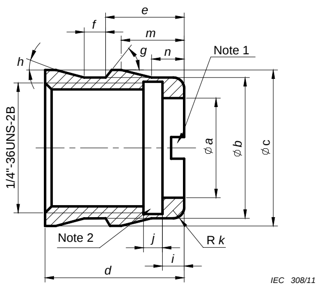
Figure A.1 – Pièce complémentaire (pour les dimensions et les notes, voir le Tableau A.1)
