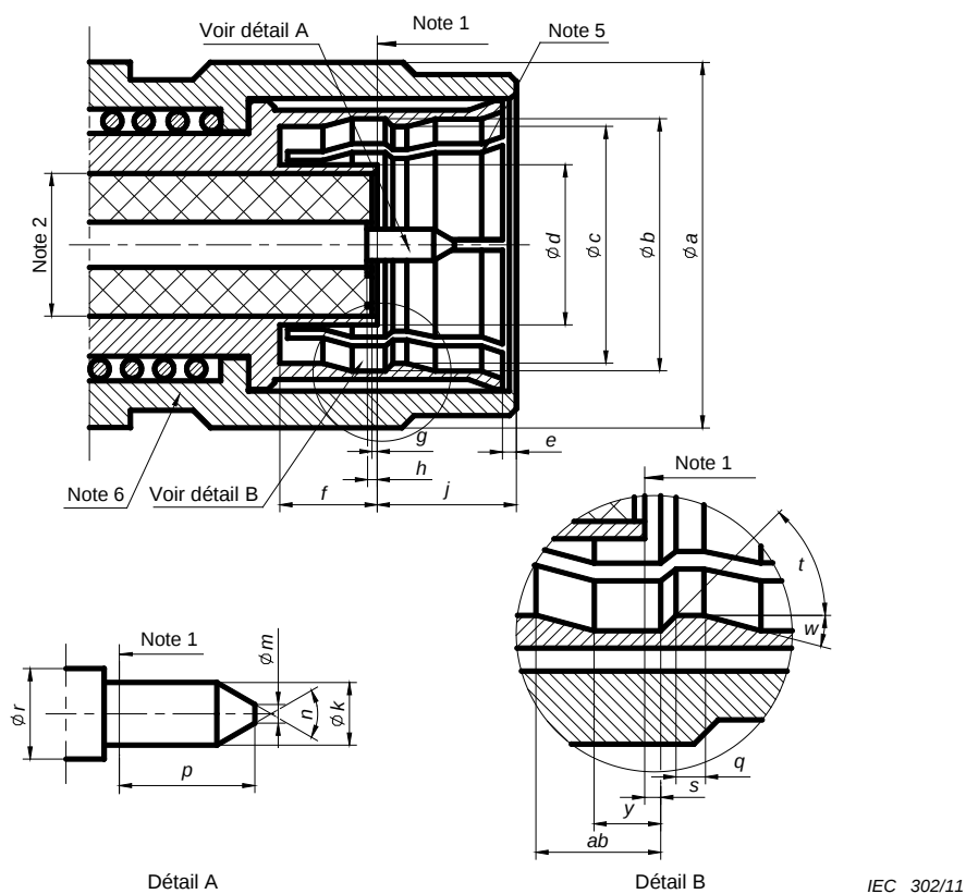
Figure 1 – Connecteur avec contact central mâle (pour les dimensions et les notes, voir le Tableau 1)
