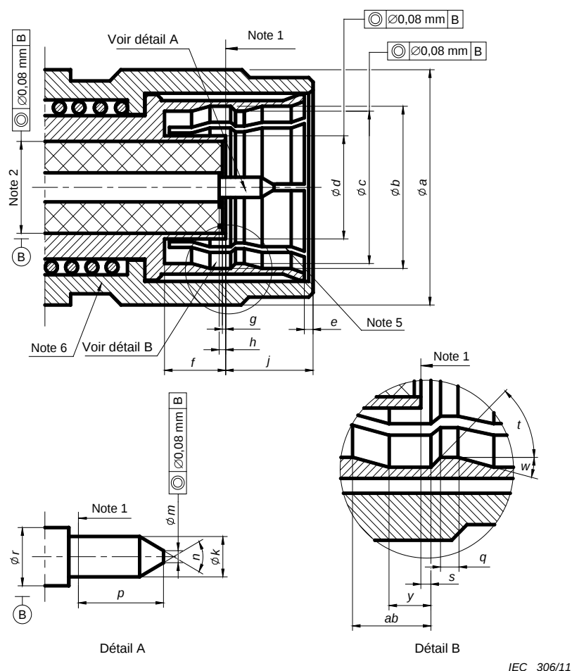
Figure 5 – Connecteur avec contact central mâle (pour les dimensions et les notes, voir le Tableau 5)
