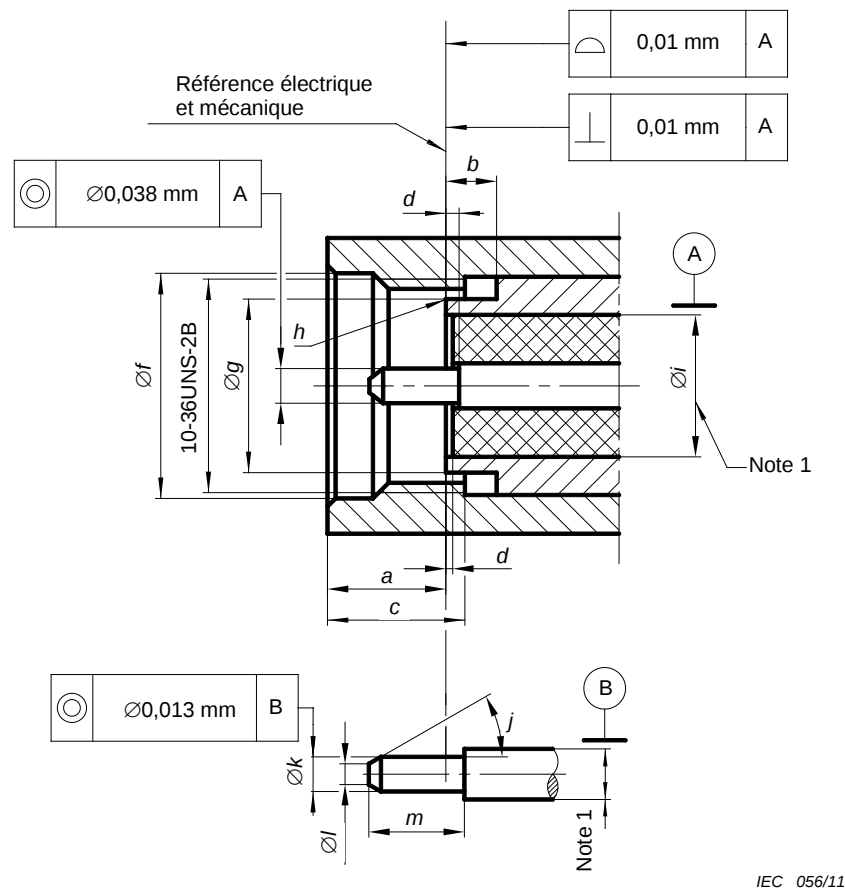
Figure 4 – Connecteur avec contact central mâle (pour les dimensions et les notes, voir le Tableau 4)
