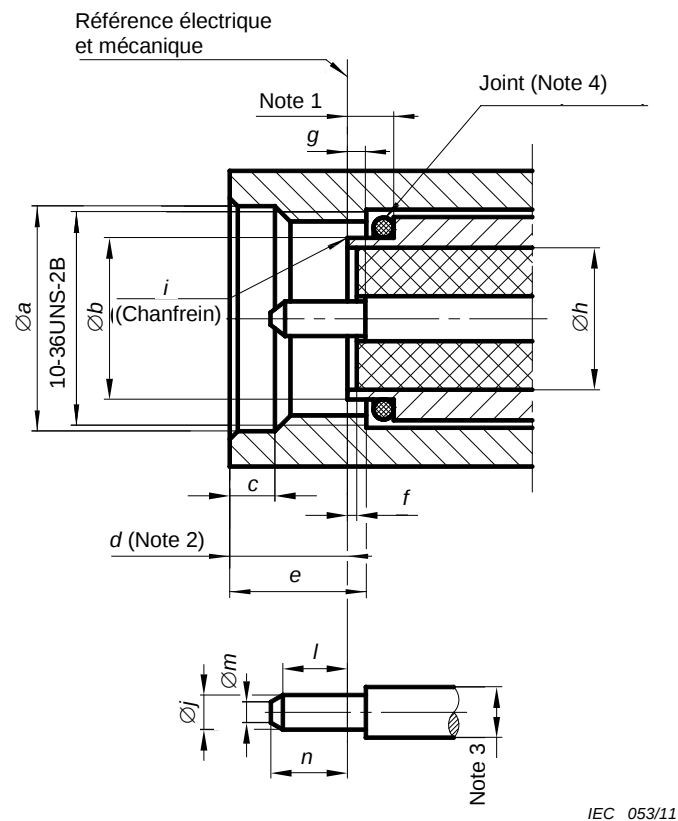
Figure 1 – Connecteur avec contact central mâle (pour les dimensions et les notes, voir le Tableau 1)
