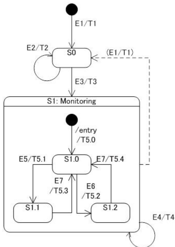
Figure 29 – Schéma d'états de l'ARPM-FDCMN
