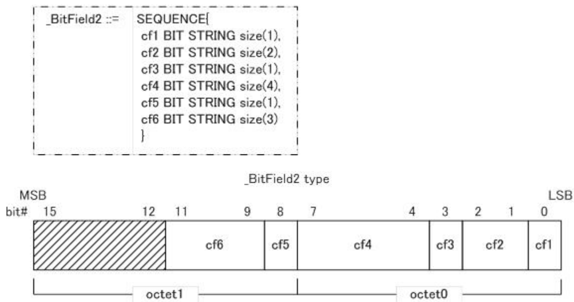
Figure 8 – Exemple de définition de champ binaire avec taille de champ
