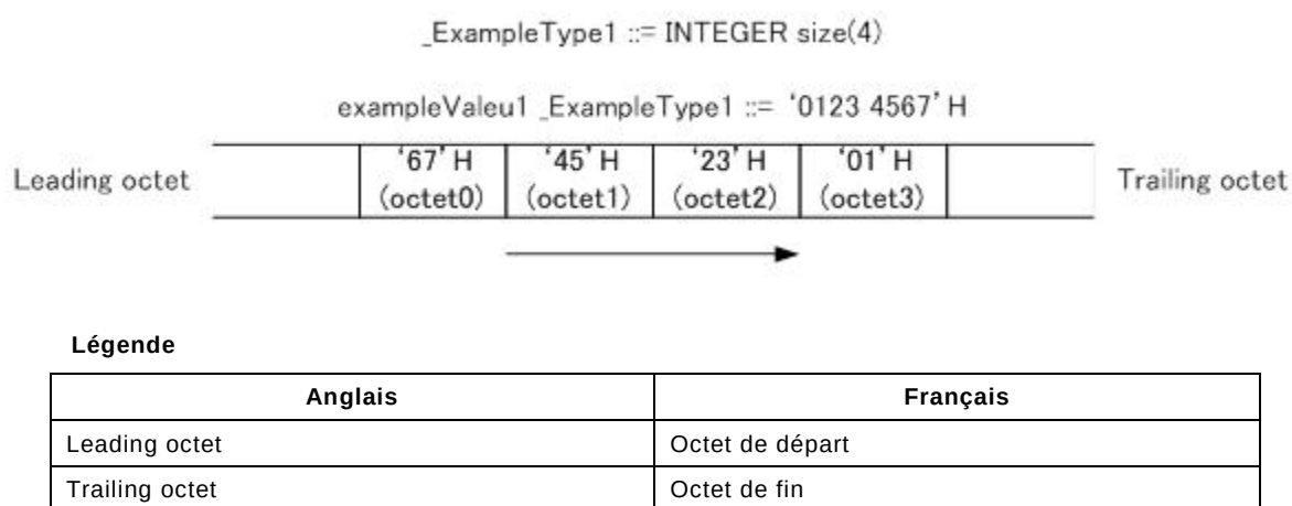
Figure 3 – Exemple de transfert de la valeur INTEGER
