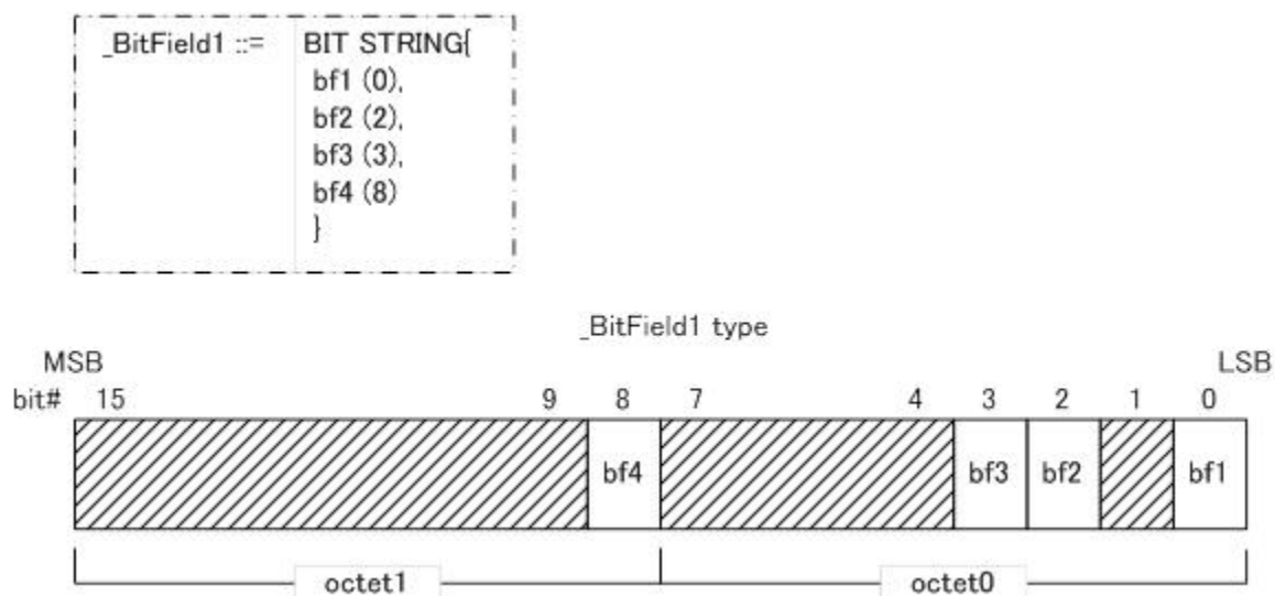
Figure 7 – Exemple de définition de champ binaire avec bits nommés
