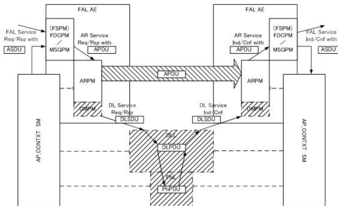
Figure 10 – Structure des diagrammes d'états de protocole FAL
