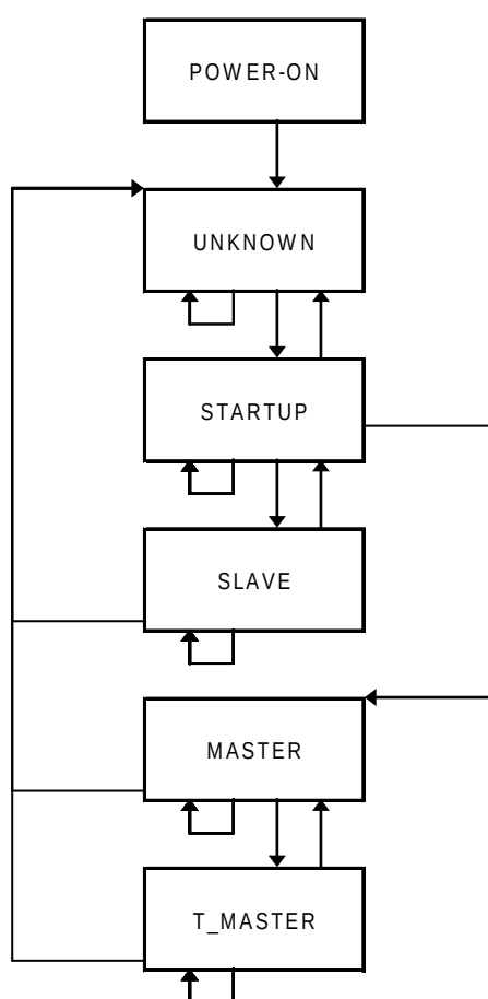
Figure 43 – Schéma de transition d'états de SYN_BMA
