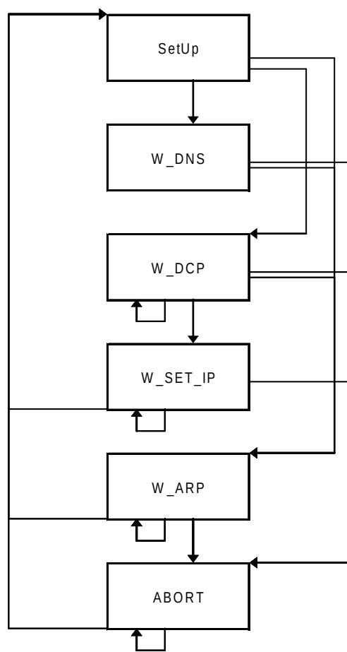
Figure 124 – Schéma de transition d'états de CTLDINA
