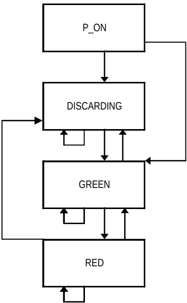
Figure 78 – Schéma de transition d'états de DEMUX
