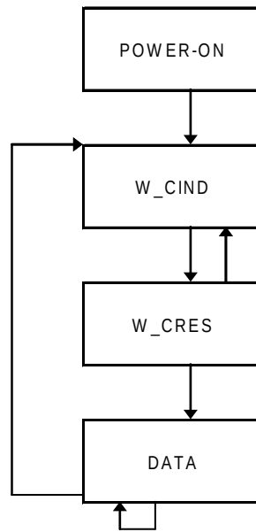
Figure 102 – Schéma de transition d'états de CMDEV_DA
