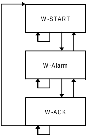
Figure 96 – Schéma de transition d'états d'ALPMI
