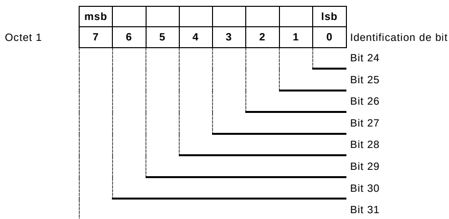
Figure 4 – Structure commune de champs spécifiques pour l'octet 1 (élevé)
