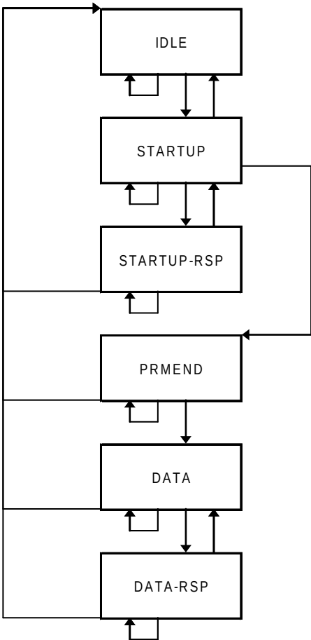
Figure 105 – Schéma de transition d'états de CMWRR
