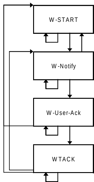
Figure 97 – Schéma de transition d'états d'ALPMR
