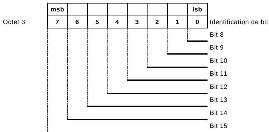
Figure 6 – Structure commune de champs spécifiques pour l'octet 3
