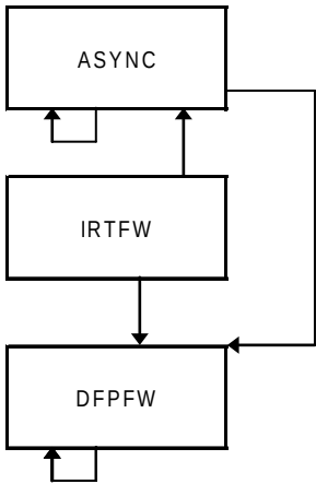
Figure 73 – Schéma de transition d'états de DFP_RELAY
