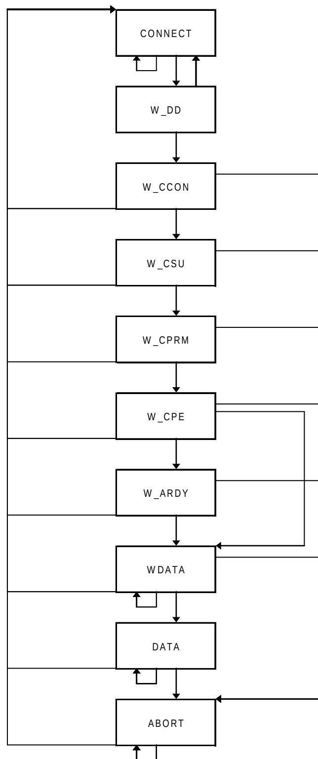
Figure 114 – Schéma de transition d'états de CMCTL
