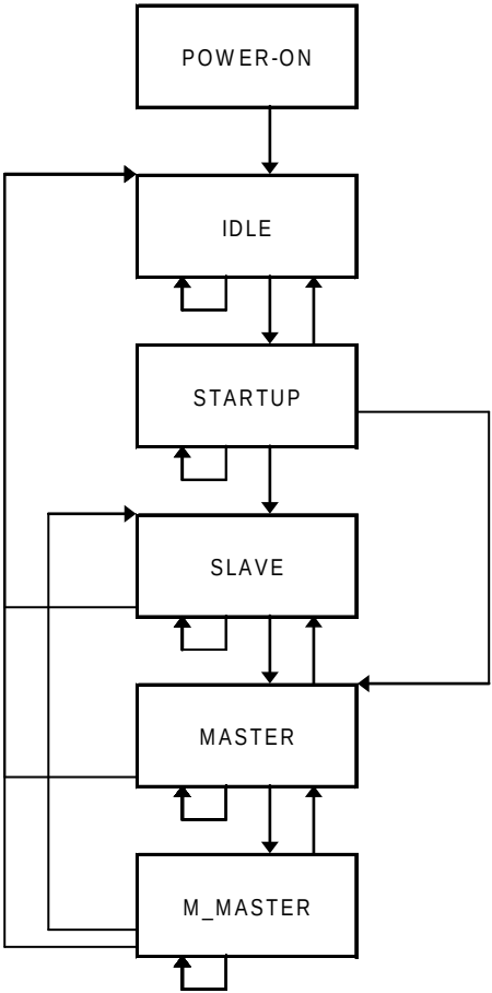
Figure 44 – Schéma de transition d'états de SYN_MPSM
