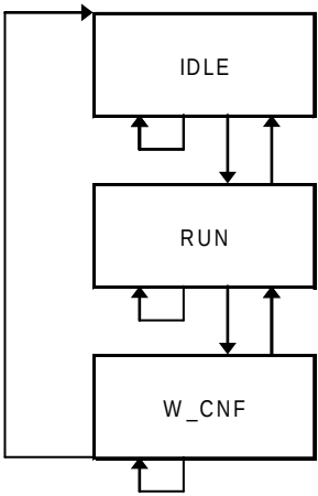
Figure 117 – Schéma de transition d'états de CTLRDI
