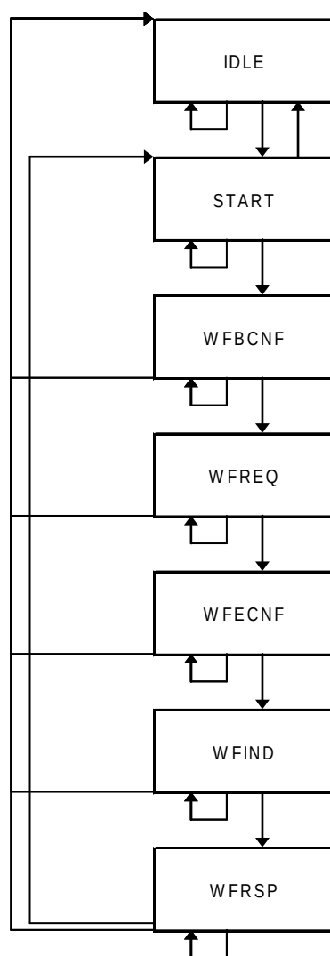
Figure 123 – Schéma de transition d'états de CTLPBE
