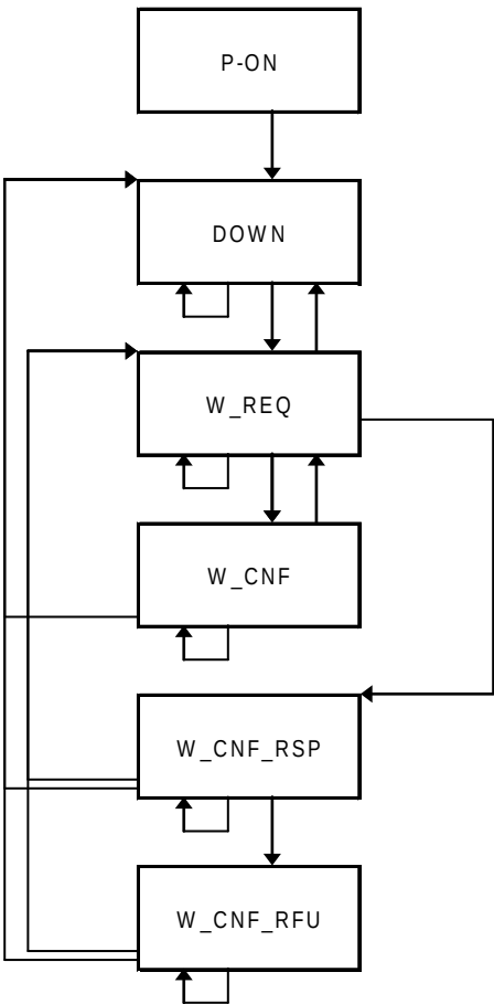
Figure 41 – Schéma de transition d'états de DELAY_RSP
