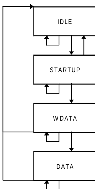
Figure 116 – Schéma de transition d'états de CTLIO
