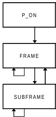
Figure 74 – Schéma de transition d'états de DFP_RELAY_INBOUND
