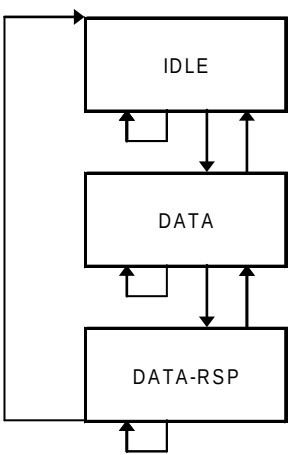
Figure 122 – Schéma de transition d'états de CTLWRR
