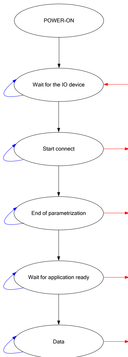
Figure 113 – Schéma de transition d'états de IO controller CM (CM d'appareil de commande E/S)
