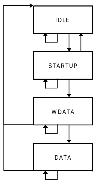
Figure 104 – Schéma de transition d'états de CMIO
