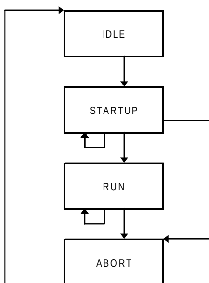
Figure 103 – Schéma de transition d'états de CMSU
