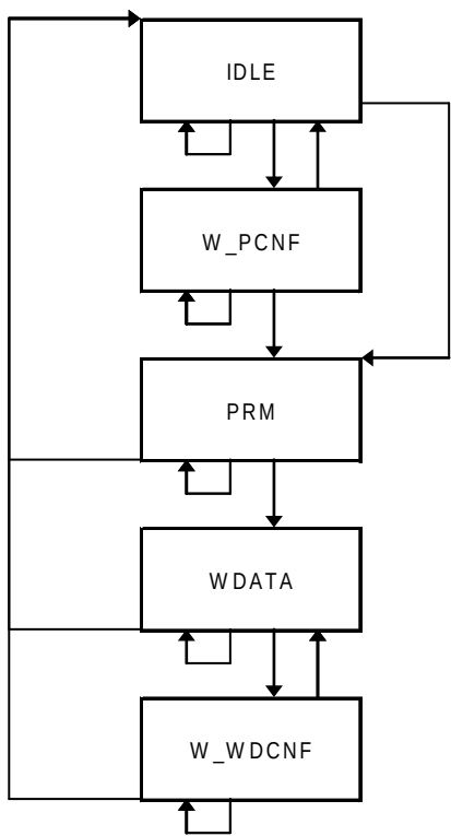
Figure 121 – Schéma de transition d'états de CTLWRI
