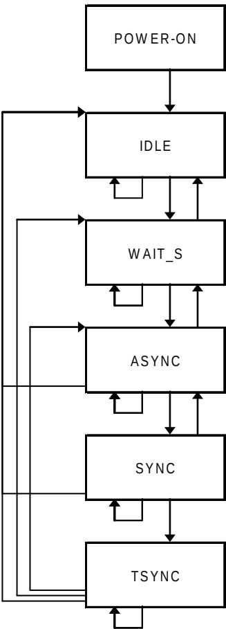
Figure 45 – Schéma de transition d'états de SYN_SPSM
