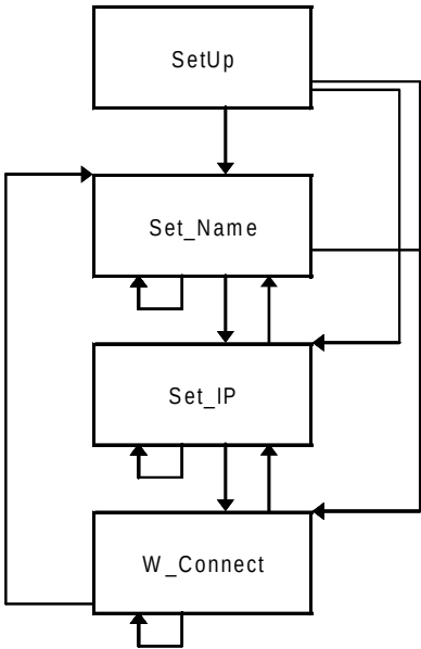
Figure 110 – Schéma de transition d'états de CMINA
