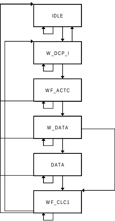
Figure 109 – Schéma de transition d'états de CMDMC
