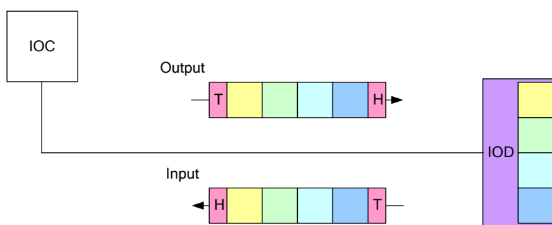
Figure N.4 – End node mode
