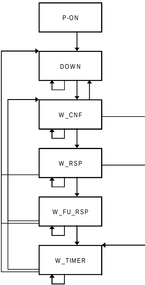
Figure 40 – Schéma de transition d'états de DELAY_REQ
