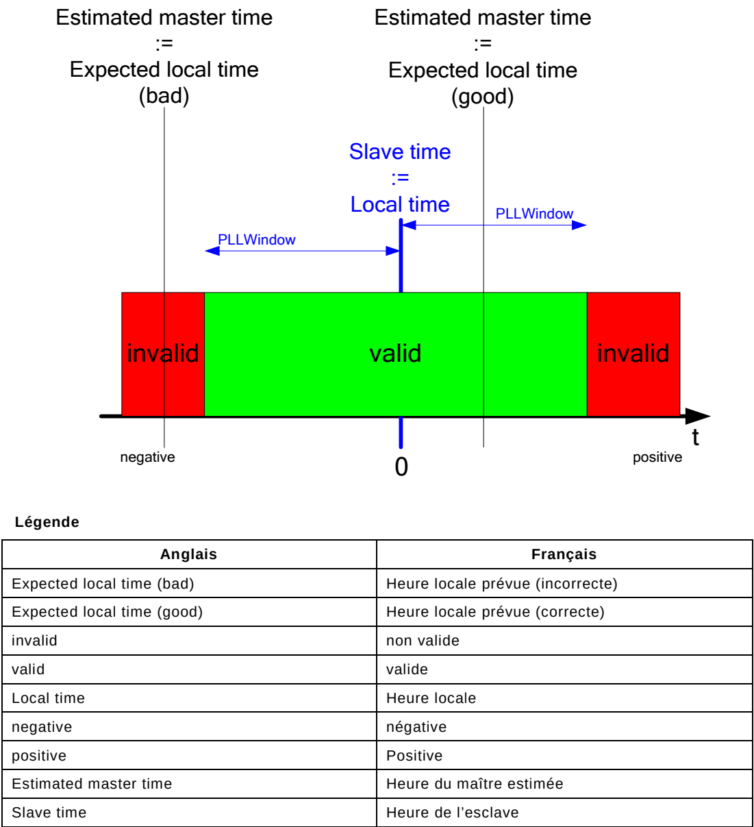
Figure 88 – Définition de PLL window
