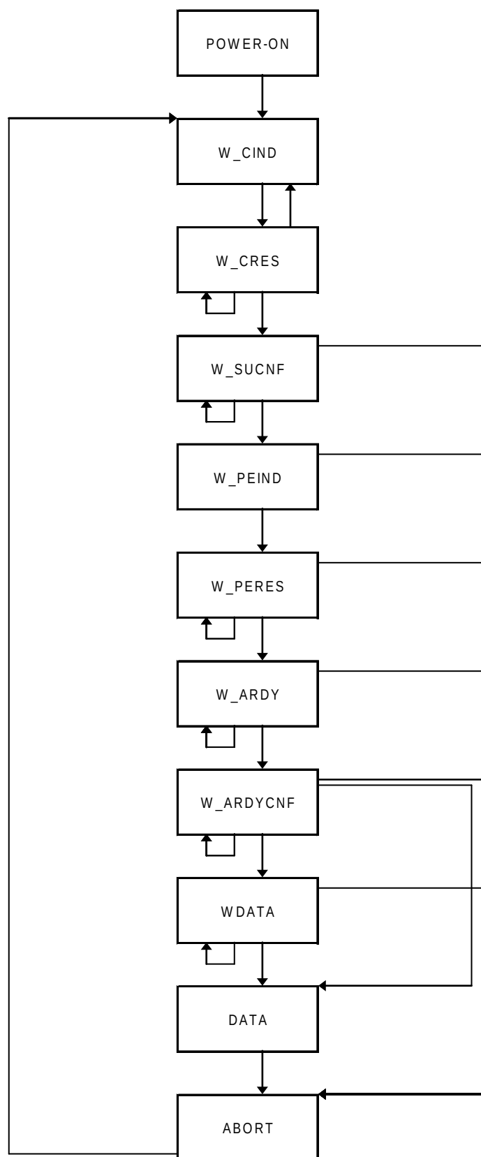
Figure 100 – Schéma de transition d'états de CMDEV
