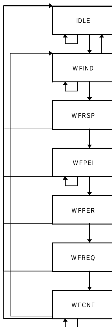
Figure 108 – Schéma de transition d'états de CMPBE
