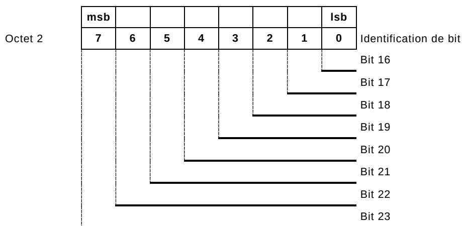
Figure 5 – Structure commune de champs spécifiques pour l'octet 2
