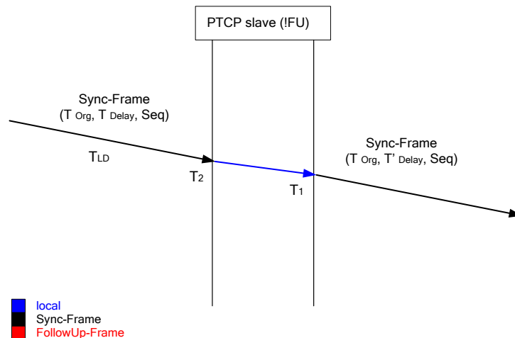
Figure 36 – Esclave de synchronisation !FU transférant une Sync-Frame (trame de synchronisation)
