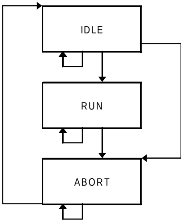
Figure 120 – Schéma de transition d'états de CTLSU
