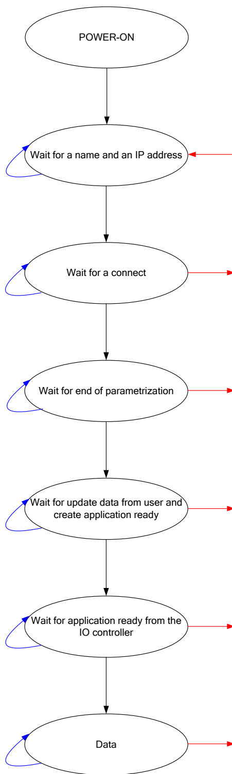
Figure 99 – Schéma de transition d'états du CM d'appareil E/S
