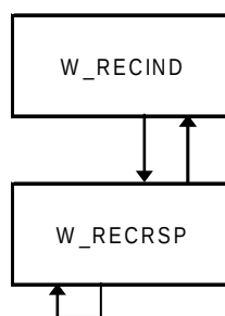
Figure 118 – Schéma de transition d'états de CTLRDR
