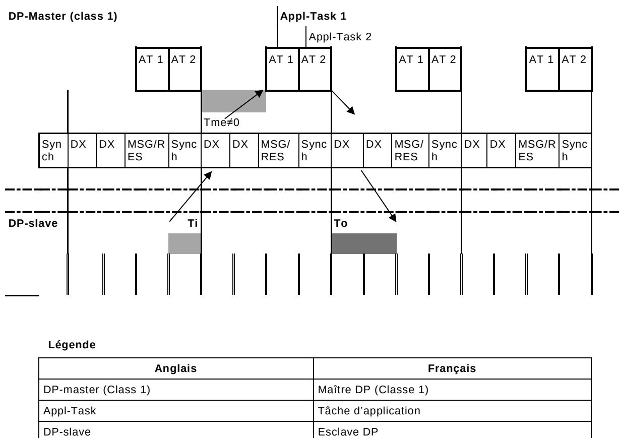
Figure 17 – Système de DP avec cycle de DP isochrone optimisé
