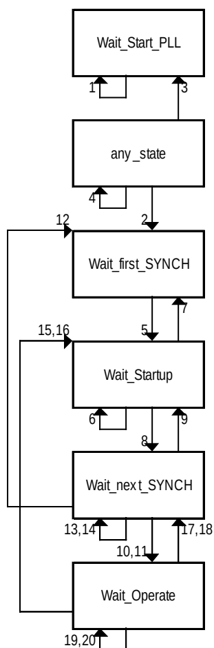
Figure 21 – Diagramme d'états de PLL
