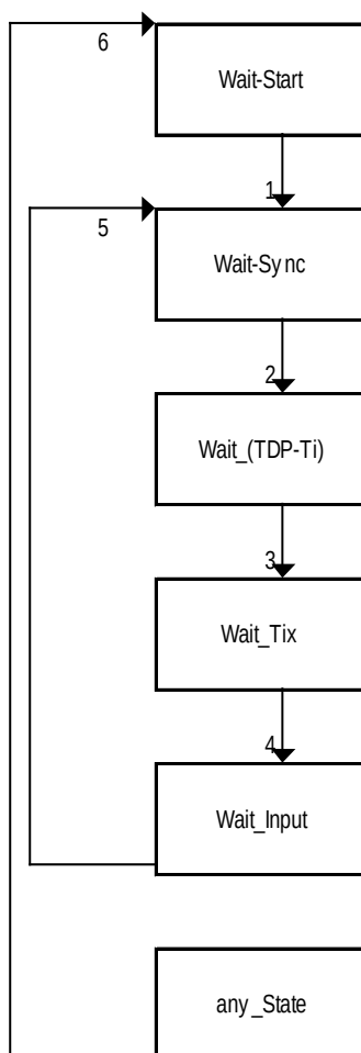
Figure 23 – Diagramme d'états de l'INPUT
