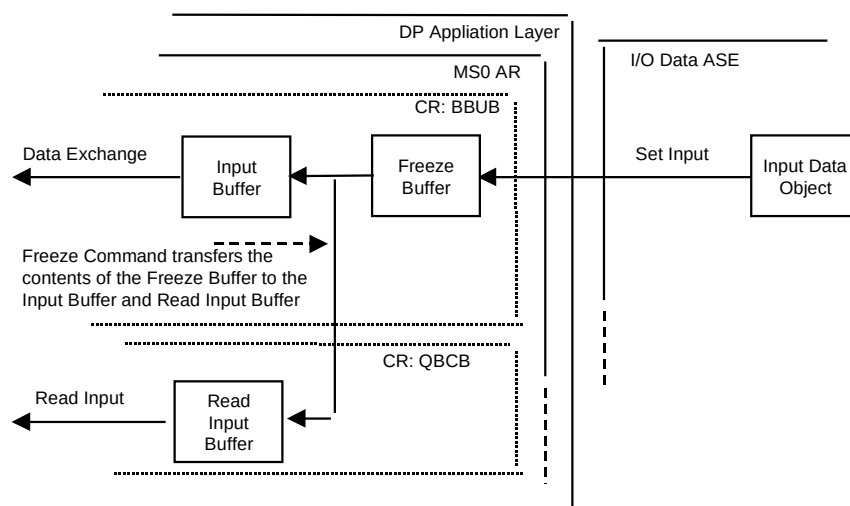
Figure 33 – Modèle de tampon d'entrées d'un esclave DP sans fonctionnalité freeze
