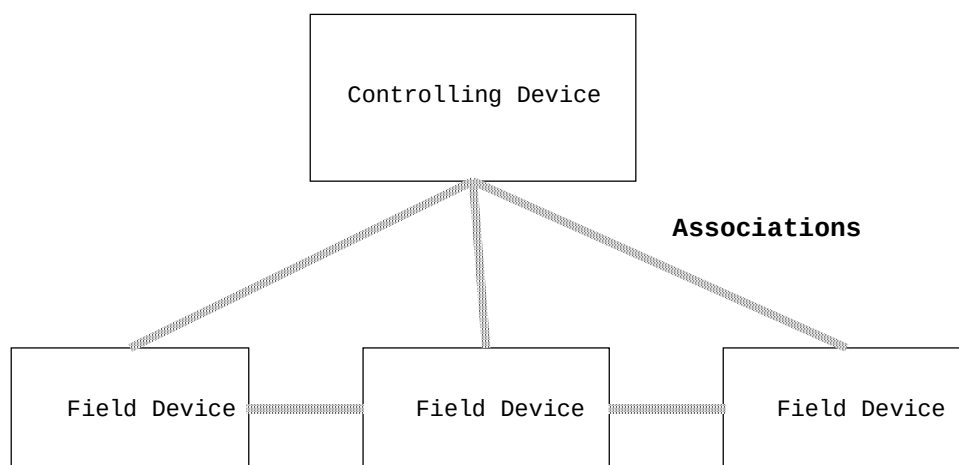
Figure 2 – Exemple de communication DP avec plusieurs appareils de commande
