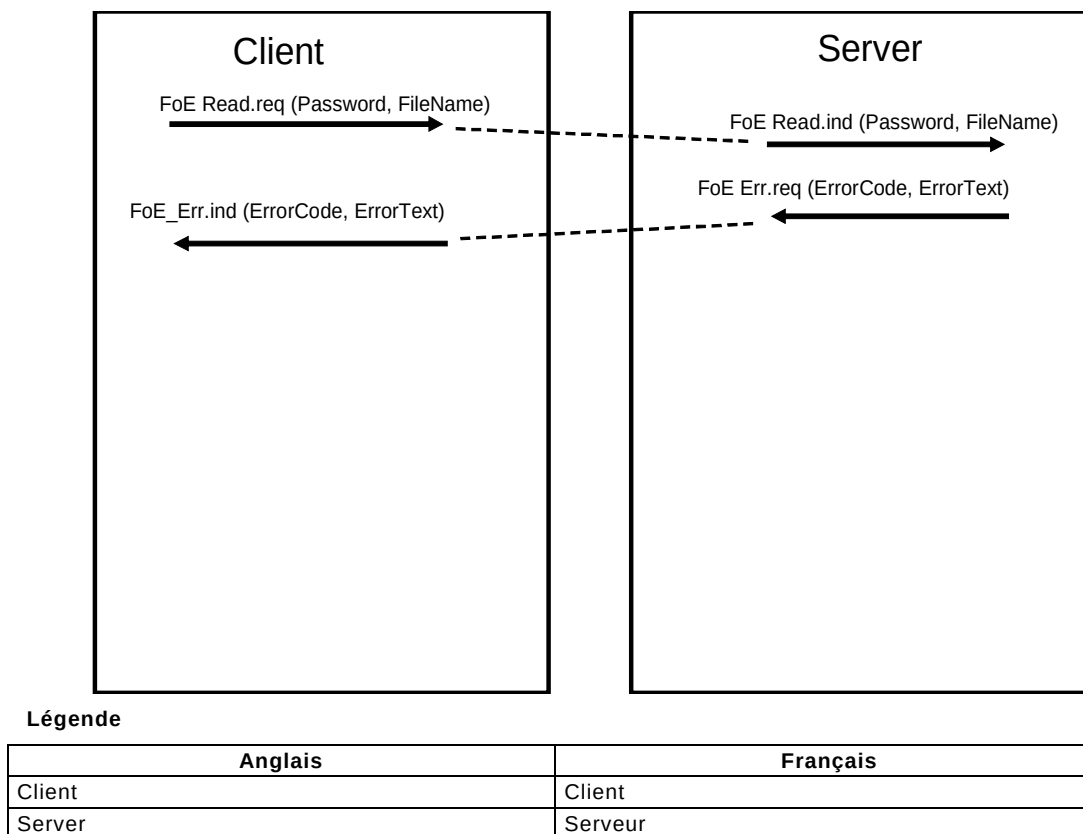
Figure 28 – Séquence "FoE read" avec erreur
