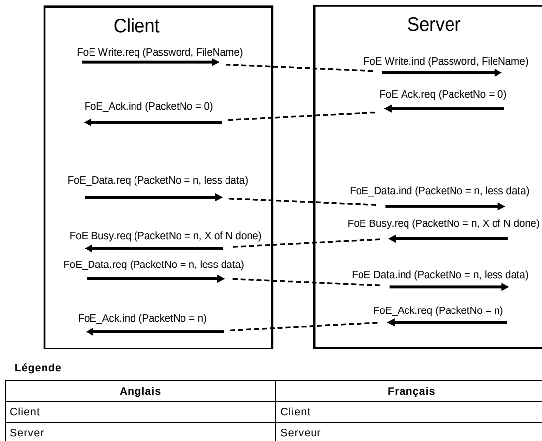
Figure 31 – Séquence "FoE write" avec occupation
