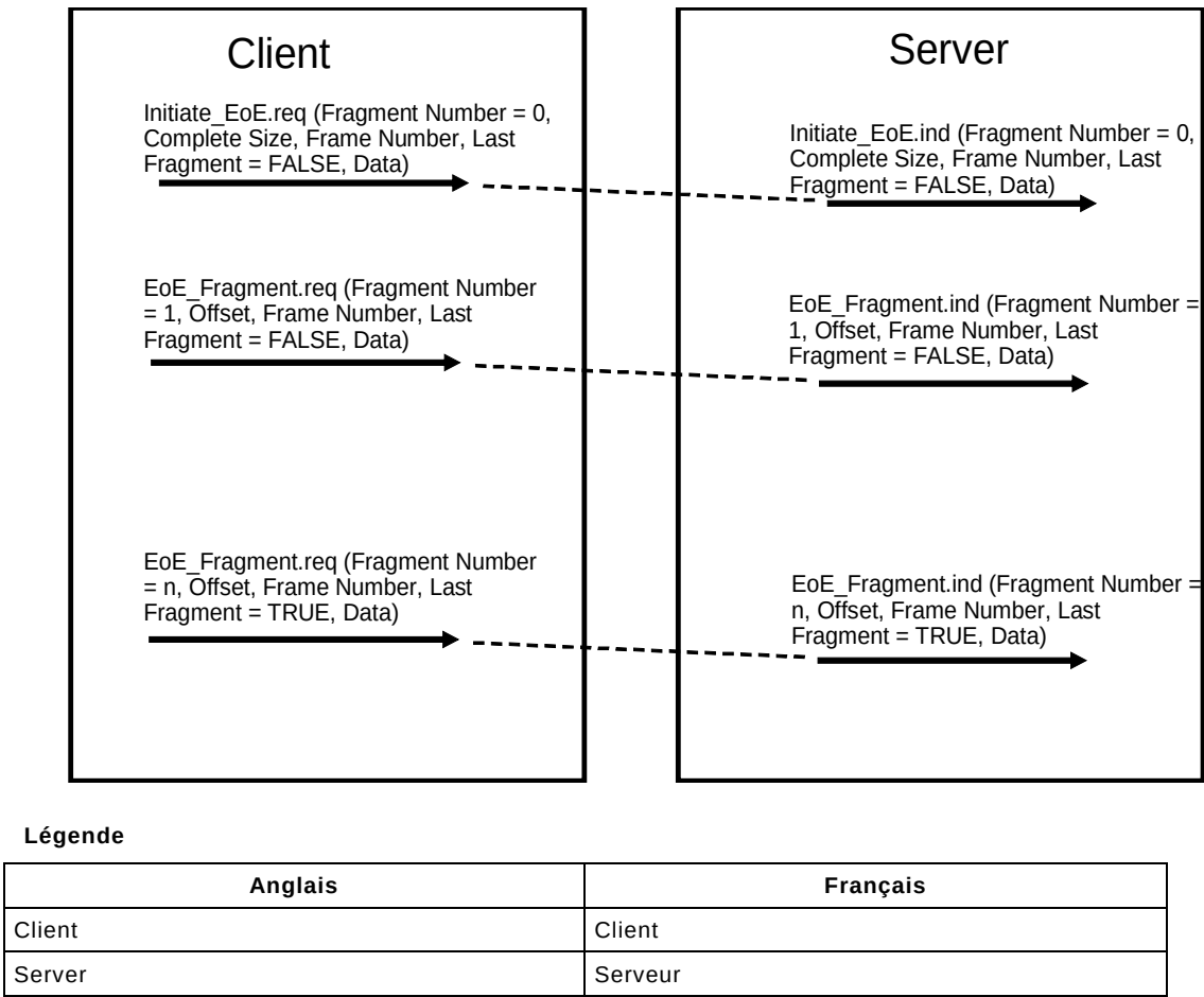
Figure 26 – Séquence "EoE"
