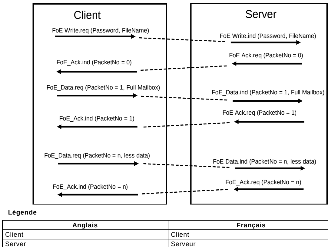
Figure 29 – Séquence "FoE write" avec succès
