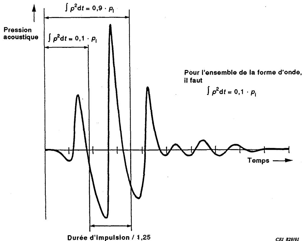
Figure 3 - Schéma indiquant la méthode de détermination de la durée d'impulsion.
