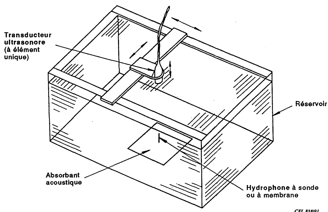
Figure 12 - Schéma de montage d'un transducteur ultrasonore et d'un hydrophone, représentés avec un nombre limité de degrés de liberté de translation et de rotation.
