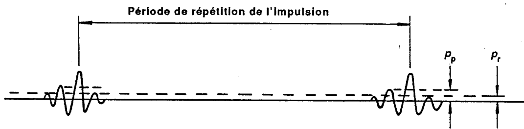
Figure 7 - Schéma représentant les paramètres pression acoustique sur l'impulsion et pression acoustique efficace.
