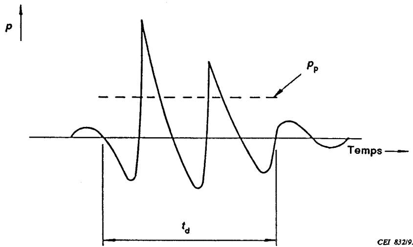
Figure 6 - Schéma représentant le paramètre pression acoustique moyenne sur l'impulsion.
