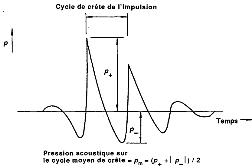
Figure 5 - Schéma représentatif des paramètres crête impulsion.
