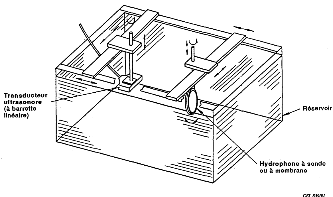
Figure 13 - Schéma de montage d'un transducteur ultrasonore et d'un hydrophone, représentés avec une gamme complète de degrés de liberté.
