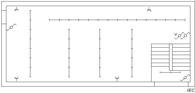
c) Dessin de base avec ajout de l'installation d'éclairage
