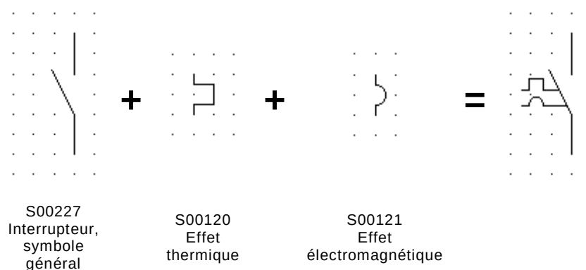
Figure A.5 – Disjoncteur miniature représenté avec le symbole général pour un interrupteur qualifié avec les symboles pour les effets thermique et électromagnétique
