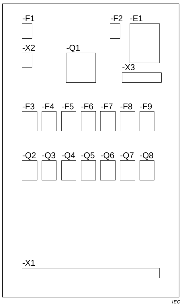
Figure 89 – Dessin d'installation du panneau de montage d'une armoire
