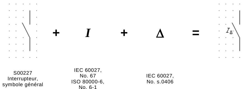
Figure A.10 – Exemple de symbole pour DDR
