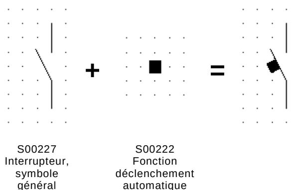
Figure A.3 – Disjoncteur miniature représenté avec le symbole général pour un interrupteur qualifié avec le symbole pour le déclenchement automatique
