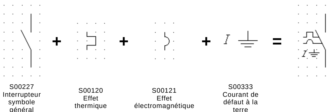
Figure A.7 – Symbole pour un disjoncteur miniature avec DDR, version 1
