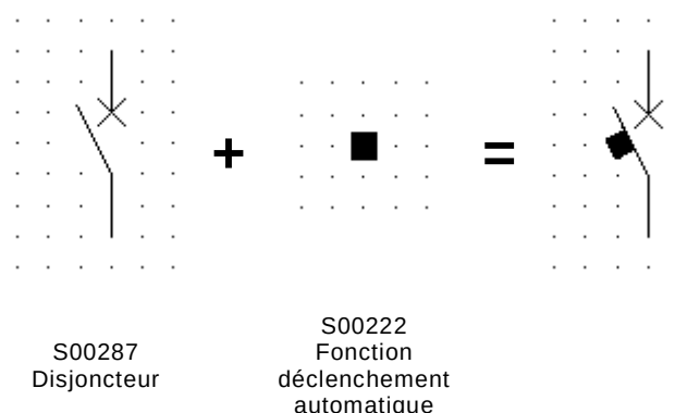
Figure A.4 – Disjoncteur miniature représenté avec le symbole des disjoncteurs qualifié avec le symbole pour le déclenchement automatique
