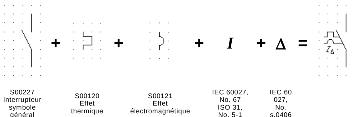
Figure A.9 – Symbole pour un disjoncteur miniature avec DDR, version 3
