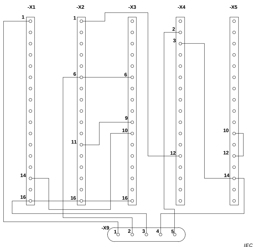
Figure 84 – Exemple de schéma de connexion pour un bac à cartes
