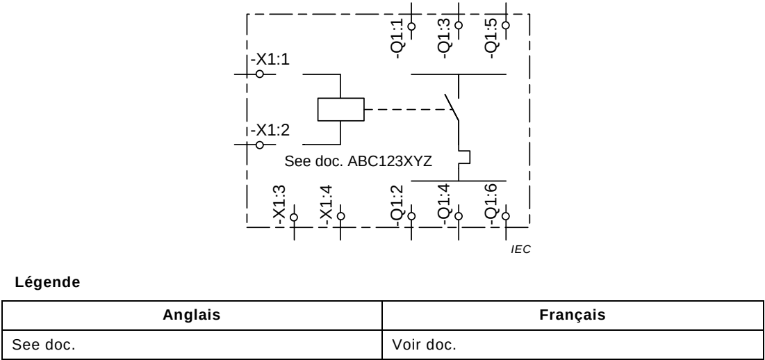
Figure 97 – Exemple de schéma d'exemple d'un démarreur
