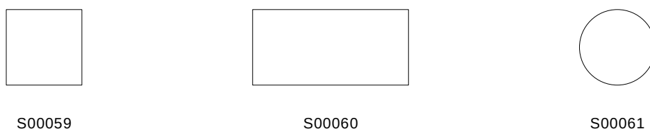
Figure A.1 – Symboles généraux pour un objet dans l'IEC 60617
