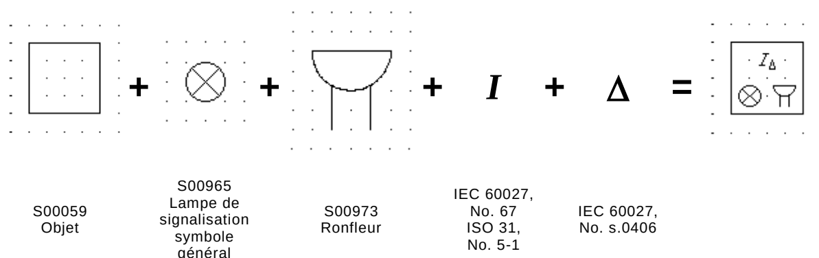
Figure A.11 – Exemple de symbole pour RCM
