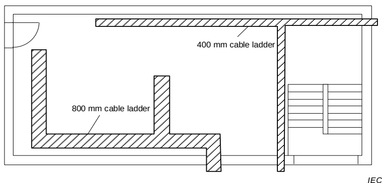
b) Dessin de base avec ajout de cheminement des câbles
