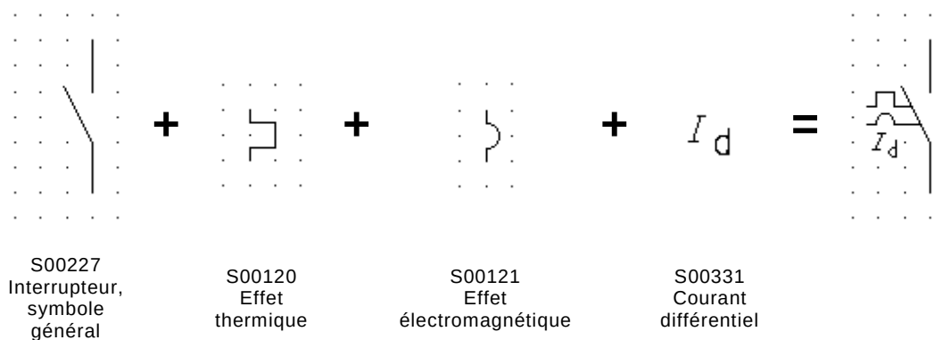
Figure A.8 – Symbole pour un disjoncteur miniature avec DDR, version 2
