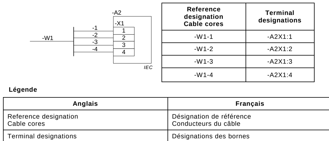
Figure 82 – Exemple de présentation de terminaison d'un câble multiconducteur
