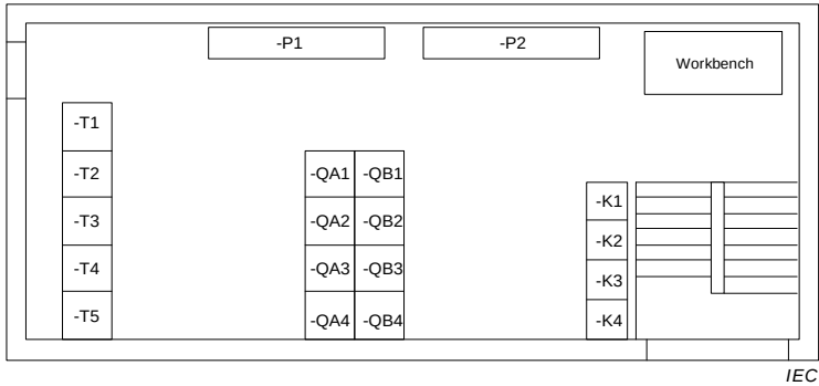
d) Dessin de base avec ajout de l'aménagement des armoires d'appareillage et de télécommunications
