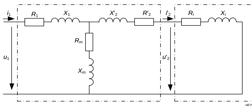
Figure 62 – Exemple de schéma d'équivalence des circuits
