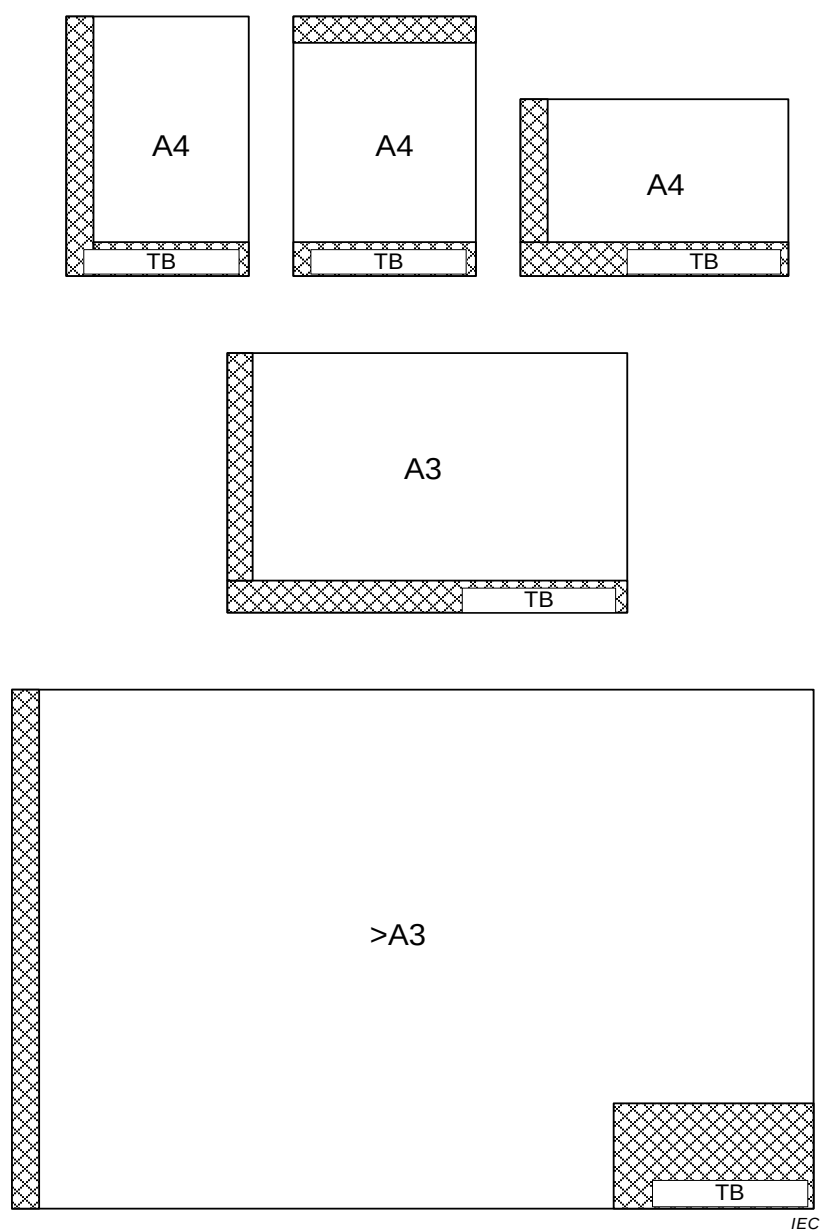
Figure B.3 – Exemples d'emplacements de zones d'identification et de cartouches d'inscriptions possibles
