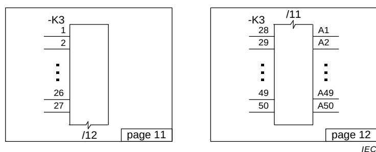
Figure 80 – Exemple de présentation éclatée d'un symbole
