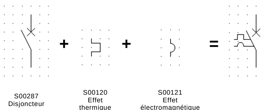
Figure A.6 – Disjoncteur miniature représenté avec le symbole pour un disjoncteur qualifié avec le symbole pour les effets thermique et électromagnétique
