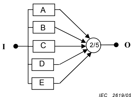
Figure 16 – 2 sur 5 système non identique
