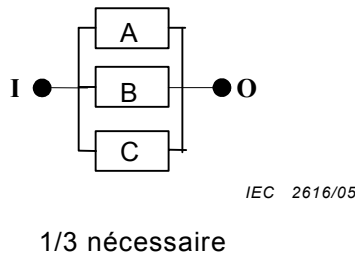
Figure 13 – Arrangement parallèle avec une entité opérationnelle nécessaire sur trois
