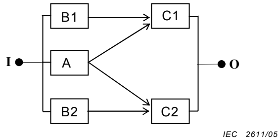
Figure 8 – Bloc diagramme non représenté facilement par un arrangement de blocs série/parallèle
