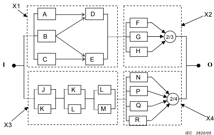
Figure 17 – Illustration de groupements de blocs avant réduction
