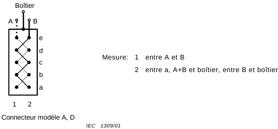
Figure 19 – Câblage d'un spécimen
