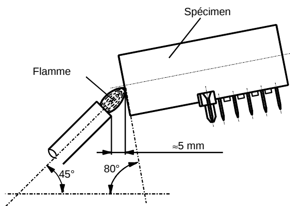
Figure 21 – Montage pour l'essai d'inflammabilité
