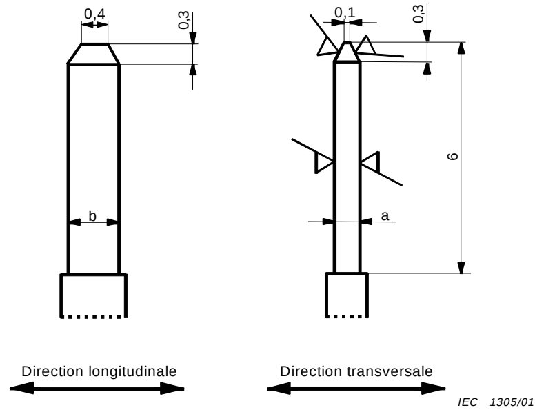
Figure 15 – Calibres de dimensionnement et de force de rétention pour contacts femelles
