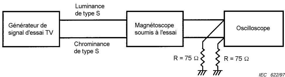
Figure 31 – Synoptique pour un signal d'entrée vidéo de type S
