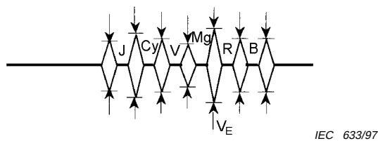
Figure 42 – Mesures du niveau des signaux
