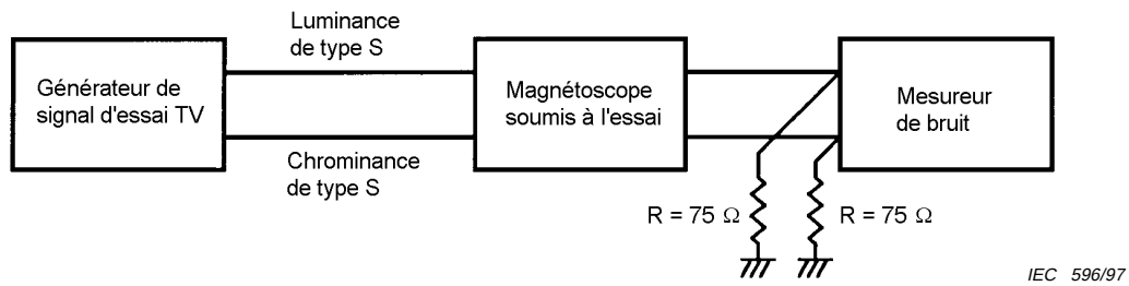
Figure 5 – Synoptique pour une entrée vidéo de type S
