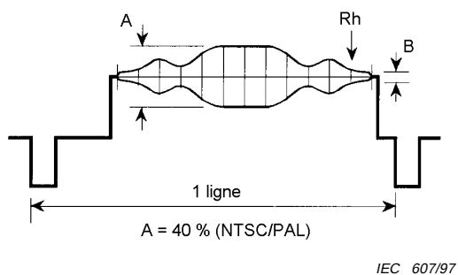
Figure 16 – Forme d'onde pour un signal d'entrée composite
