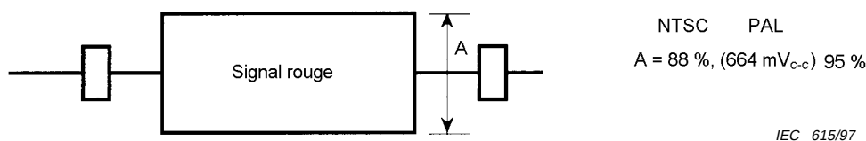
Figure 24 – Signal d'essai de chrominance de type S
