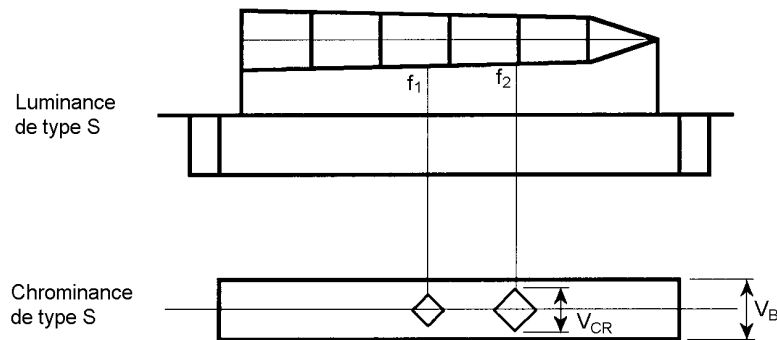
Figure 47 – Mesures du niveau des signaux
