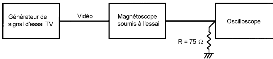
Figure 39 – Synoptique pour les mesures
