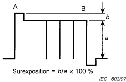
Figure 10 – Forme d'onde pour un rebondissement
