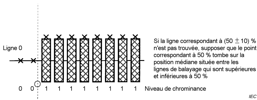
Figure 33 – Forme d'onde du signal de chrominance de type S sur la ligne 0 (exemple de mesure n° 1)
