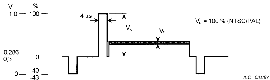
Figure 40 – Mesures pour le niveau des signaux
