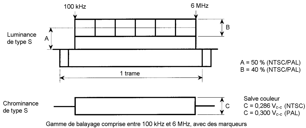
Figure 45 – Signal d'essai de rampe de fréquence vidéo
