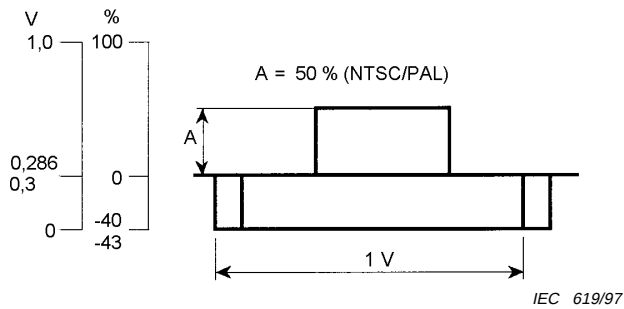
Figure 28 – Signal d'essai de fenêtre de luminance de type S
