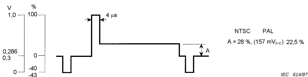
Figure 23 – Signal d'essai de luminance de type S
