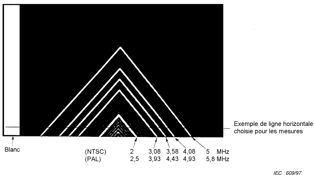
Figure 18 – Signal d'essai sur un moniteur de télévision
