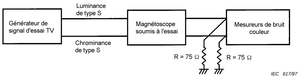
Figure 26 – Synoptique pour une entrée vidéo de type S
