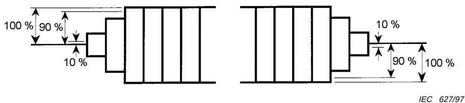
Figure 36 – Mesures du niveau du signal de chrominance
