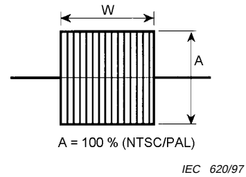
Figure 29 – Signal d'essai de fenêtre de chrominance de type S
