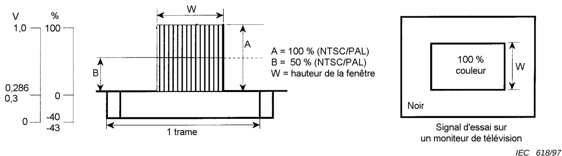
Figure 27 – Signal d'essai de fenêtre couleur composite
