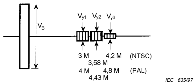
Figure 44 – Mesures du niveau des signaux
