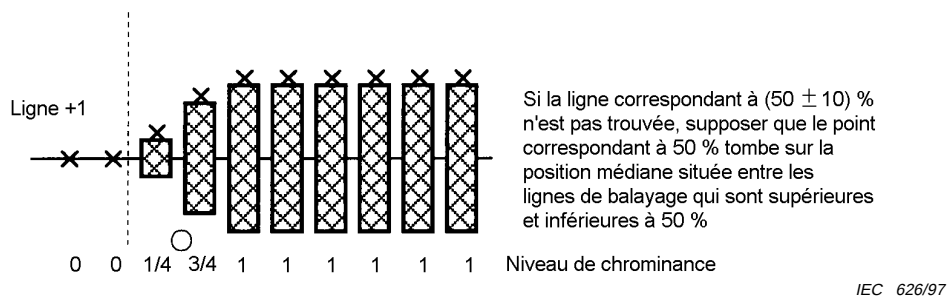
Figure 34 – Forme d'onde du signal de chrominance de type S sur la ligne +1/2 (exemple de mesure n° 2)
