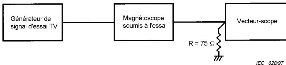
Figure 37 – Synoptique pour les mesures
