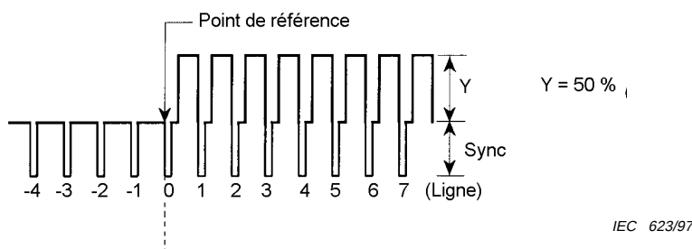
Figure 32 – Forme d'onde du signal de luminance de type S
