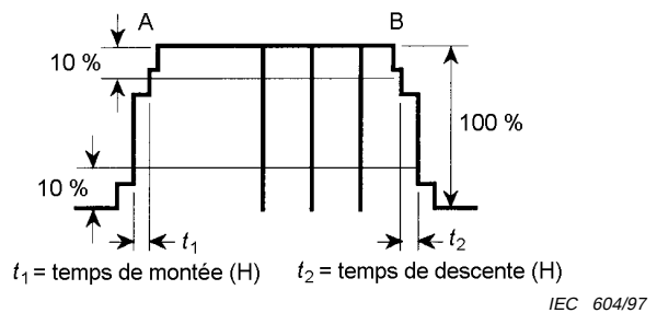
Figure 13 – Forme d'onde du temps de montée et de descente
