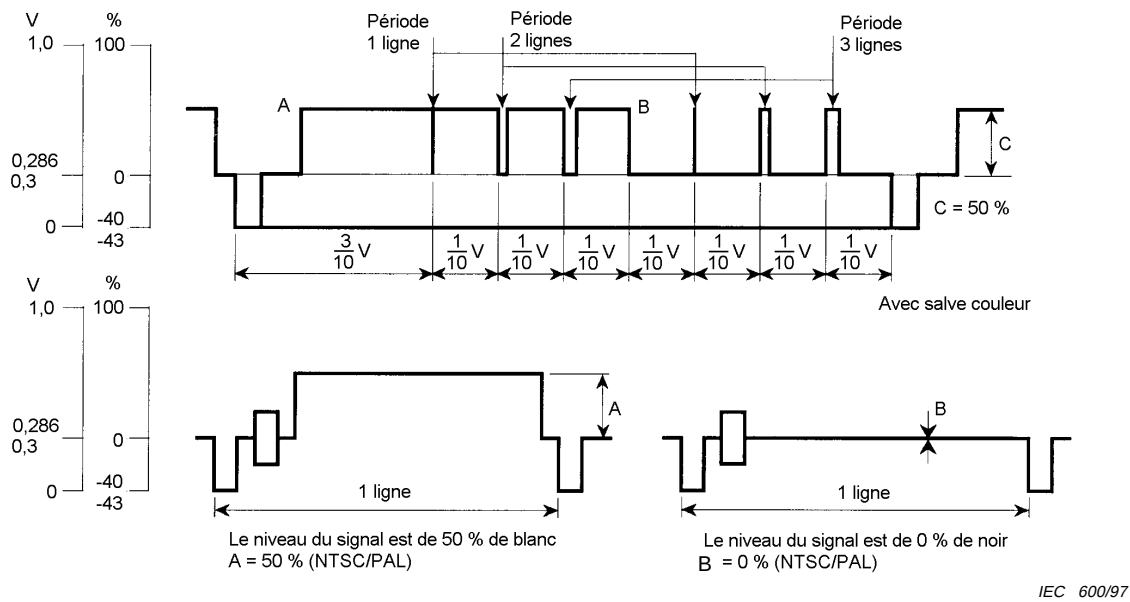
Figure 9 – Signal d'essai vidéo composite
