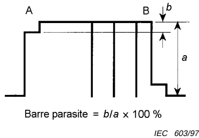
Figure 12 – Forme d'onde de barre parasite
