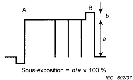
Figure 11 – Forme d'onde pour une suroscillation
