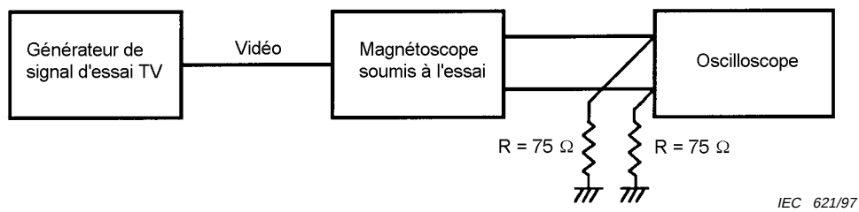
Figure 30 – Synoptique pour un signal d'entrée vidéo composite
