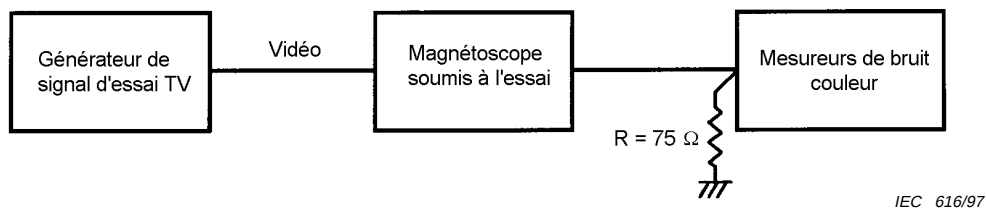
Figure 25 – Synoptique pour une entrée vidéo composite
