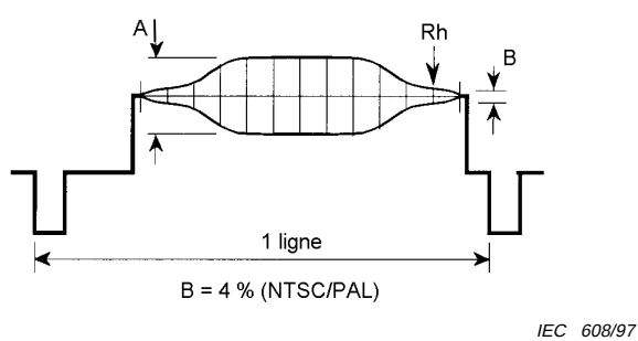
Figure 17 – Forme d'onde pour un signal d'entrée de type S
