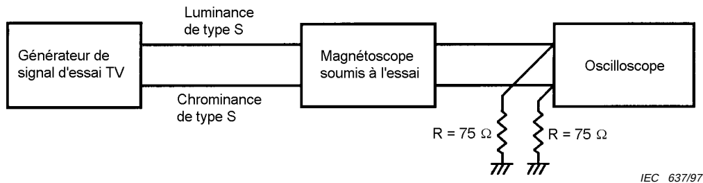
Figure 46 – Synoptique pour les mesures
