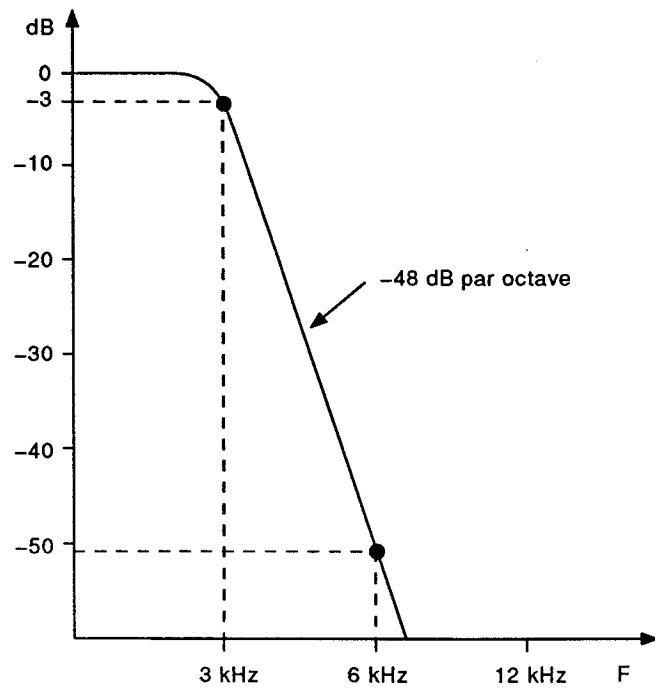
Figure 14 – Caractéristiques du filtre passe-bas
