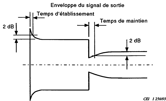
Figure 11b – Définition des temps d'établissement et de maintien (2.9.4)
