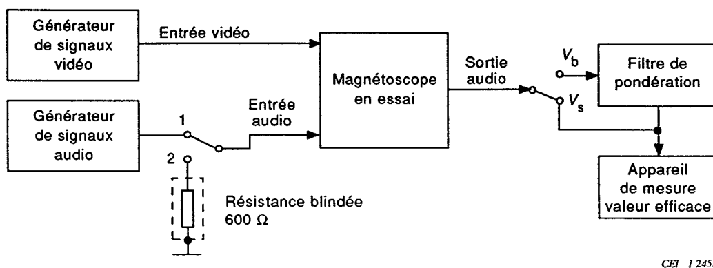
Figure 2 – Circuit de mesure: – Rapport signal sur bruit (2.2) CAG hors service – Dynamique (2.4)
