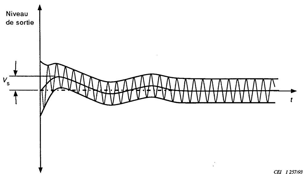
Figure 12 – Transition en sortie lors du signal établissement
