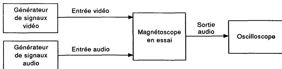
Figure 9 – Circuit de mesure – Fonctionnement du CAG (2.9) – Temps de maintien (2.9)
