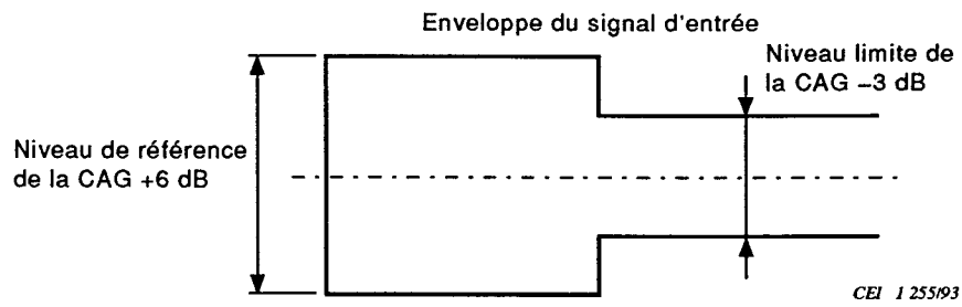
Figure 11a – Signal d'essai pour la mesure du temps d'établissement et de maintien (2.9.4)
