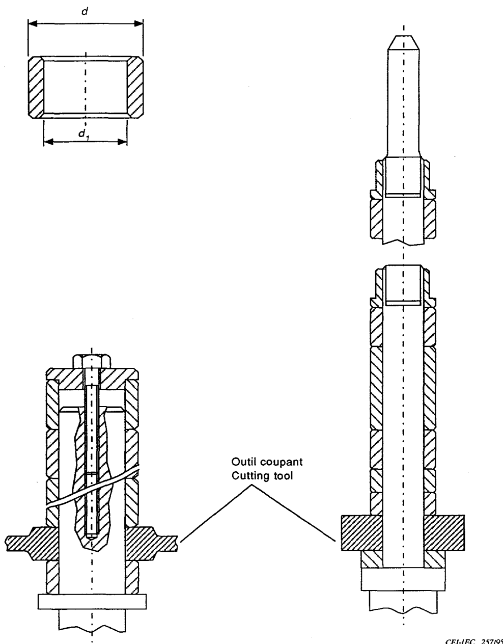
Figure 102 – Arbre porte-outil et bagues de serrage Tool holder spindles and spindle ring
