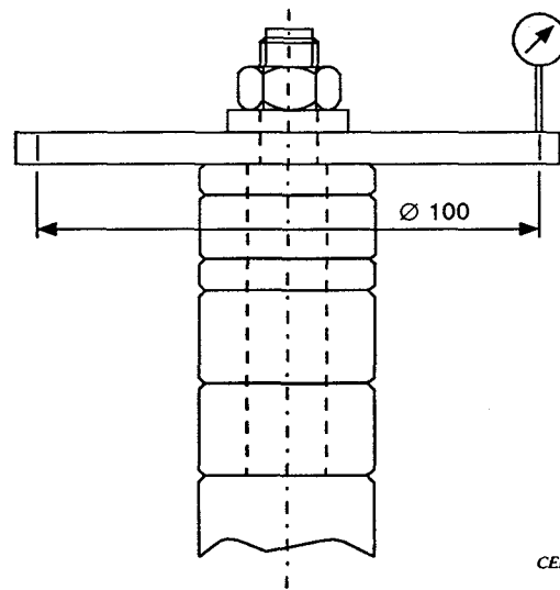
Figure 103 – Essai de battement latéral des bagues de serrage Run out test of spindle rings
