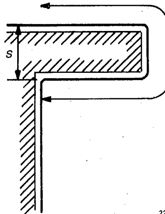
FIG. 1. - Boucle d'un conducteur de descente (voir paragraphe 2.2.4).
