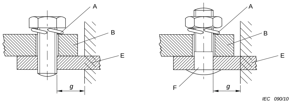
Figure IC.3 – Exemples de bornes à plaques
