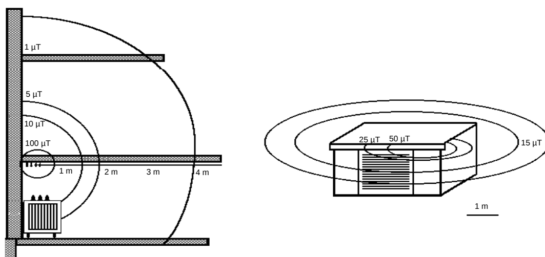
Figure 10 – Distribution du champ magnétique correspondant à un poste équipé d'un transformateur MT/BT de 315 kVA
