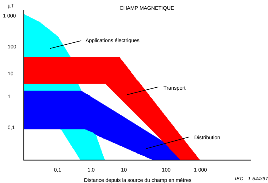
Figure 15 – Contributions représentatives des niveaux de champ magnétique – réseaux de distribution
