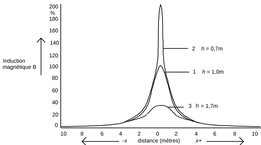
Figure 9 – Comparaison des valeurs d'induction magnétique des câbles à un seul conducteur posés à des profondeurs de 0,7 m (courbe 2), 1,7 m (courbe 3), avec un câble posé à une profondeur de 1 m (courbe 1).
