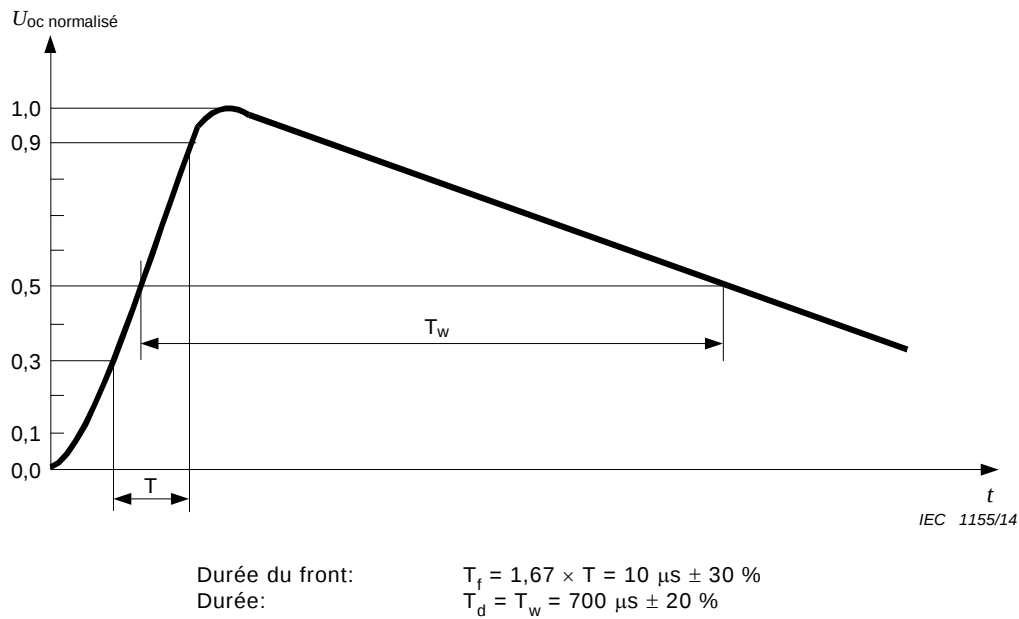
Figure A.2 – Forme d’onde de tension en circuit ouvert (10/700 μs)
