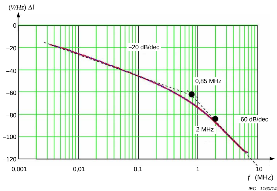
Figure E.3 – Tension de choc (1,2/50 \mu\text{s} ): réponse spectrale, \Delta f = 3,333 \text{ kHz}
