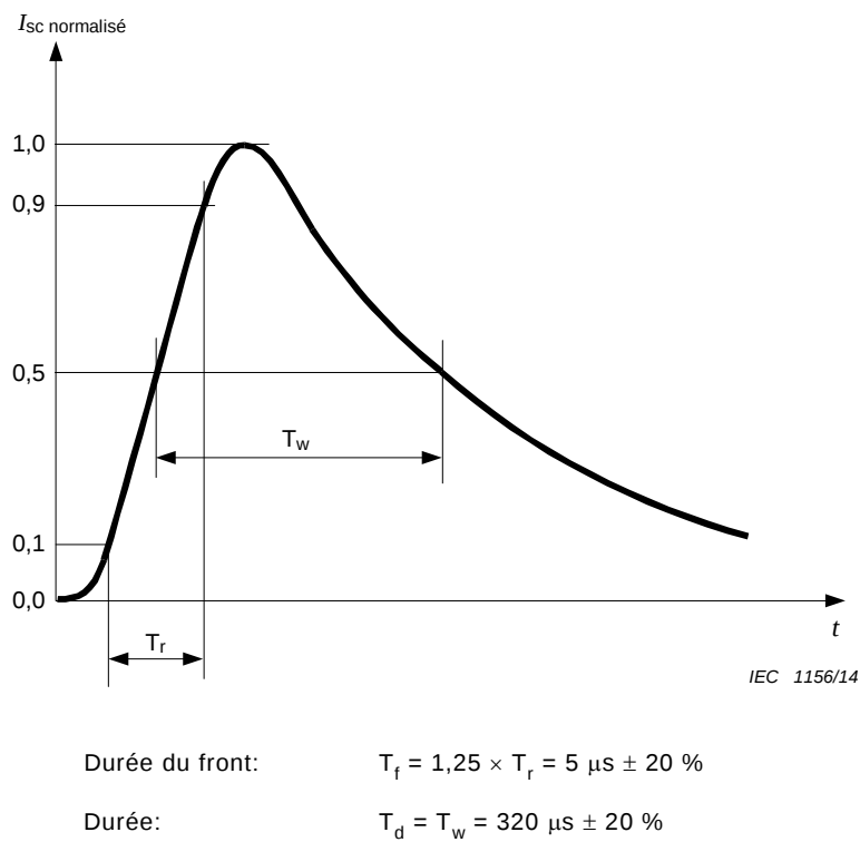
Figure A.3 – Forme d’onde de courant de court-circuit 5/320 μs
