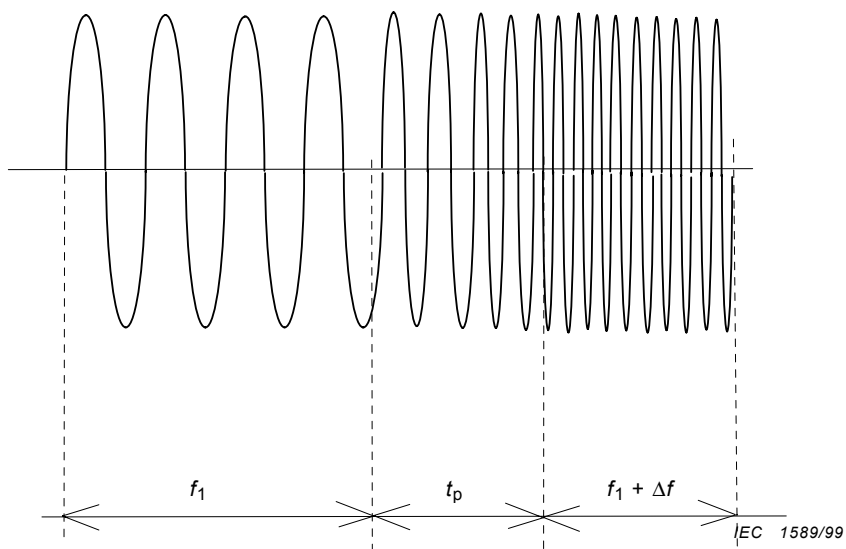
Figure 2 – Exemple de durée transitoire t_p
