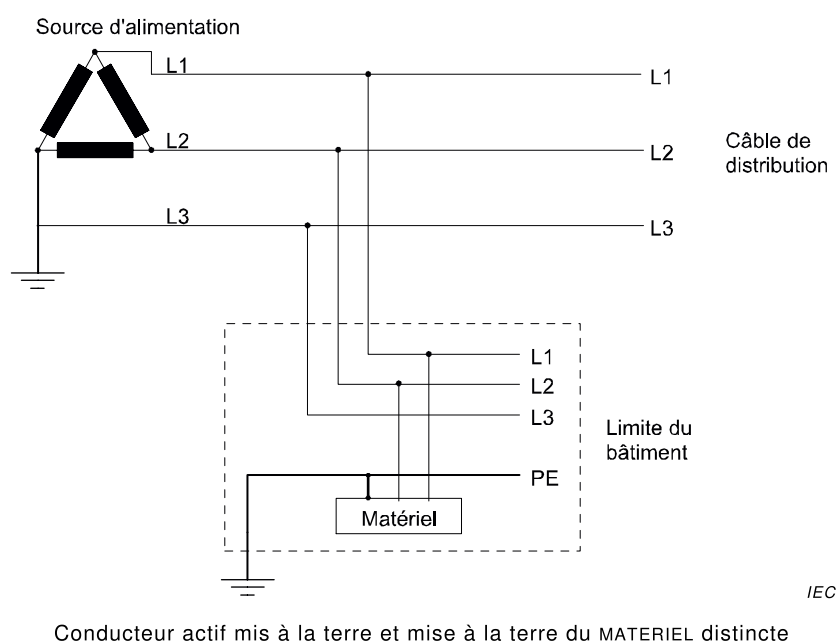
Figure I.6 – Exemple de schéma TT à 3 conducteurs actifs
