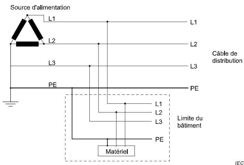
Conducteur actif mis à la terre
