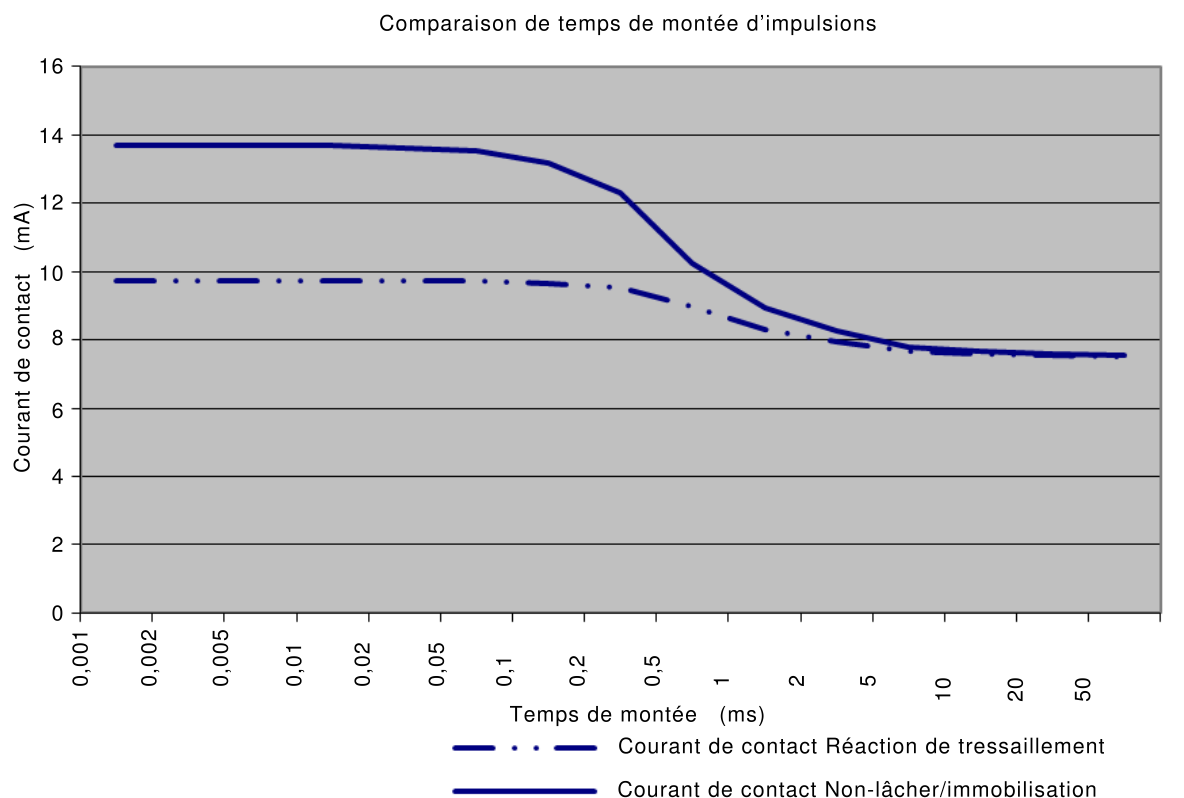
Figure H.5 – Diagramme du courant de contact en fonction du temps de montée, onde carrée de 20 ms
