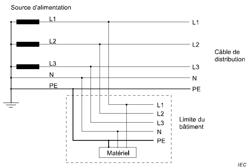
Conducteur neutre et conducteur de protection distincts
