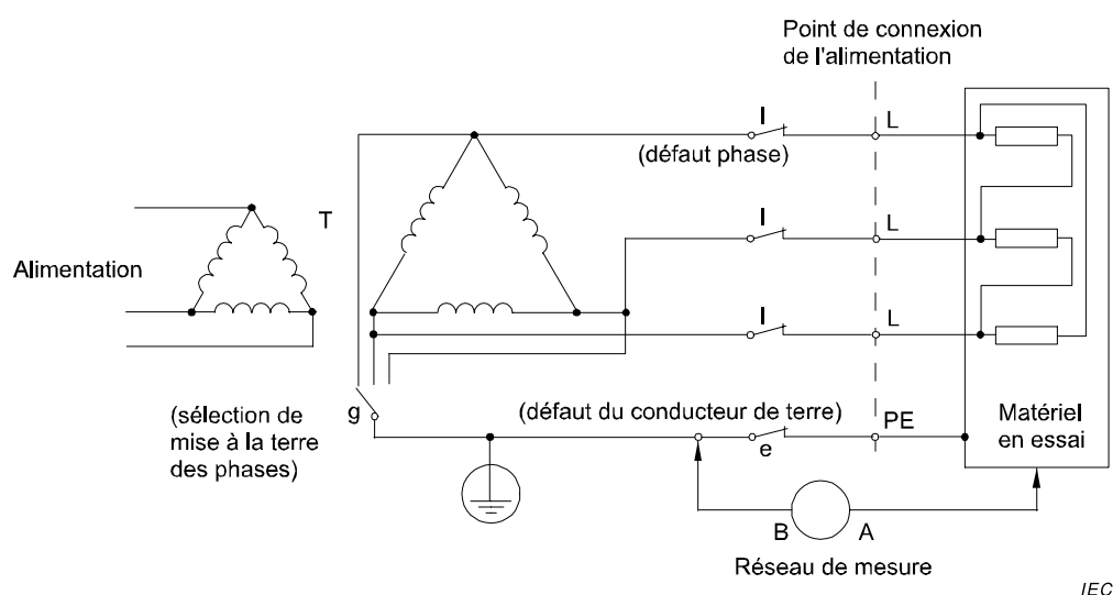
Figure 13 – Schéma triangle non mis à la terre
