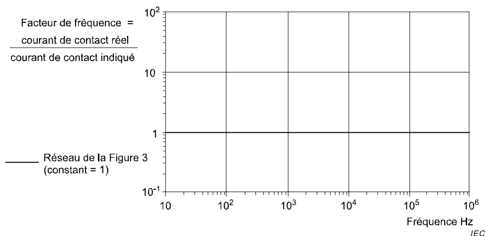
Figure F.1 – Facteur de fréquence pour les brûlures électriques
