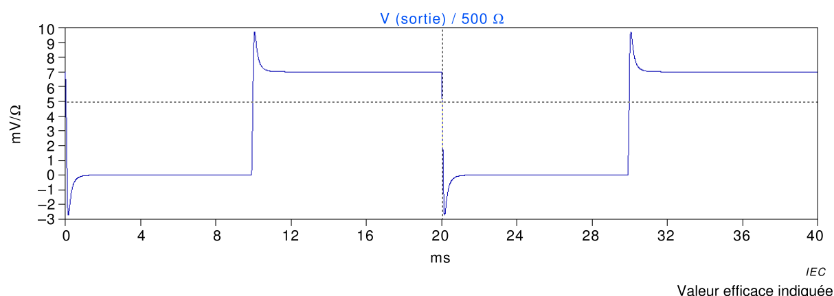
Figure H.8 – Onde carrée 50 Hz, temps de montée 0,1 ms, non-lâcher/immobilisation
