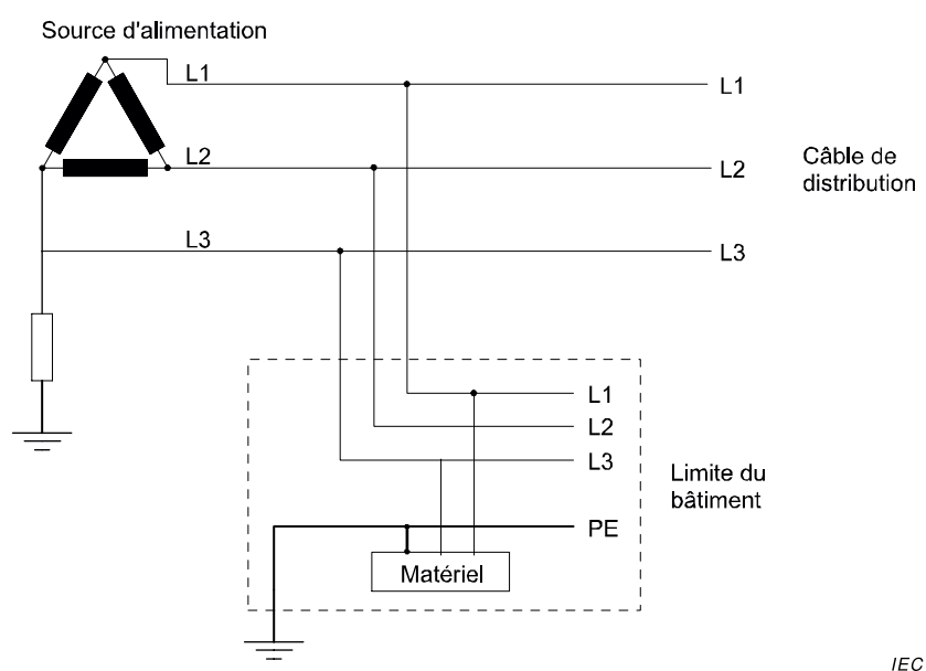
Figure I.8 – Exemple de schéma IT à 3 conducteurs actifs
