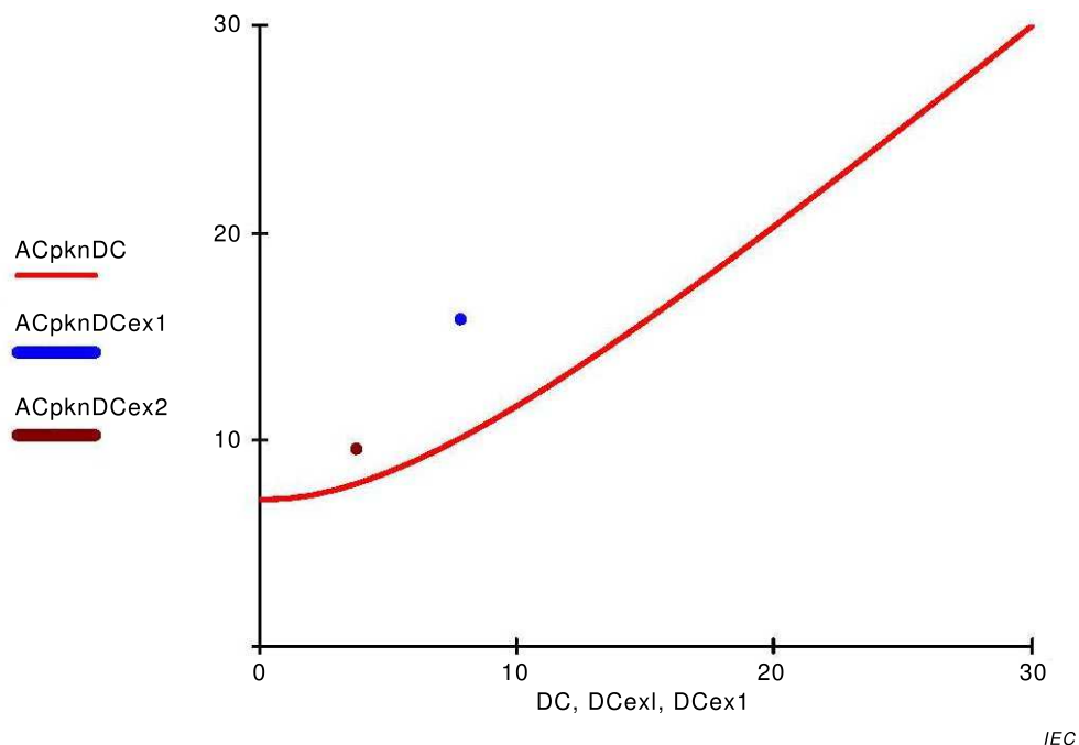
Figure H.9 – Seuil de non-lâcher de l'IEC TS 60479-2 pour des combinaisons de courant alternatif et de courant continu augmenté de données supplémentaires, en mA pour chaque axe
