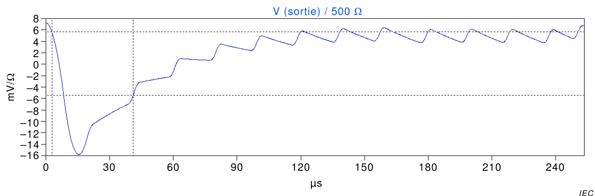
Figure H.10 – Cas ex1: fenêtre de valeurs efficaces
