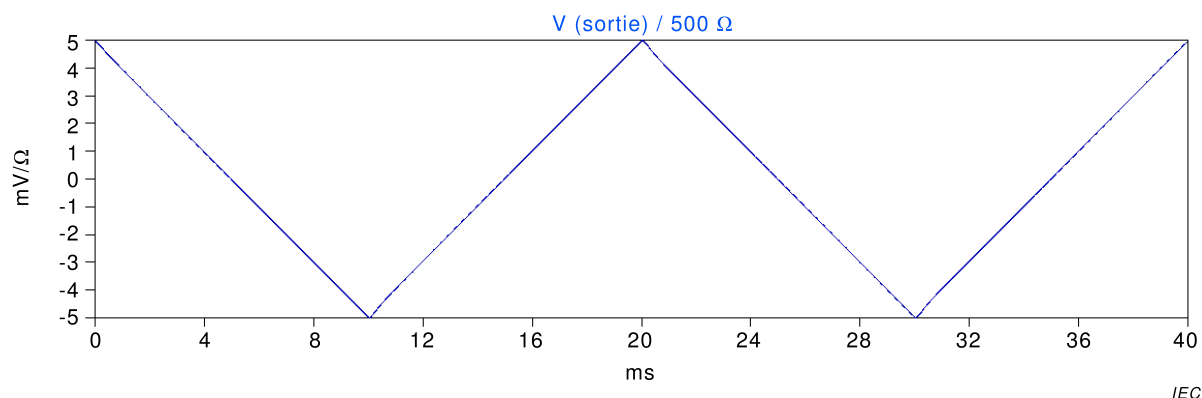
Figure H.1 – Forme d'onde triangulaire de courant de contact, réaction de tressaillement
