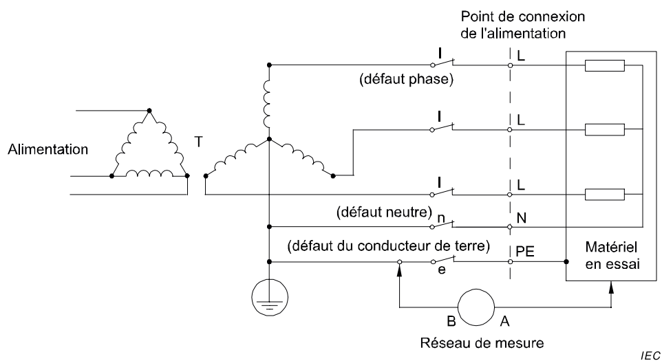
Figure 11 – Matériel triphasé dans un schéma étoile TN ou TT
