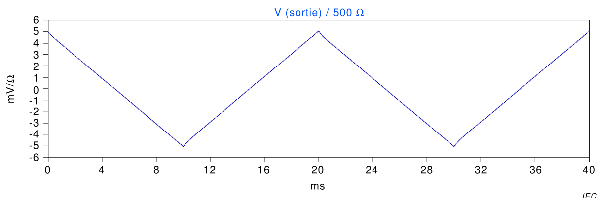
Figure H.2 – Forme d'onde triangulaire de courant de contact, non-lâcher/immobilisation
