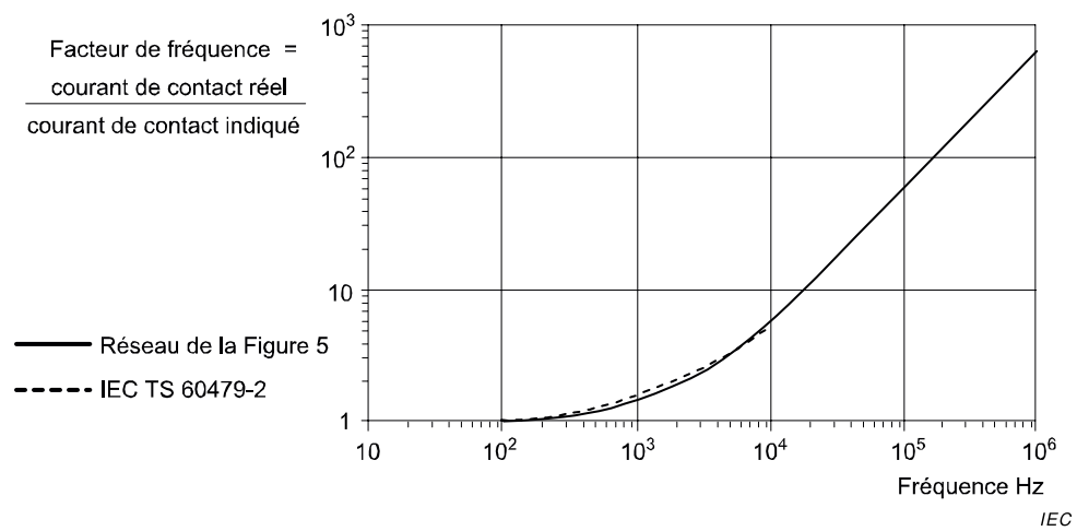
Figure F.3 – Facteur de fréquence pour le non-lâcher/l'immobilisation
