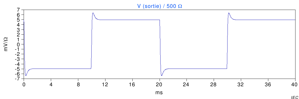
Figure H.3 – Réponse impulsionnelle avec temps de montée de 1 ms, réaction de tressaillement
