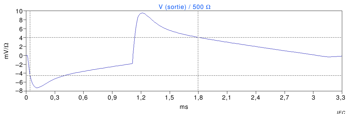
Figure H.11 – Cas ex2 de forme d'onde: fenêtre de valeurs efficaces
