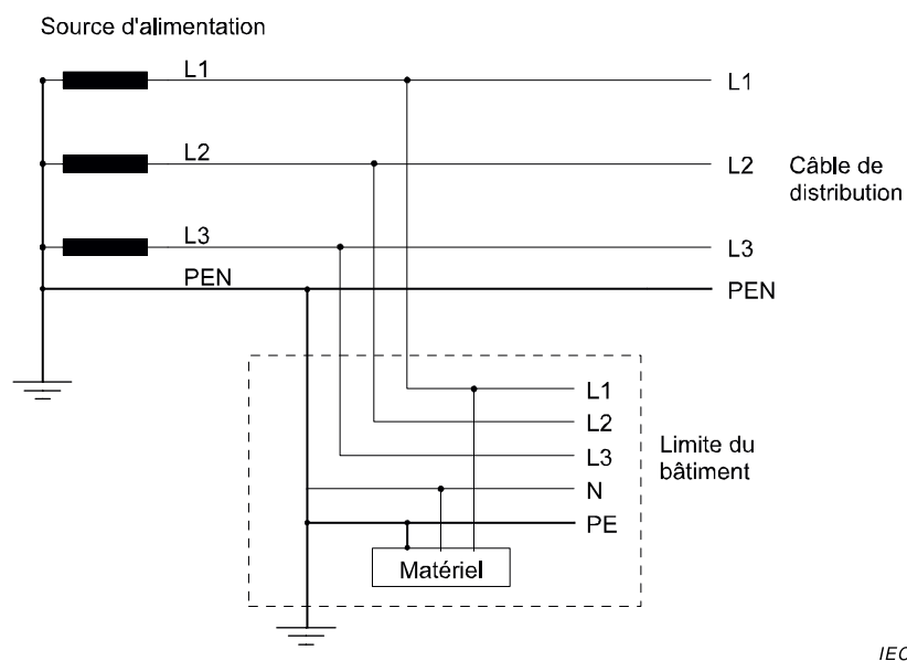
Figure I.2 – Exemple de schéma TN-C-S
