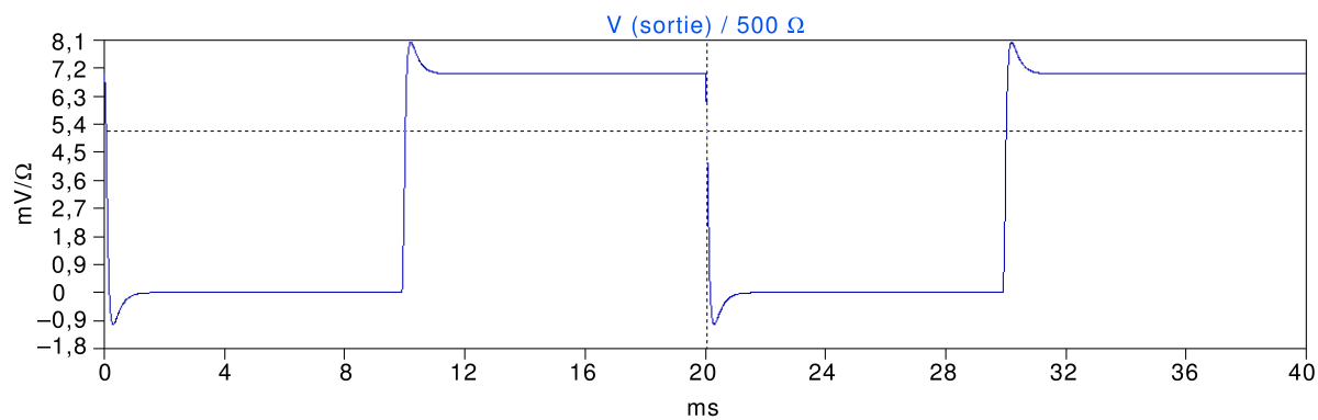
Figure H.7 – Onde carrée 50 Hz, temps de montée 0,1 ms, réaction de tressaillement
