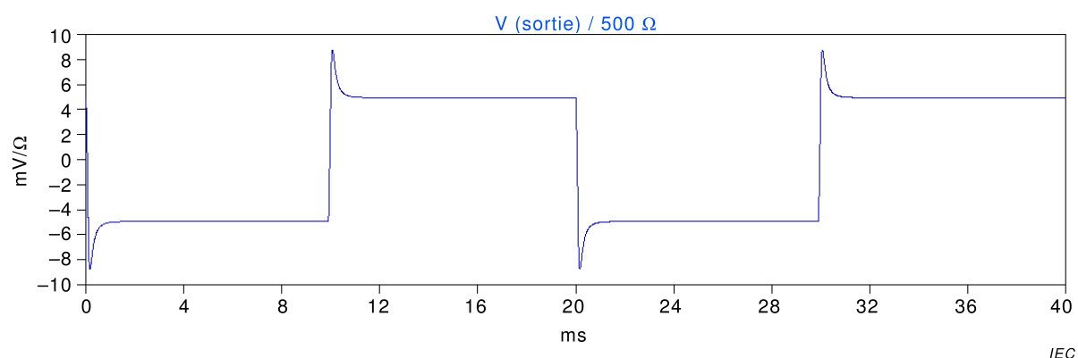
Figure H.4 – Réponse impulsionnelle avec temps de montée de 1 ms, non-lâcher/immobilisation
