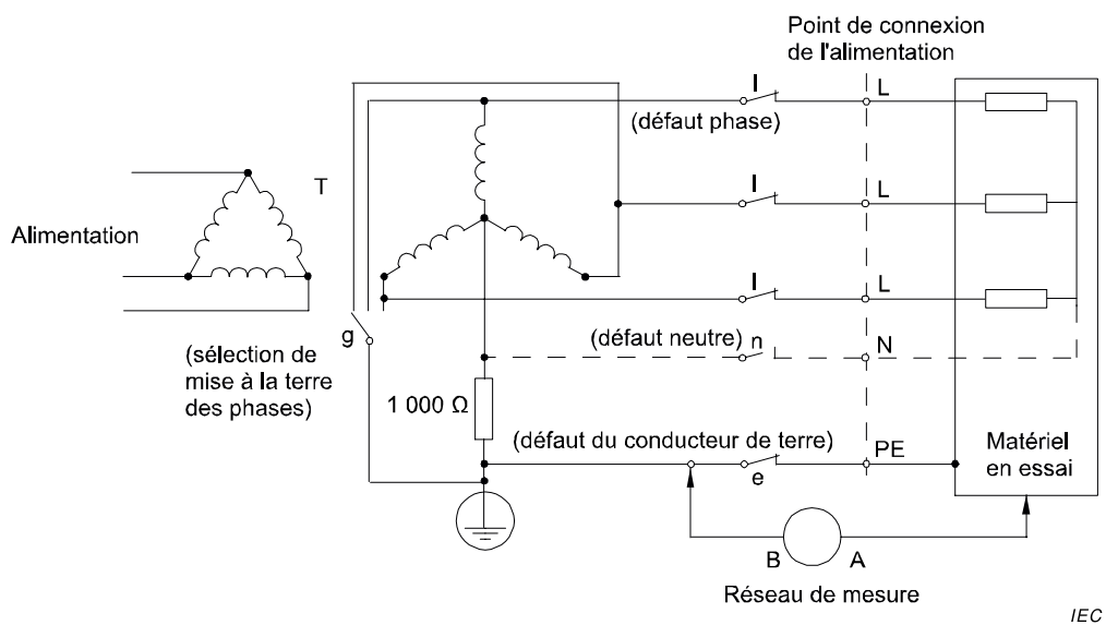
Figure 11 – Matériel triphasé dans un schéma étoile TN ou TT
