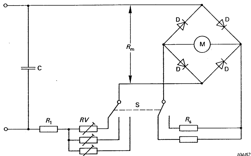
Figure C - Circuit de mesure des courants de fuite
