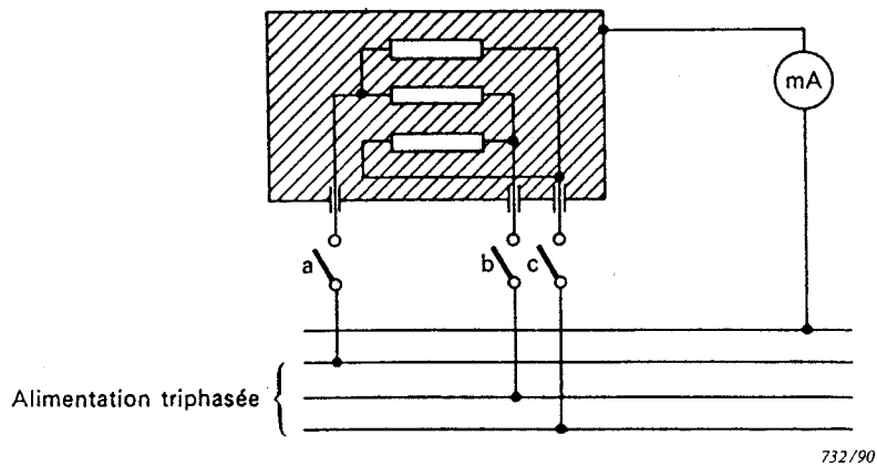
Figure B - Schéma pour la mesure du courant de fuite à la température de régime pour connexion triphasée des appareils autres que ceux de la classe II.
