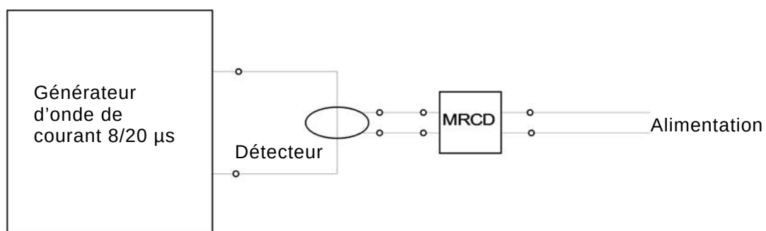
Figure M.6a) MRCD à dispositif de détection séparé
