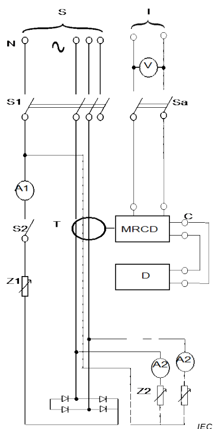
Figure M.15a) – MRCD avec un dispositif de détection séparé
