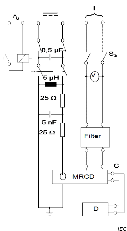
Figure M.5b) – MRCD avec un dispositif de détection intégré
