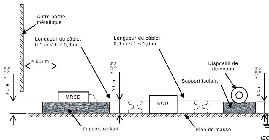
Figure M.21 – Vérification de l'immunité aux transitoires électriques rapides en sèves (TER/S) sur le raccordement du dispositif de détection d'un MRCD à dispositif de détection séparé (complémentaire à l'essai de l'Annexe B)
