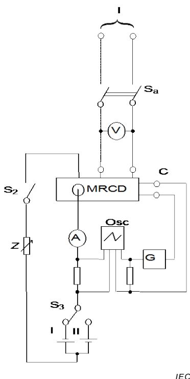
Figure M.12b) – MRCD avec un dispositif de détection intégré
