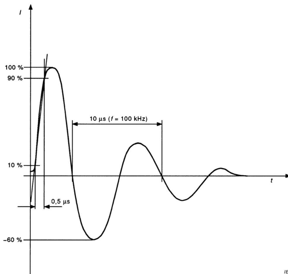
Figure B.4 – Onde de courant 0,5 μs/100 kHz
