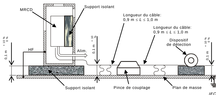
Figure M.21 – Vérification de l'immunité aux transitoires électriques rapides en sèves (TER/S) sur le raccordement du dispositif de détection d'un MRCD à dispositif de détection séparé (complémentaire à l'essai de l'Annexe B)
