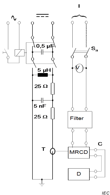
Figure M.5a) – MRCD avec un dispositif de détection séparé
