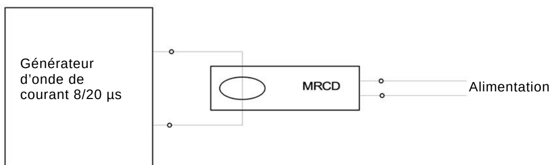
Figure M.6b) MRCD à dispositif de détection intégré
