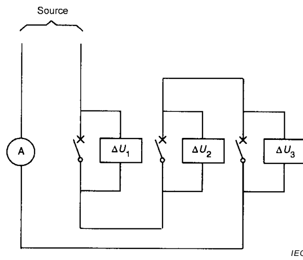
Figure G.2 – Exemple de mesure de la perte de puissance selon G.2.2 et G.2.3
