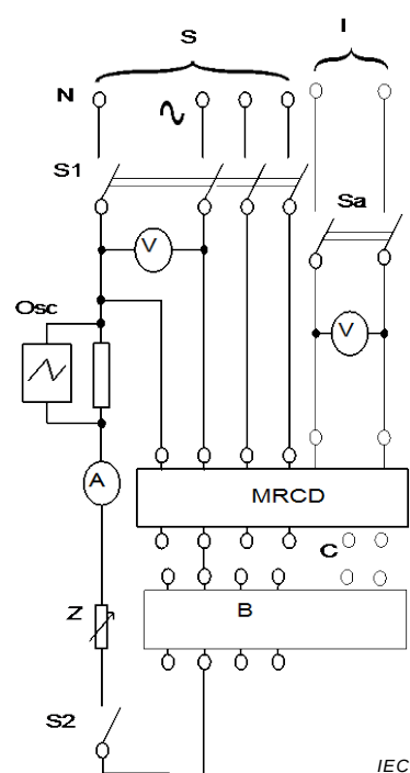
Figure M.2c) – MRCD de type à bornes
