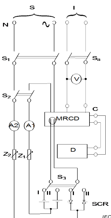
Figure M.10b) – MRCD avec un dispositif de détection intégré
