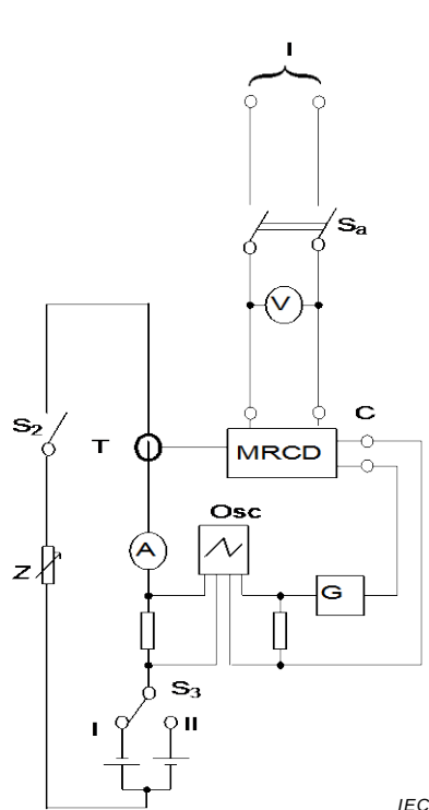
Figure M.12a) – MRCD avec un dispositif de détection séparé
