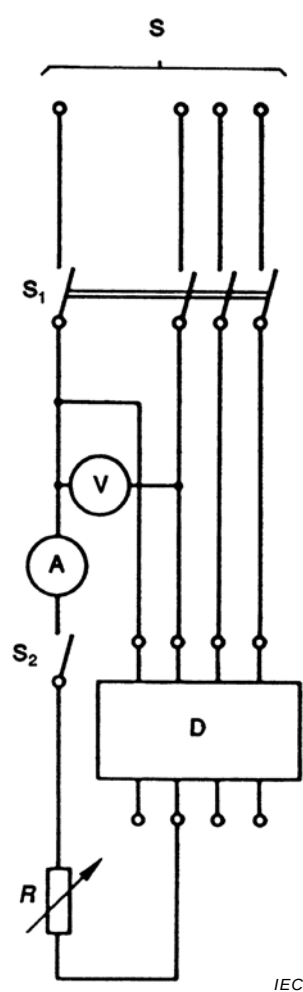
Figure B.1 – Circuit d'essai pour la vérification de la caractéristique de fonctionnement (voir B.8.2)
