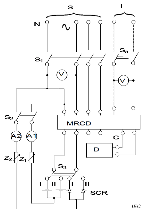
Figure M.10c) – MRCD de type à bornes
