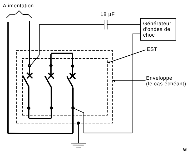
Figure F.13 – Circuit d'essai pour la vérification de l'influence des ondes de courant de choc sur le circuit principal selon F.4.5 – Trois pôles de phase en série
