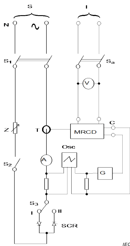
Figure M.8a) – MRCD avec un dispositif de détection séparé
