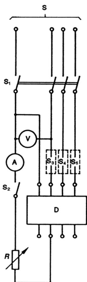
Figure B.3 – Circuit d’essai pour la vérification du comportement des DPR classés selon B.3.1.2.2 (voir B.8.9)
