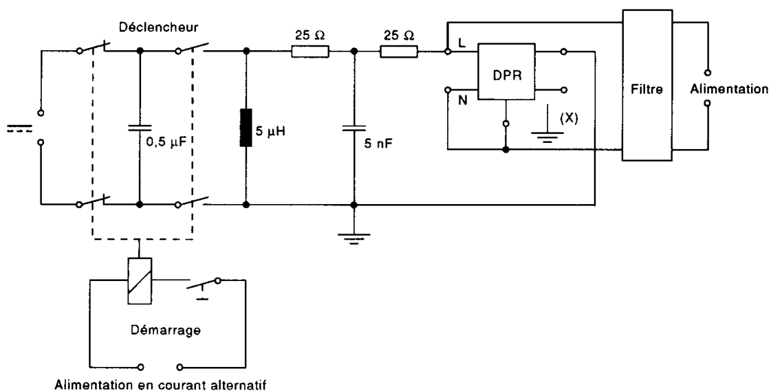
Figure B.4 – Onde de courant 0,5 μs/100 kHz
