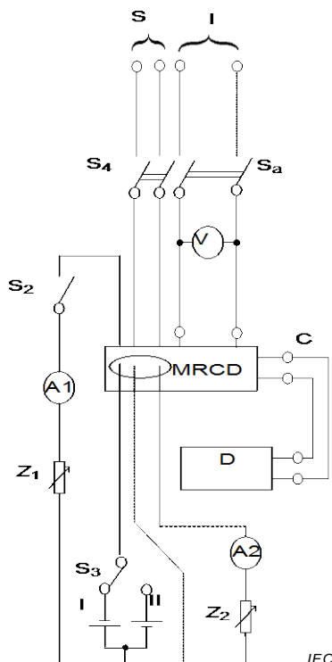
Figure M.11b) – MRCD avec un dispositif de détection intégré
