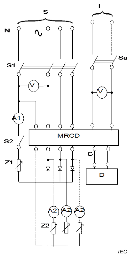
Figure M.14c) – MRCD de type à bornes
