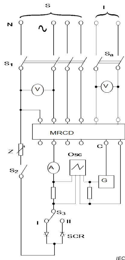
Figure M.8c) – MRCD de type à bornes
