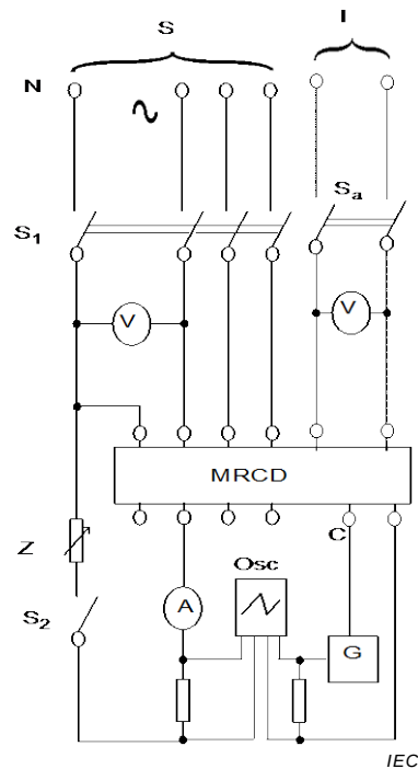
Figure M.3c) – MRCD de type à bornes
