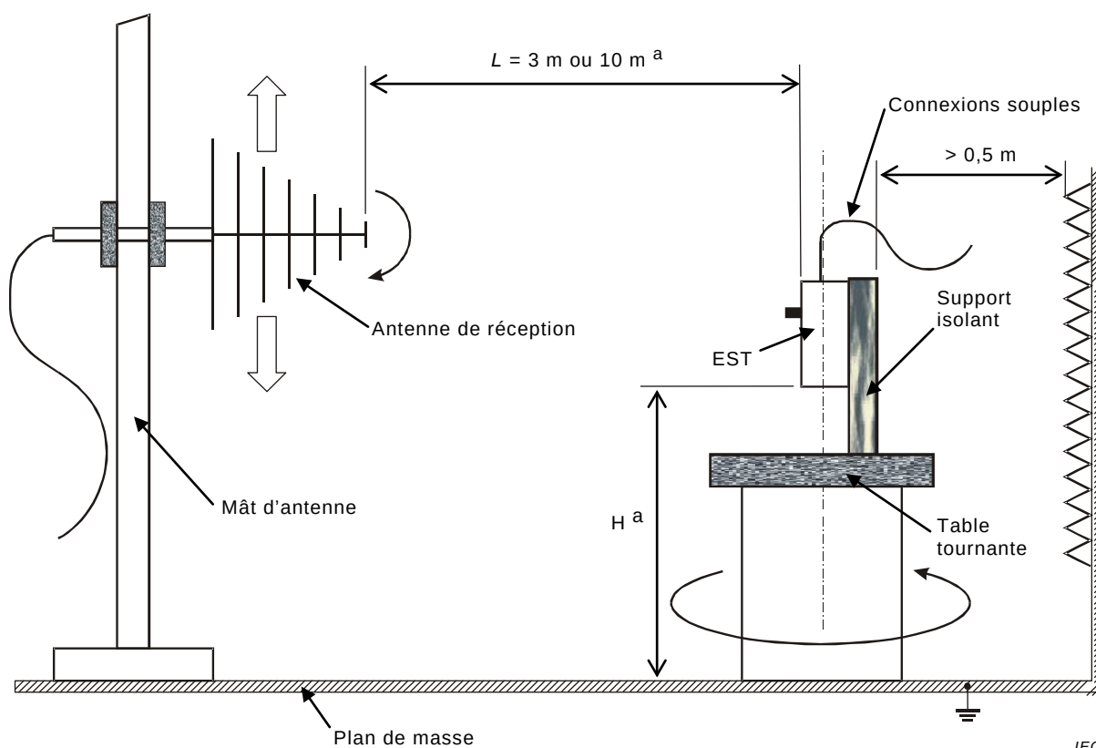
Figure J.2 – Installation d'essai pour le mesurage des émissions rayonnées aux fréquences radioélectriques
