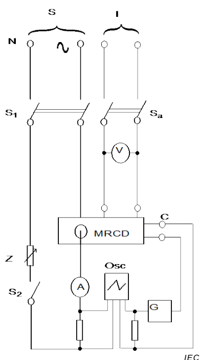
Figure M.3b) – MRCD avec un dispositif de détection intégré
