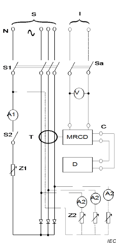
Figure M.14a) – MRCD avec un dispositif de détection séparé
