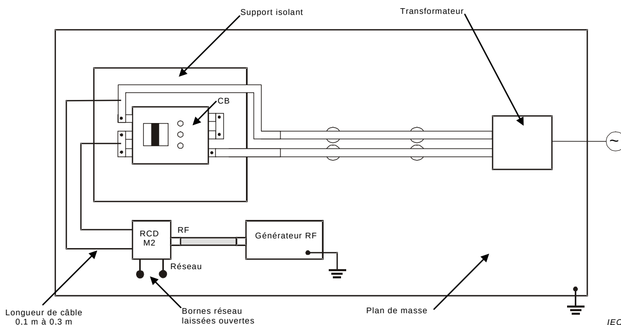
Figure F.21 – Disposition des raccordements pour la vérification de l'immunité aux perturbations conduites, induites par les champs radioélectriques – Configuration de deux pôles de phase en série
