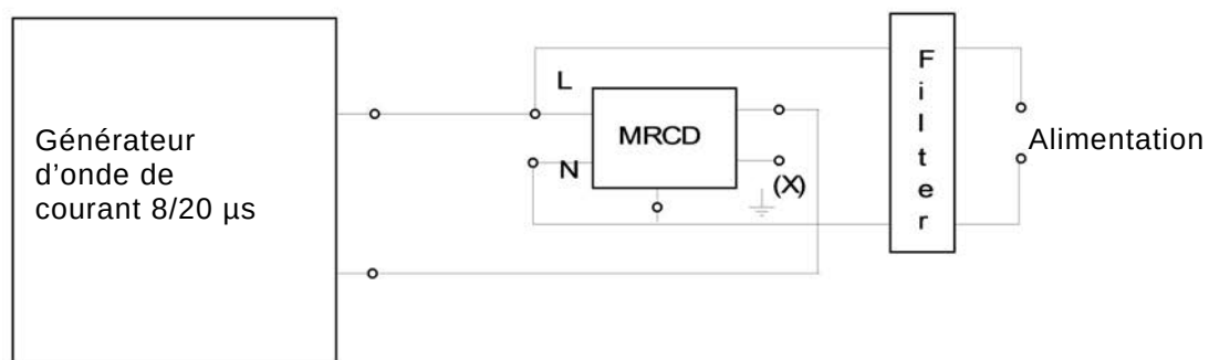
Figure M.6c) MRCD de type à bornes
