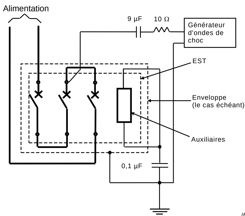
Figure F.10 – Circuit d'essai pour la vérification de l'influence des ondes de choc sur le circuit principal (phase-terre) selon F.4.5 – Trois pôles de phase en série
