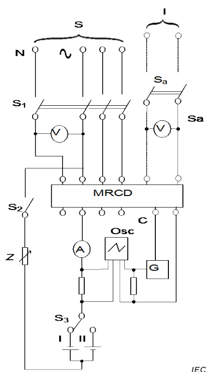
Figure M.12c) – MRCD de type à bornes
