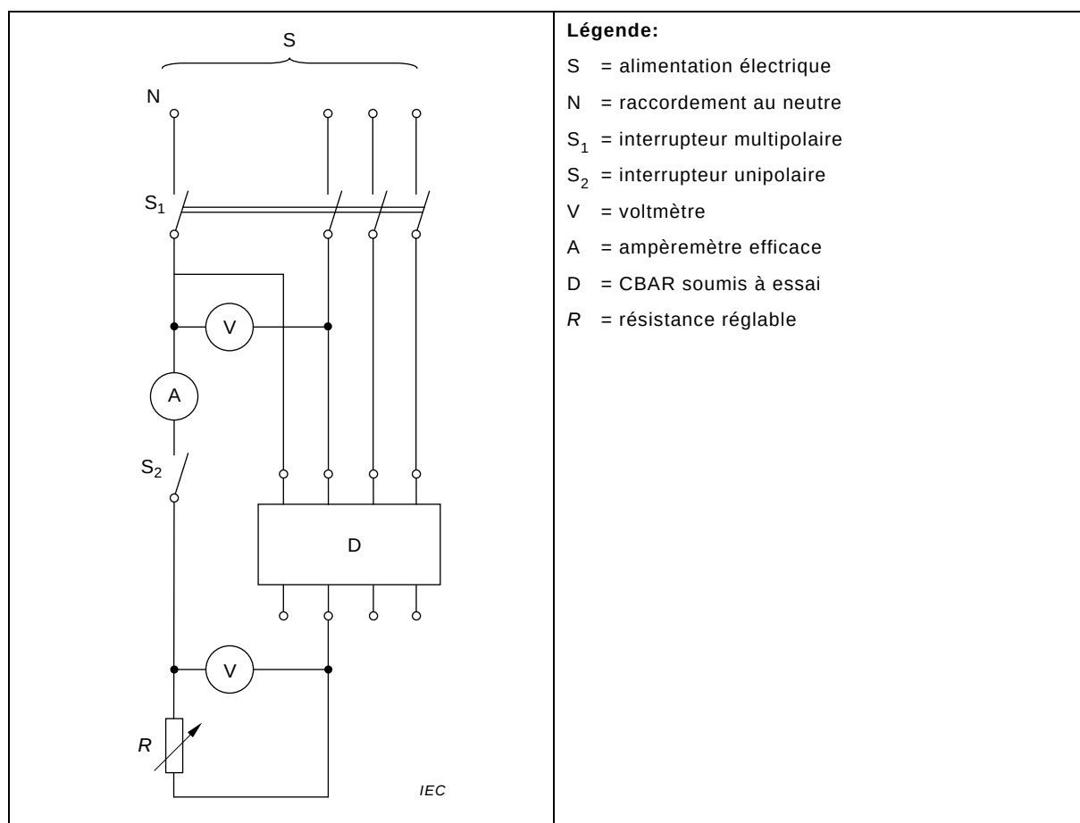
Figure R.1 – Circuit d’essai pour la vérification des fonctions de refermeture automatique
