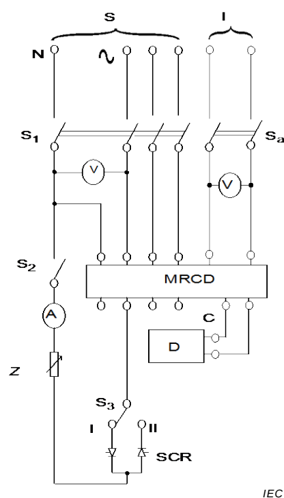
Figure M.7c) – MRCD de type à bornes
