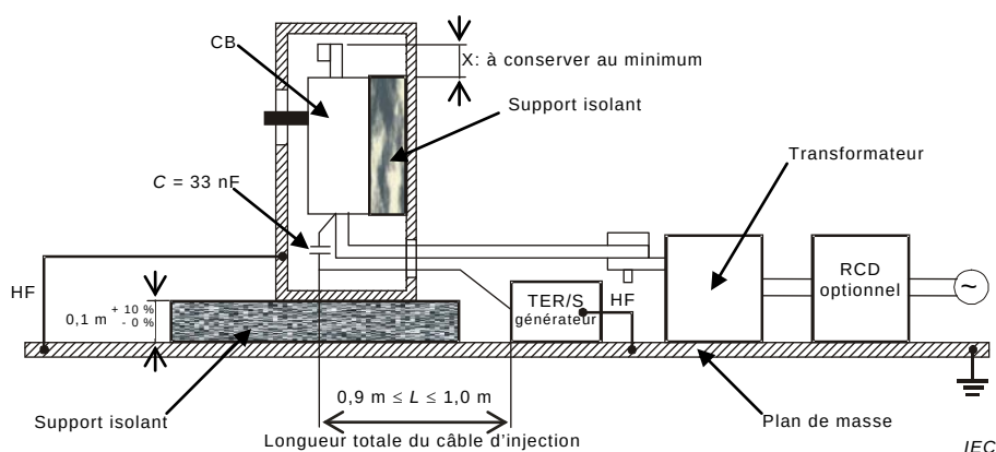
Figure F.17 – Installation d'essai pour la vérification de l'immunité aux champs électromagnétiques rayonnés aux fréquences radioélectriques
