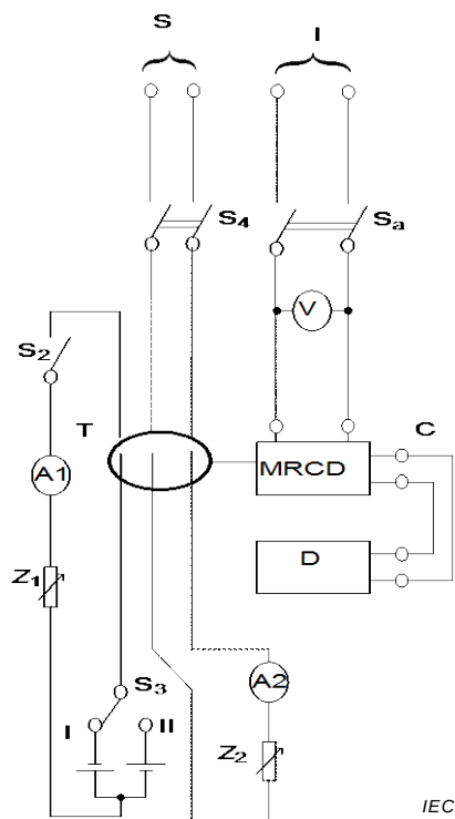
Figure M.11a) – MRCD avec un dispositif de détection séparé
