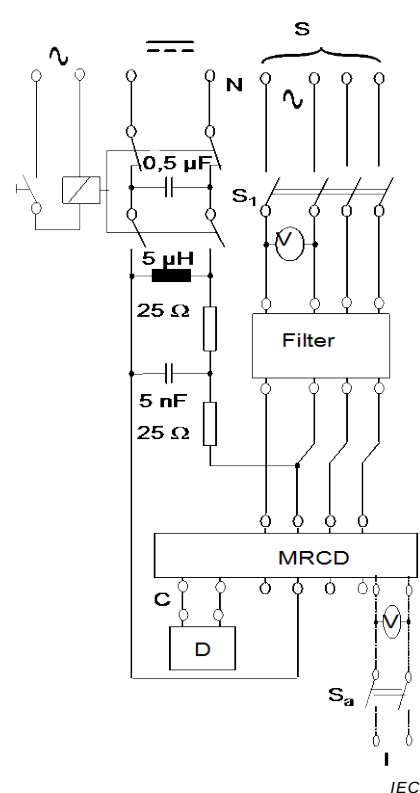
Figure M.5c) – MRCD de type à bornes
