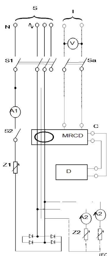
Figure M.15b) – MRCD avec un dispositif de détection intégré
