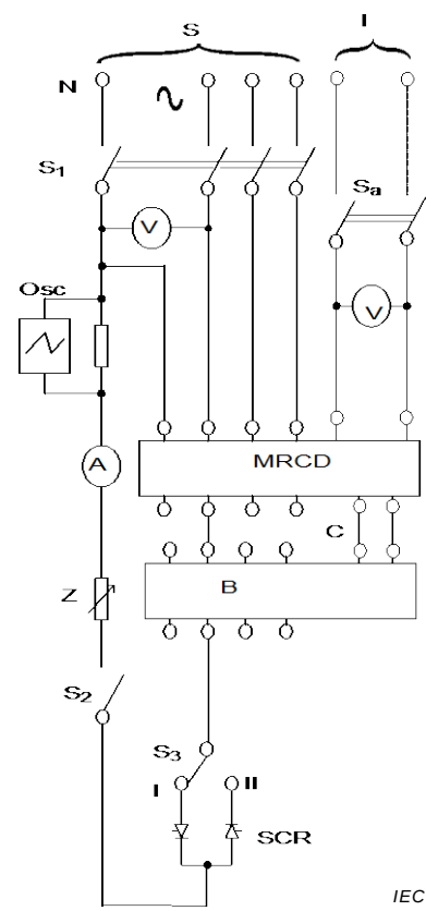
Figure M.9c) – MRCD de type à bornes
