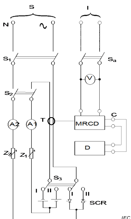
Figure M.10a) – MRCD avec un dispositif de détection séparé
