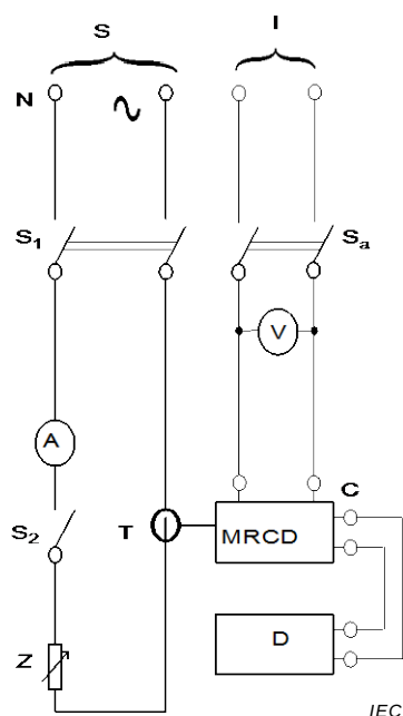
Figure M.1a) – MRCD avec un dispositif de détection séparé
