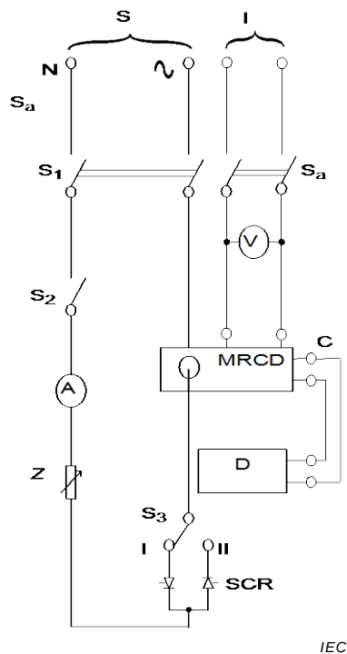
Figure M.7b) – MRCD avec un dispositif de détection intégré
