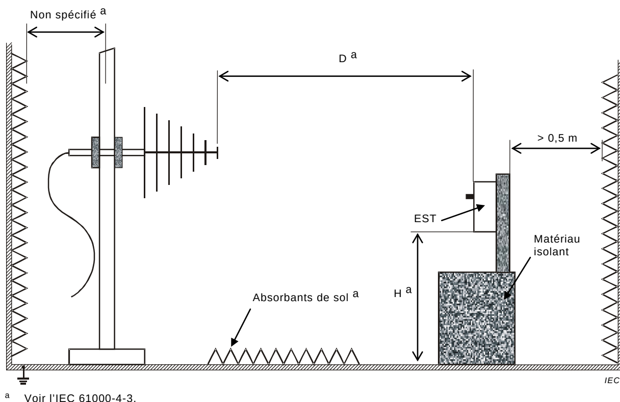
Figure J.4 – Installation d'essai pour la vérification de l'immunité aux champs électromagnétiques rayonnés aux fréquences radioélectriques
