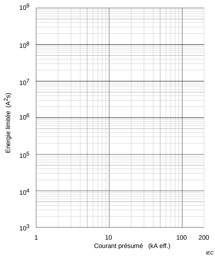
Figure K.4 – Modèle de caractéristiques de l'énergie limitée par rapport au courant présumé de 1 kA à 200 kA
