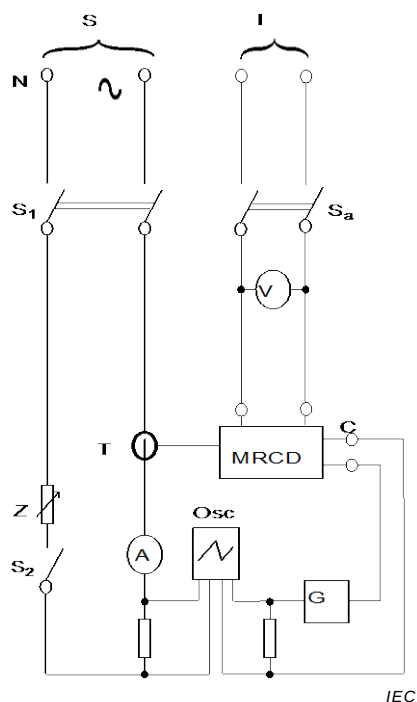
Figure M.3a) – MRCD avec un dispositif de détection séparé
