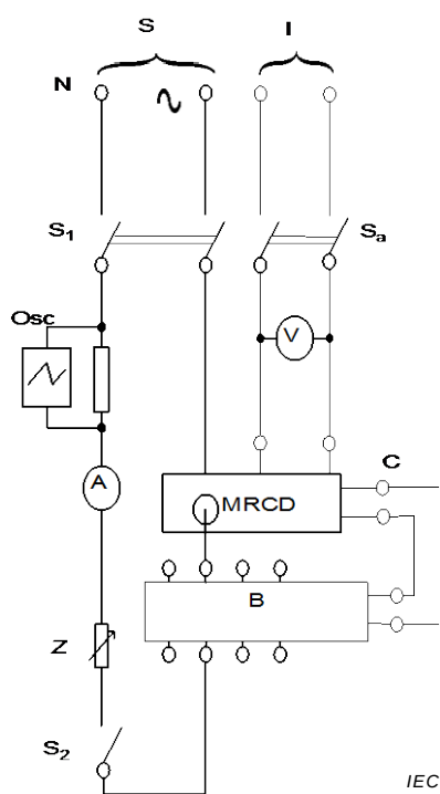
Figure M.2b) – MRCD avec un dispositif de détection intégré
