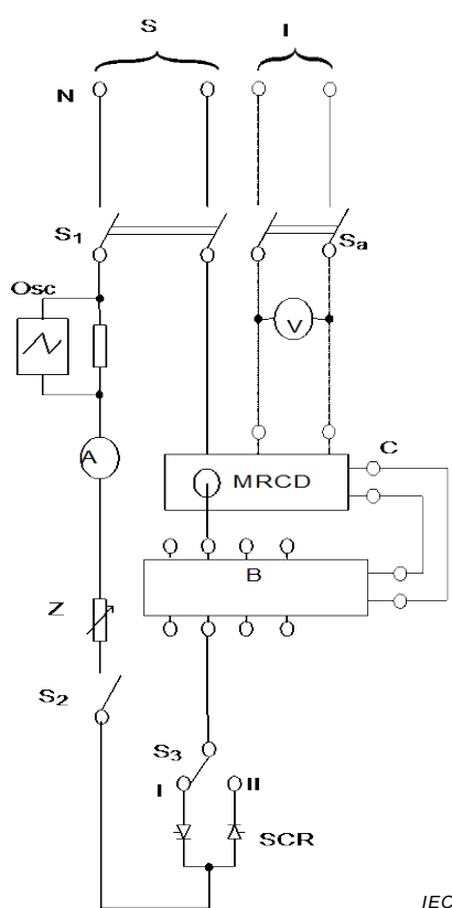
Figure M.9b) – MRCD avec un dispositif de détection intégré
