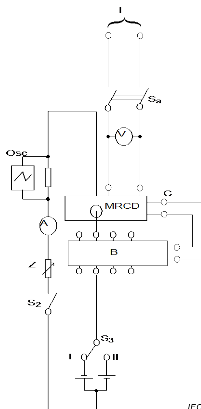
Figure M.13b) – MRCD avec un dispositif de détection intégré
