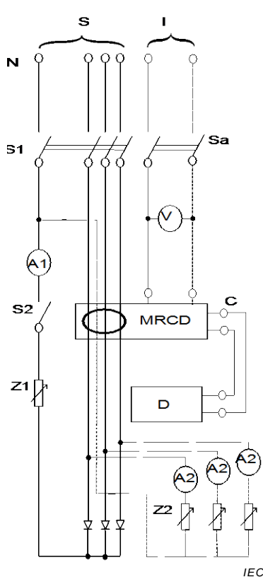
Figure M.14b) – MRCD avec un dispositif de détection intégré
