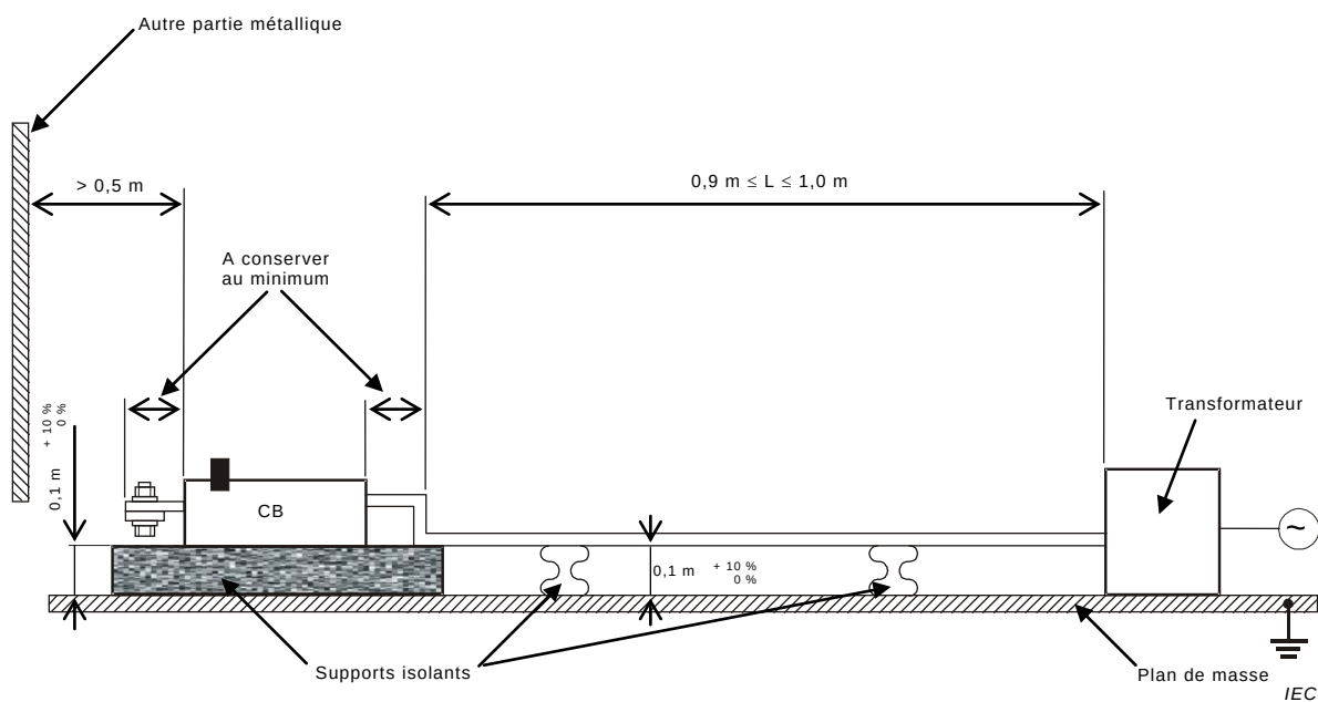
Figure F.19 – Installation d'essai pour la vérification de l'immunité aux transitoires électriques rapides en salves (TER/S) sur les lignes de signaux
