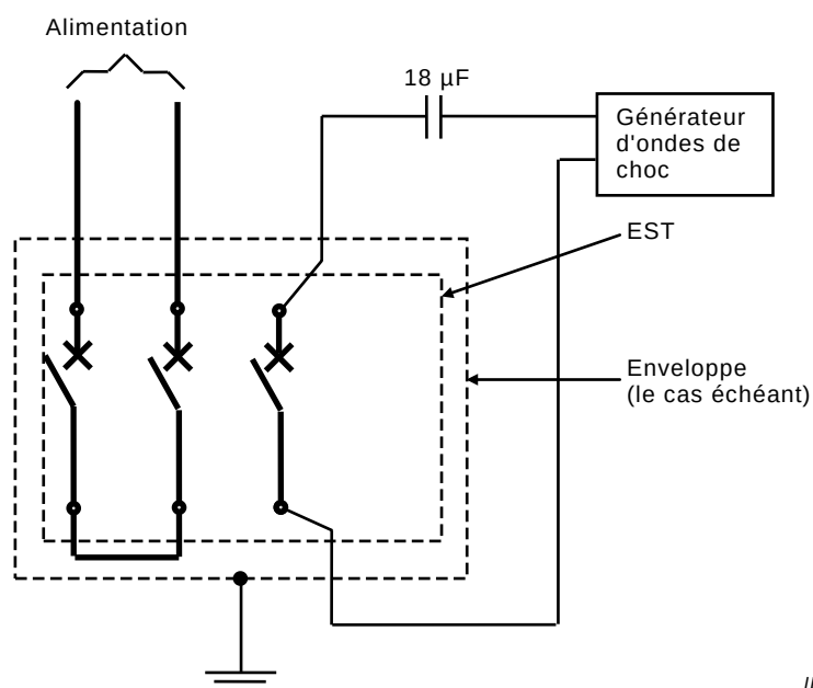
Figure F.12 – Circuit d'essai pour la vérification de l'influence des ondes de courant de choc sur le circuit principal selon F.4.5 – Deux pôles de phase en série
