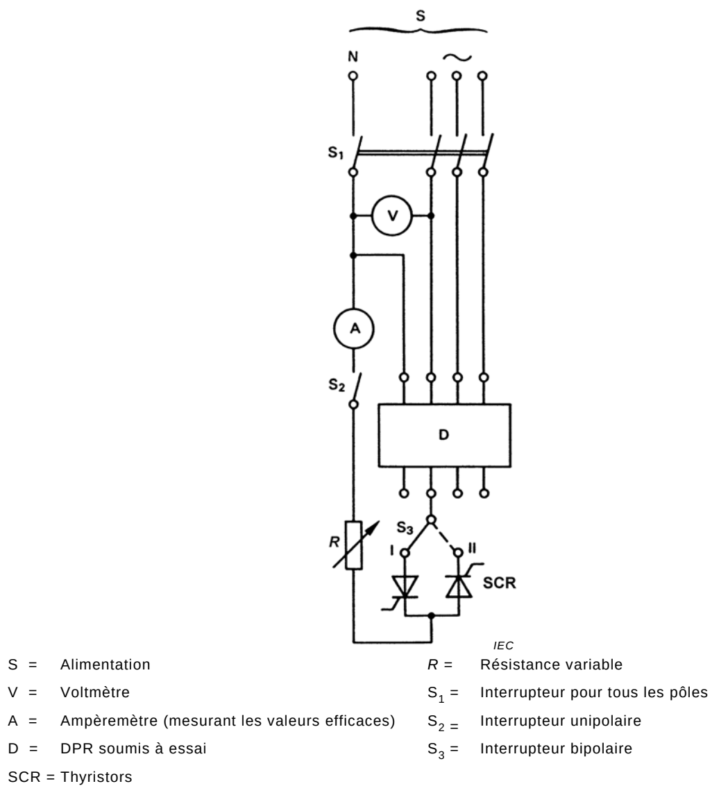
Figure B.8 – Circuit d'essai pour la vérification du fonctionnement correct des DPR, dans le cas de courants différentiels résiduels continus pulsés (voir B.8.7.2.1, B.8.7.2.2 et B.8.7.2.3)
