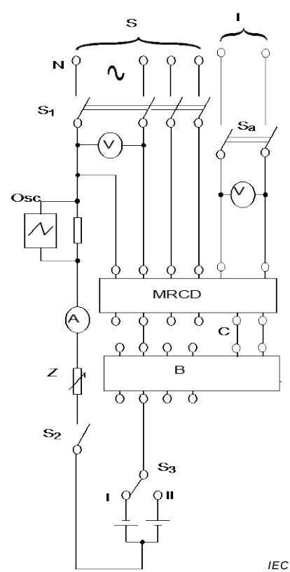
Figure M.13c) – MRCD de type à bornes
