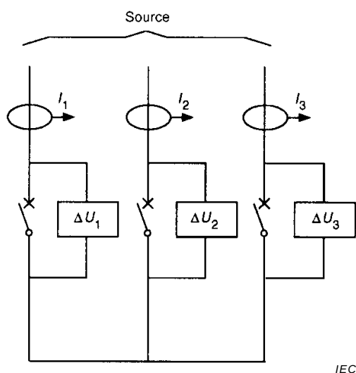
Figure G.1 – Exemple de mesure de la perte de puissance selon G.2.1
