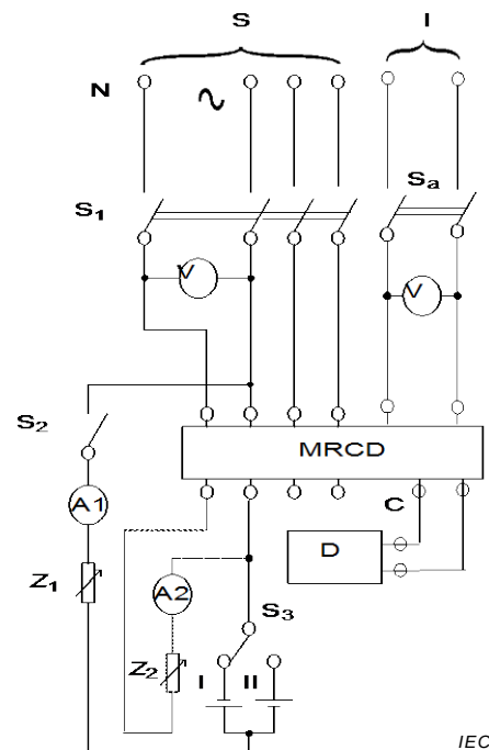
Figure M.11c) – MRCD de type à bornes
