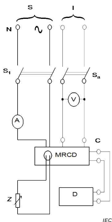
Figure M.4b) – MRCD avec un dispositif de détection intégré
