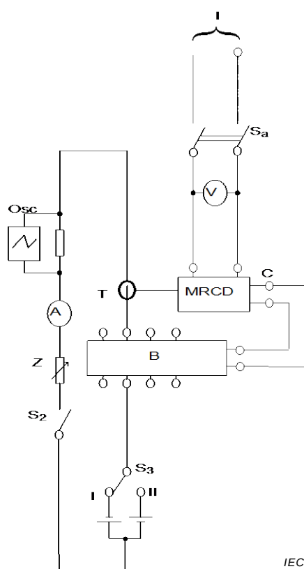
Figure M.13a) – MRCD avec un dispositif de détection séparé
