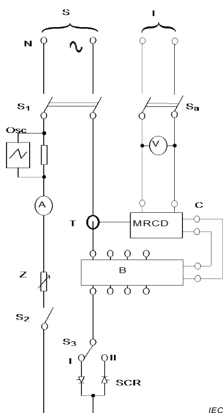
Figure M.9a) – MRCD avec un dispositif de détection séparé
