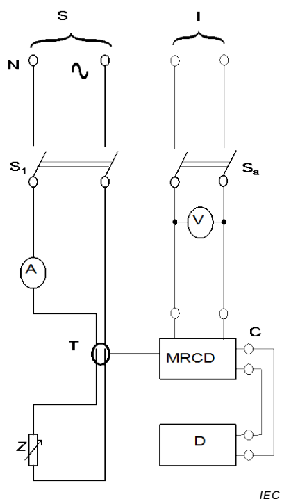
Figure M.4a) – MRCD avec un dispositif de détection séparé
