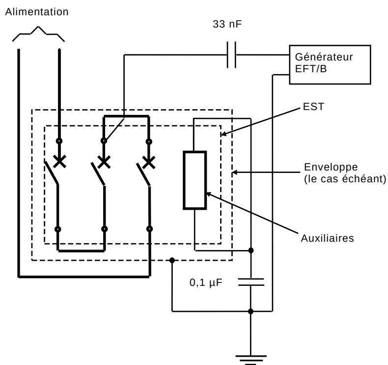
Figure F.7 – Circuit pour l'essai d'immunité aux transitoires électriques rapides en salves (TER/S) selon F.4.4 – Trois pôles de phase en série
