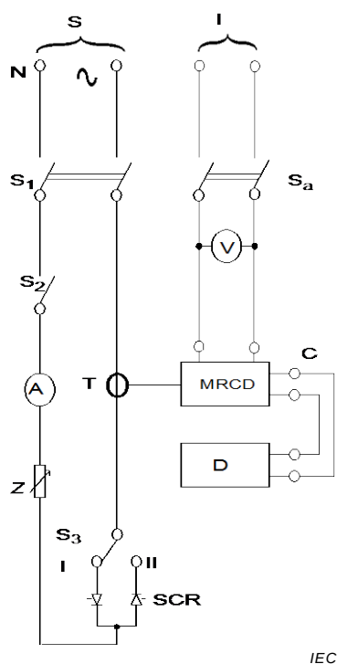
Figure M.7a) – MRCD avec un dispositif de détection séparé
