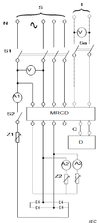
Figure M.15c) – MRCD de type à bornes
