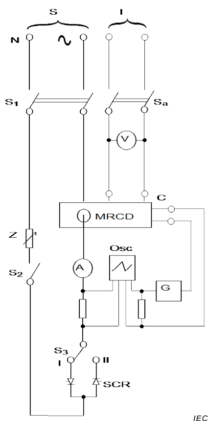
Figure M.8b) – MRCD avec un dispositif de détection intégré
