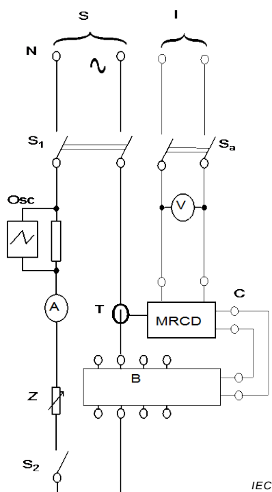
Figure M.2a) – MRCD avec un dispositif de détection séparé
