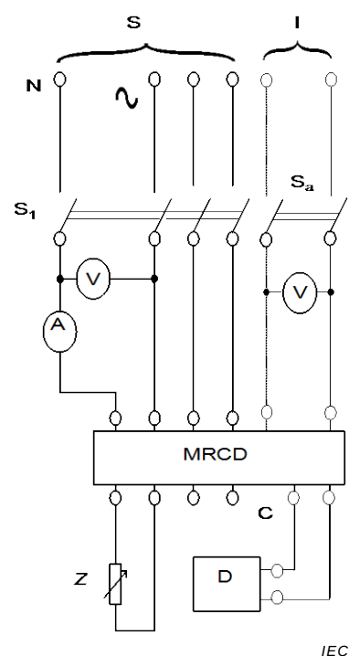
Figure M.4c) – MRCD de type à bornes
