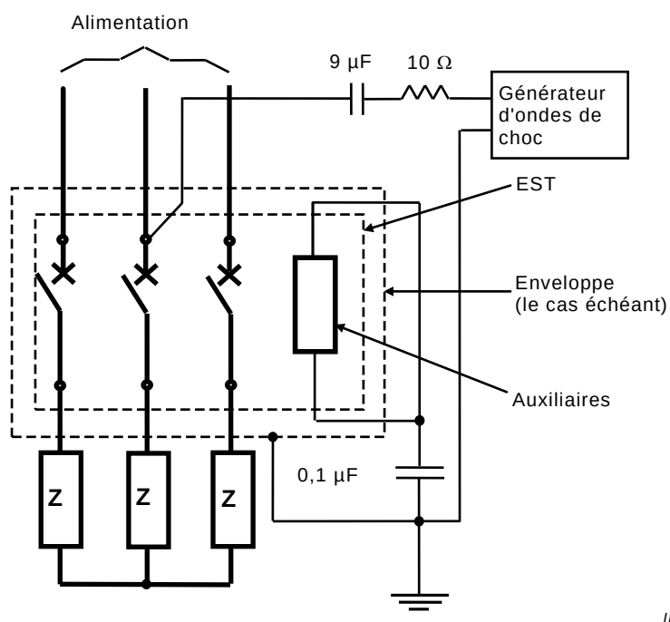
Figure F.10 – Circuit d'essai pour la vérification de l'influence des ondes de choc sur le circuit principal (phase-terre) selon F.4.5 – Trois pôles de phase en série
