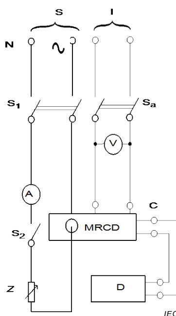
Figure M.1b) – MRCD avec un dispositif de détection intégré
