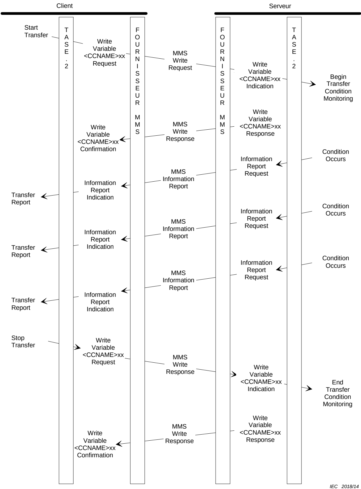
Figure F.1 – Séquence d'opérations et d'actions Transfer Set
