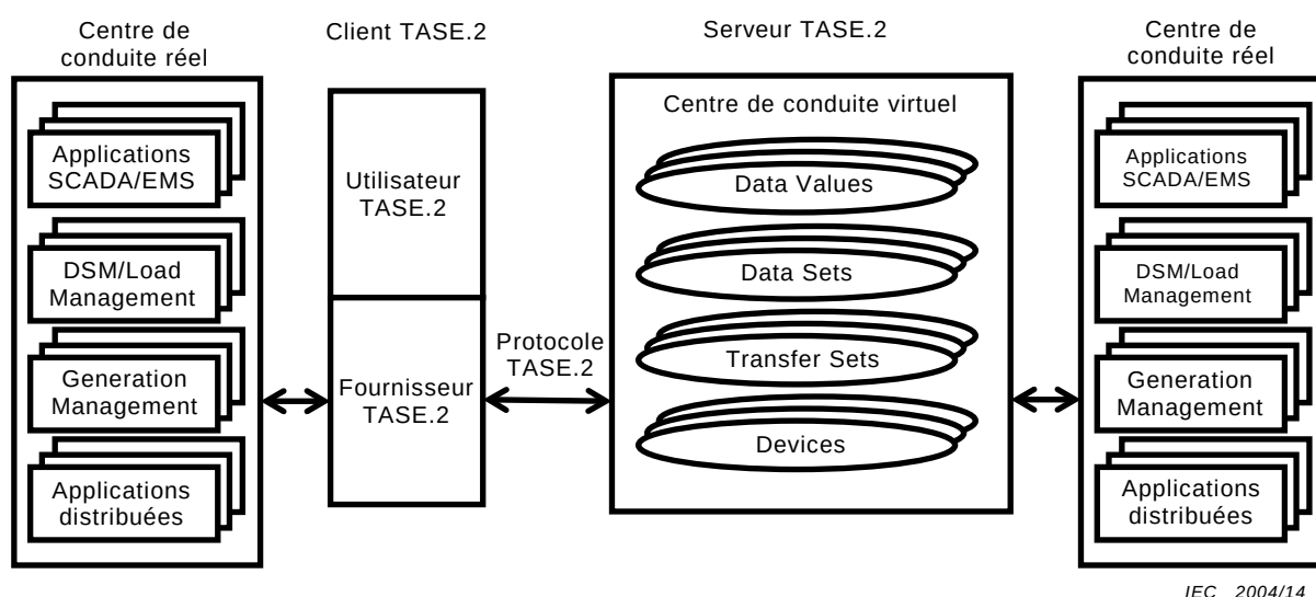
Figure 6 – Relations entre TASE.2 et centres de conduite réels
