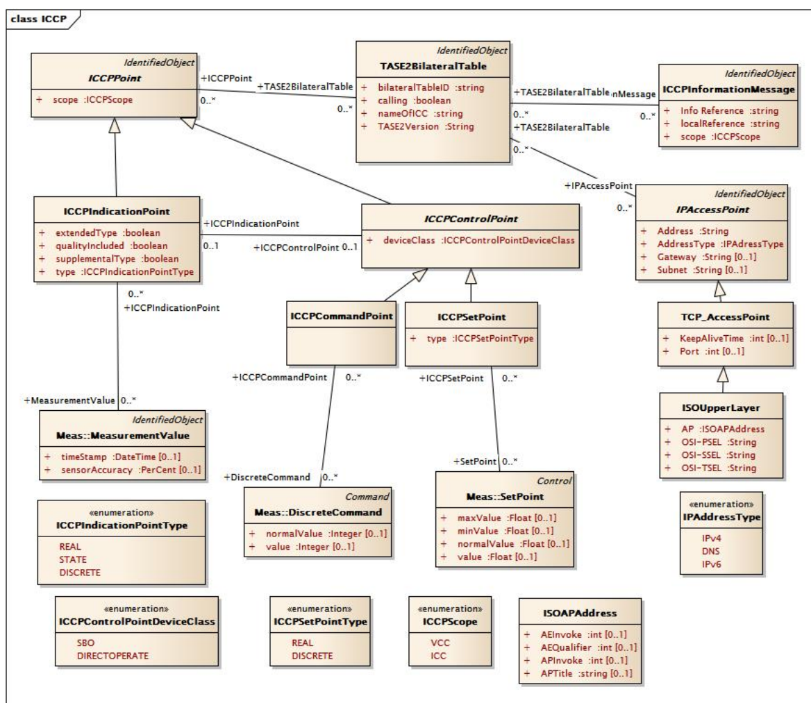
Figure 18 – Harmonisation sémantique CIM et ICCP
