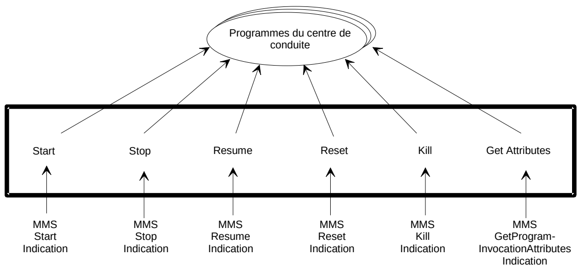
Figure F.3 – Séquence des opérations Program Invocation
