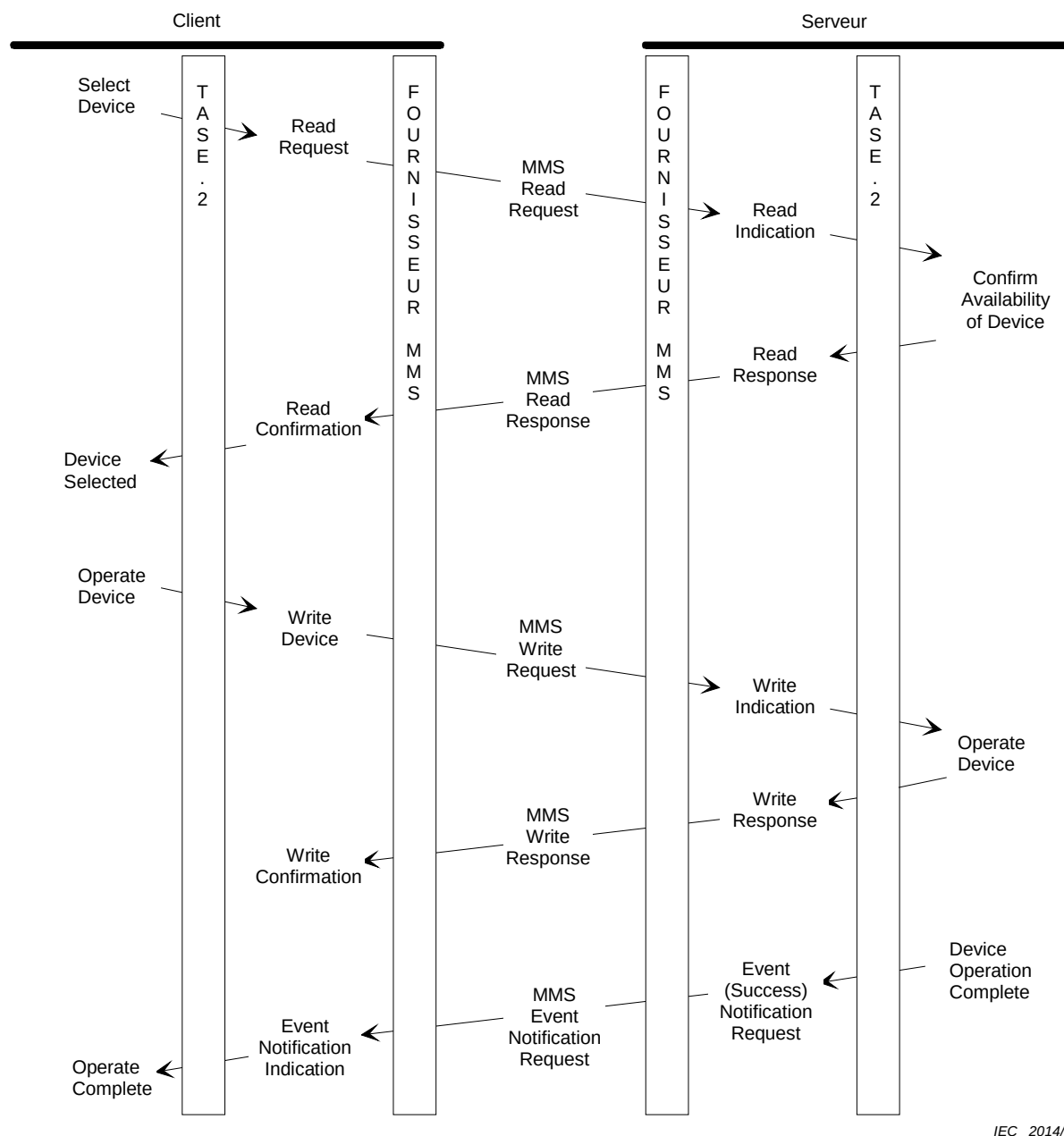
Figure 16 – Séquence de Device Control
