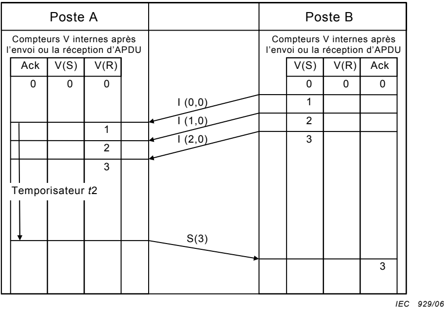
Figure 10 – Séquence non perturbée d'APDU de format numéroté I acquittée par un APDU de format S
