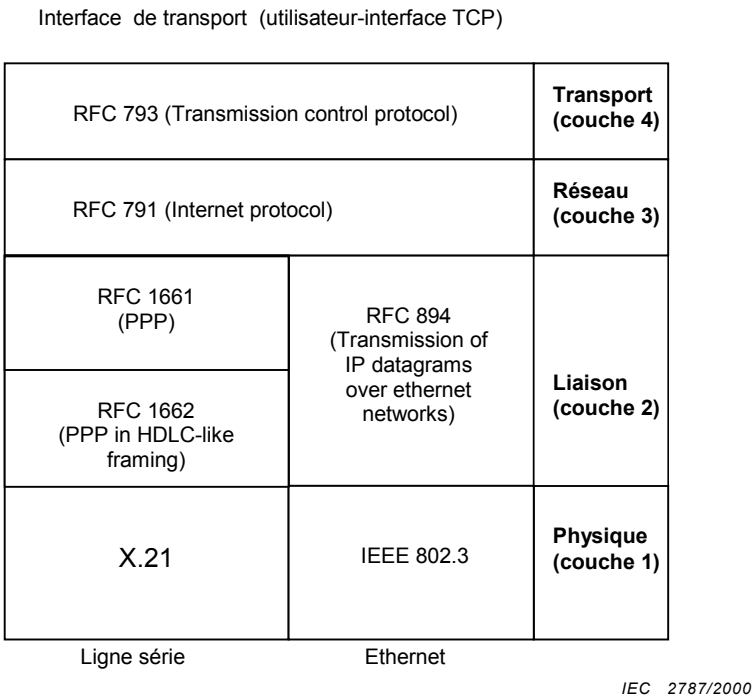
Figure 3 – Sélection dans l'ensemble des normes du protocole TCP/RFC 2200 (exemple)
