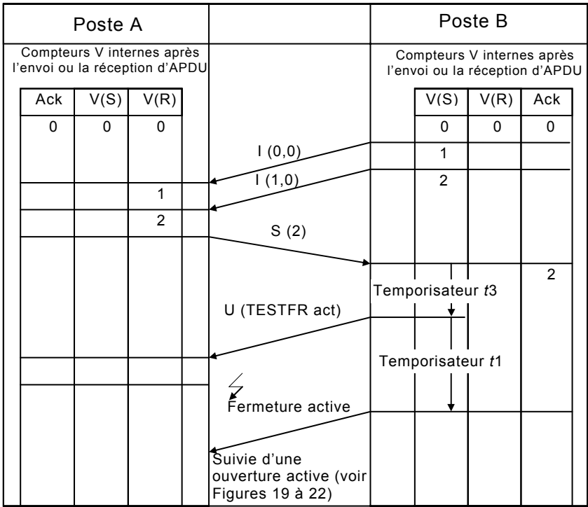
Figure 14 – Procédure d'essai non confirmée
