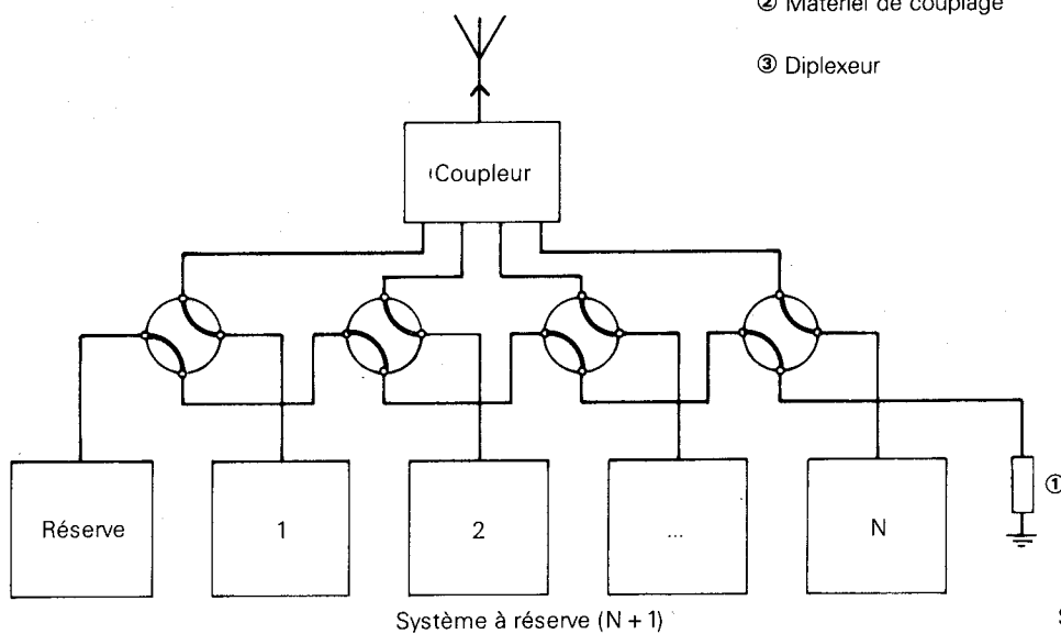
FIG. 3. — Schémas de principe des systèmes d'émetteurs communément utilisés.
