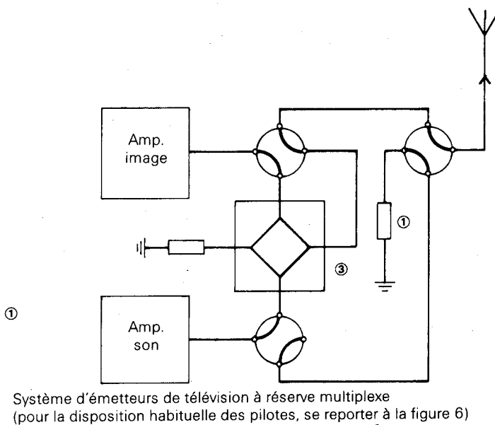
FIG. 3. — Schémas de principe des systèmes d'émetteurs communément utilisés.
