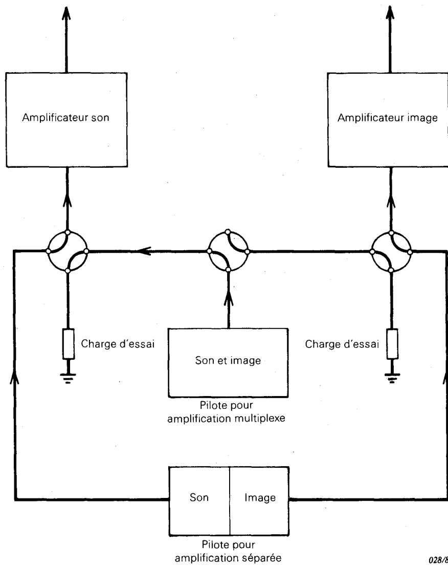
FIG. 6. — Disposition habituelle des pilotes d'un système d'émetteurs de télévision à réserve multiplexe.
