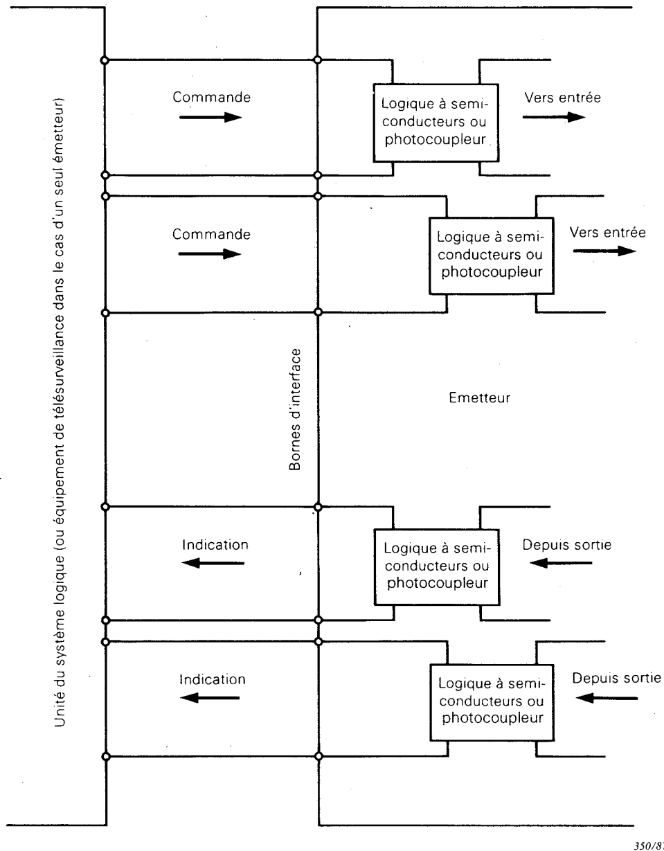
FIG. 5. — Principe des techniques d'interface à semiconducteurs et à photocoupleur.
