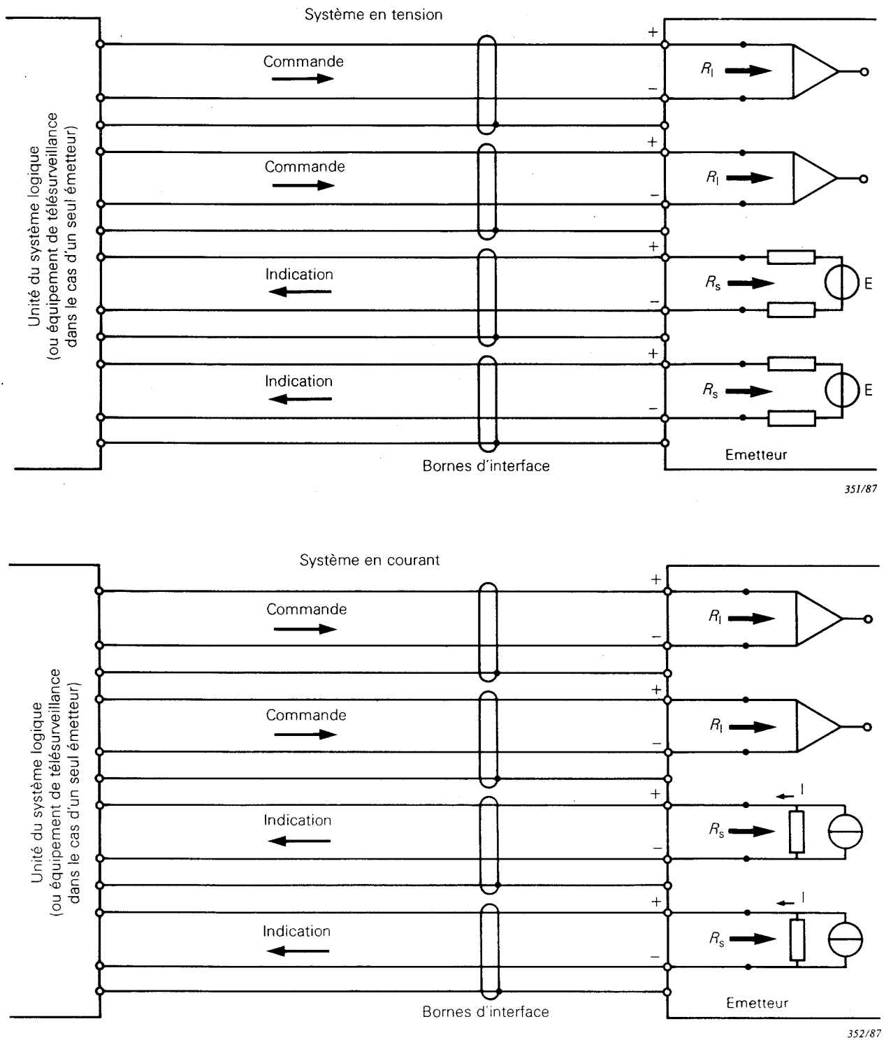
FIG. 7. — Exemple de la technique d'interface analogique.
