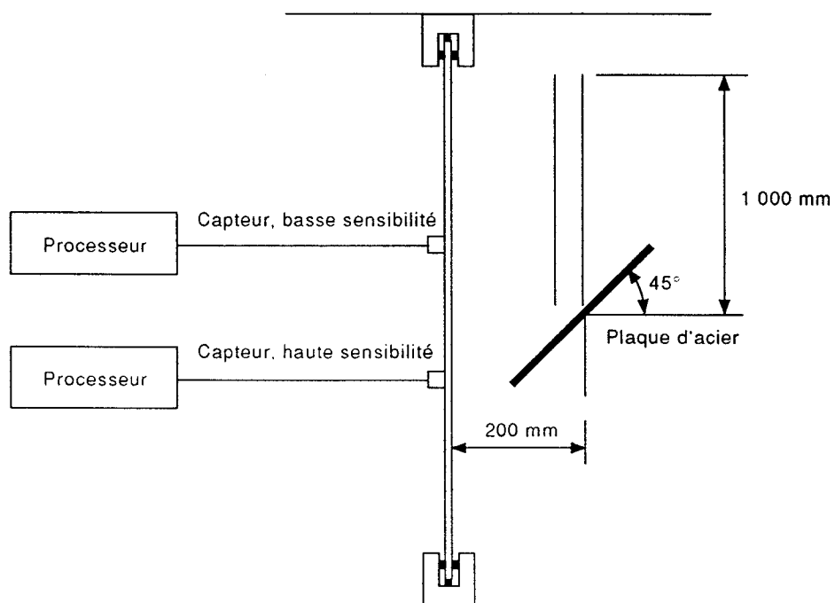
Figure 3 – Montage d'essai pour l'impact de balle
