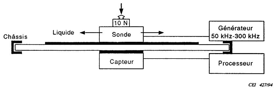
Figure 6 – Montage d'essai pour les essais de base
