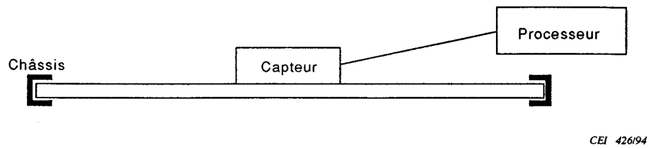
Figure 5 – Montage d'essai pour les essais du groupe 2
