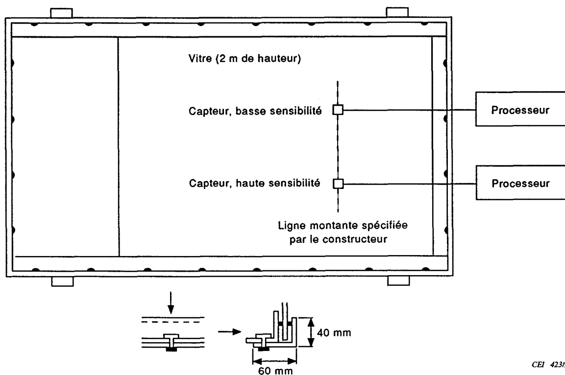
Figure 2 – Montage d'essai pour les essais du groupe 1
