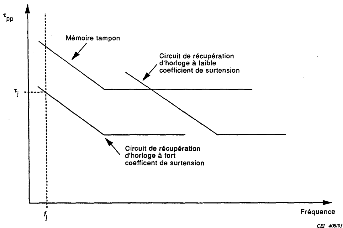
Figure 3 – Comparaison des caractéristiques de gigue tolérable entre l'entrée du circuit de récupération d'horloge et l'entrée du sous-ensemble à l'essai
