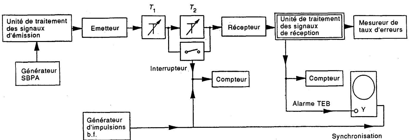
Figure 9 – Montage pour mesurer les caractéristiques de l'alarme sur le taux d'erreur (TEB)
