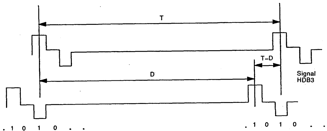
Figure 7b – Exemple de séquence binaire à utiliser pour évaluer le temps de propagation absolu
