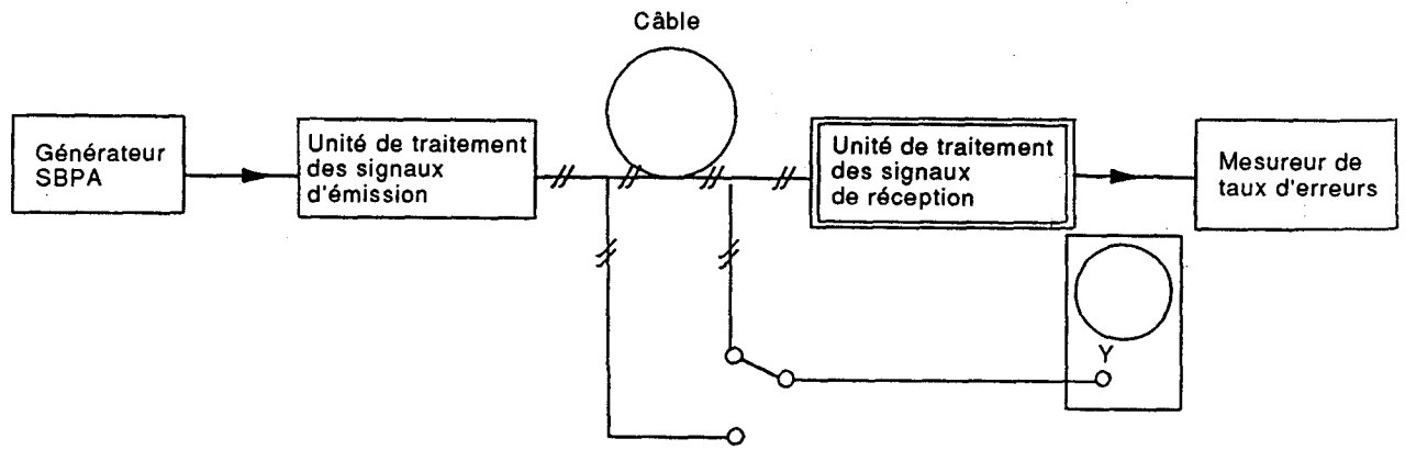
Figure 6 – Montage pour mesurer les caractéristiques acceptables du signal à l'entrée de l'unité de traitement des signaux de réception
