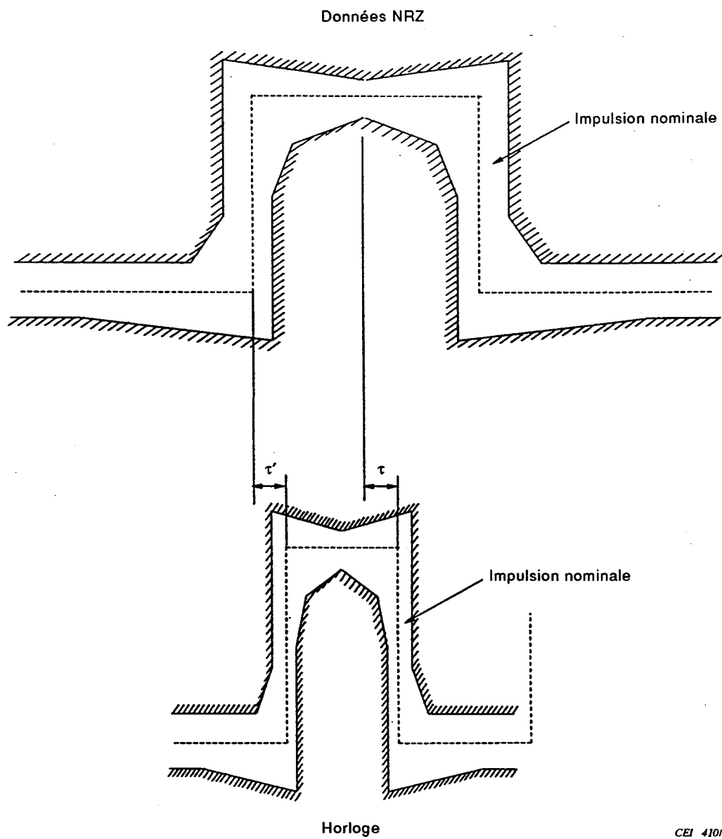
Figure 5 – Exemple de gabarits d'impulsion dans le cas de signaux NRZ et H (horloge)
