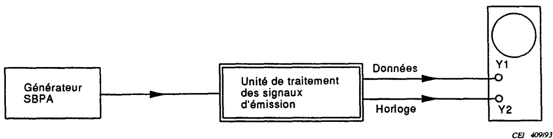
Figure 4 – Montage pour mesurer le niveau et la forme du signal à la sortie de l'unité de traitement des signaux d'émission
