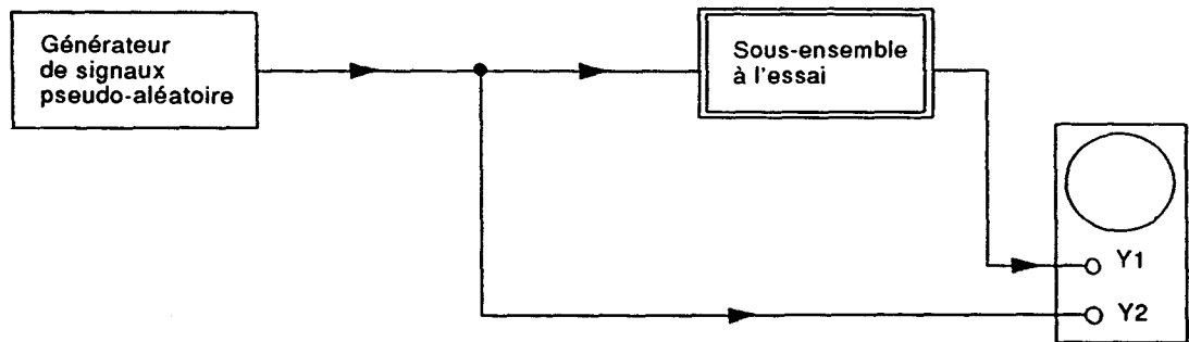
Figure 7a – Montage pour mesurer le temps de propagation absolu
