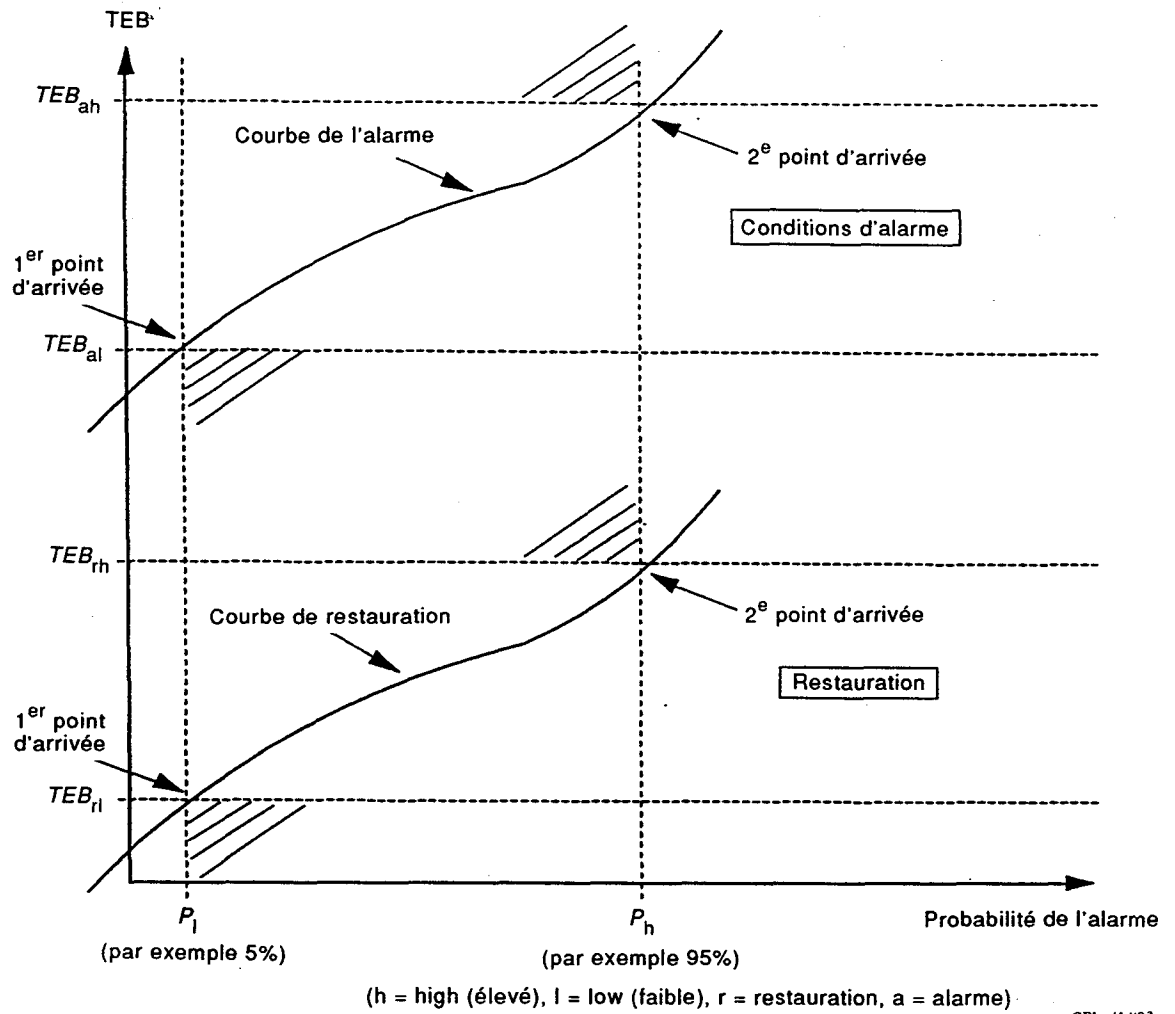
Figure 8 – Exemples de courbes pour l'évaluation des caractéristiques de l'alarme sur le taux d'erreur (TEB)
