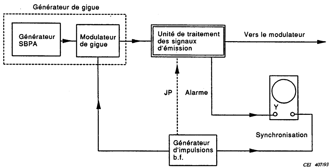
Figure 2 – Montage pour mesurer la constante de temps de l'alarme de dépassement de la capacité de la mémoire tampon
