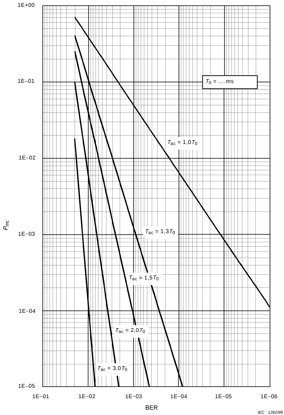
Figure 22 – Exemple de courbes de fiabilité pour une téléprotection numérique
