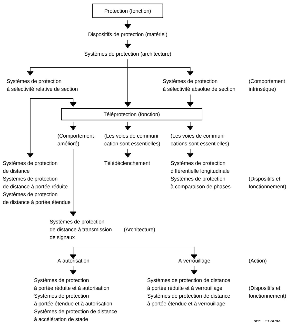
Figure 5 – Termes fondamentaux en protection et en téléprotection
