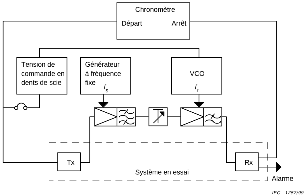
Figure 17 – Montage d'essai pour la mesure des perturbations par écart de fréquence
