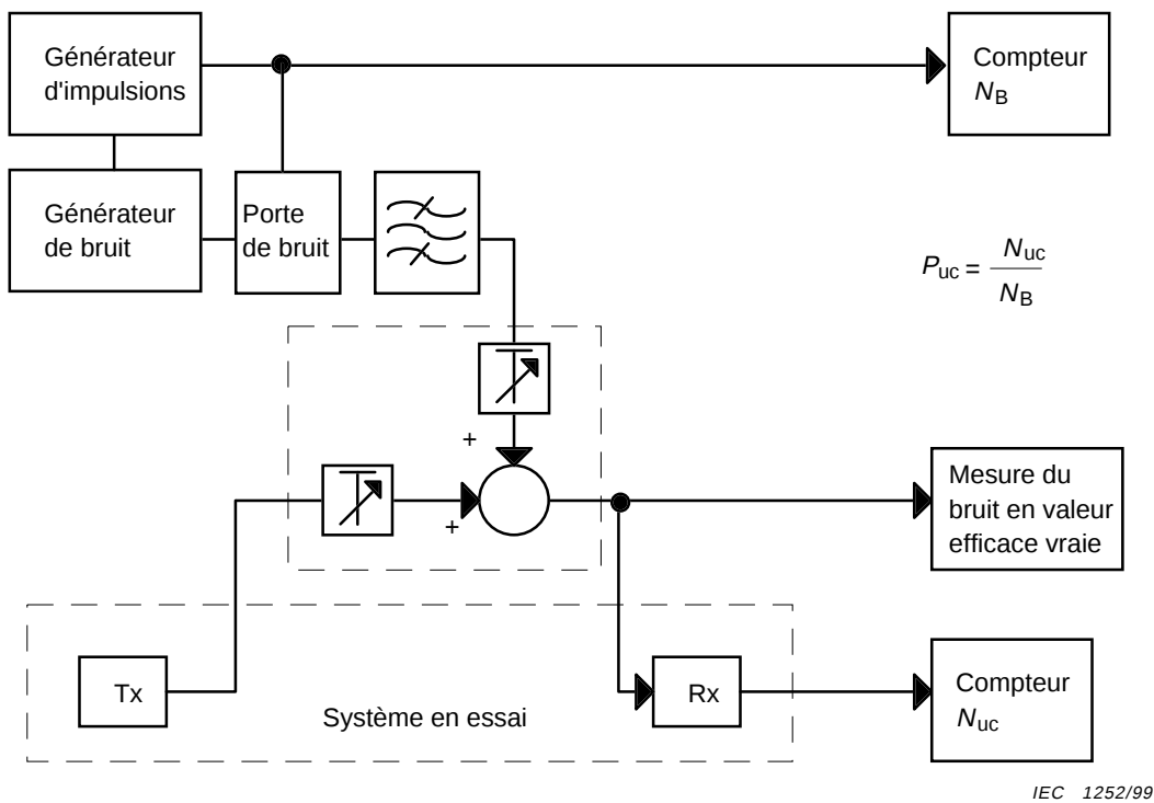
Figure 12 – Montage d'essai pour la mesure de la sécurité (téléprotection analogique)
