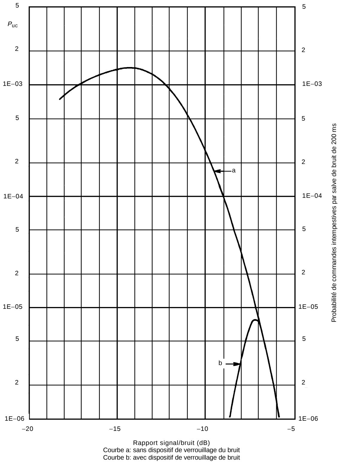
Figure 14 – Exemples de probabilité de commandes intempestives en fonction du rapport signal/bruit pour un canal de 200 Bd
