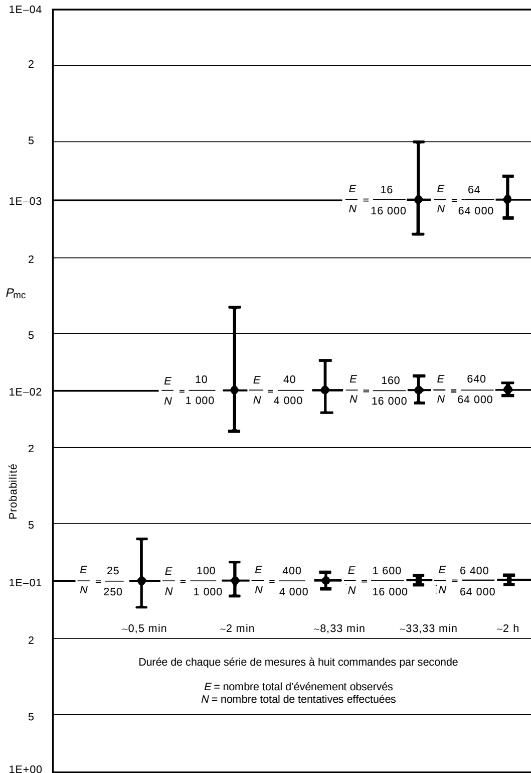
Figure A.1 – Graphique représentant l'incertitude de probabilité pour un niveau de confiance de 95 % pour diverses valeurs de E et de N
