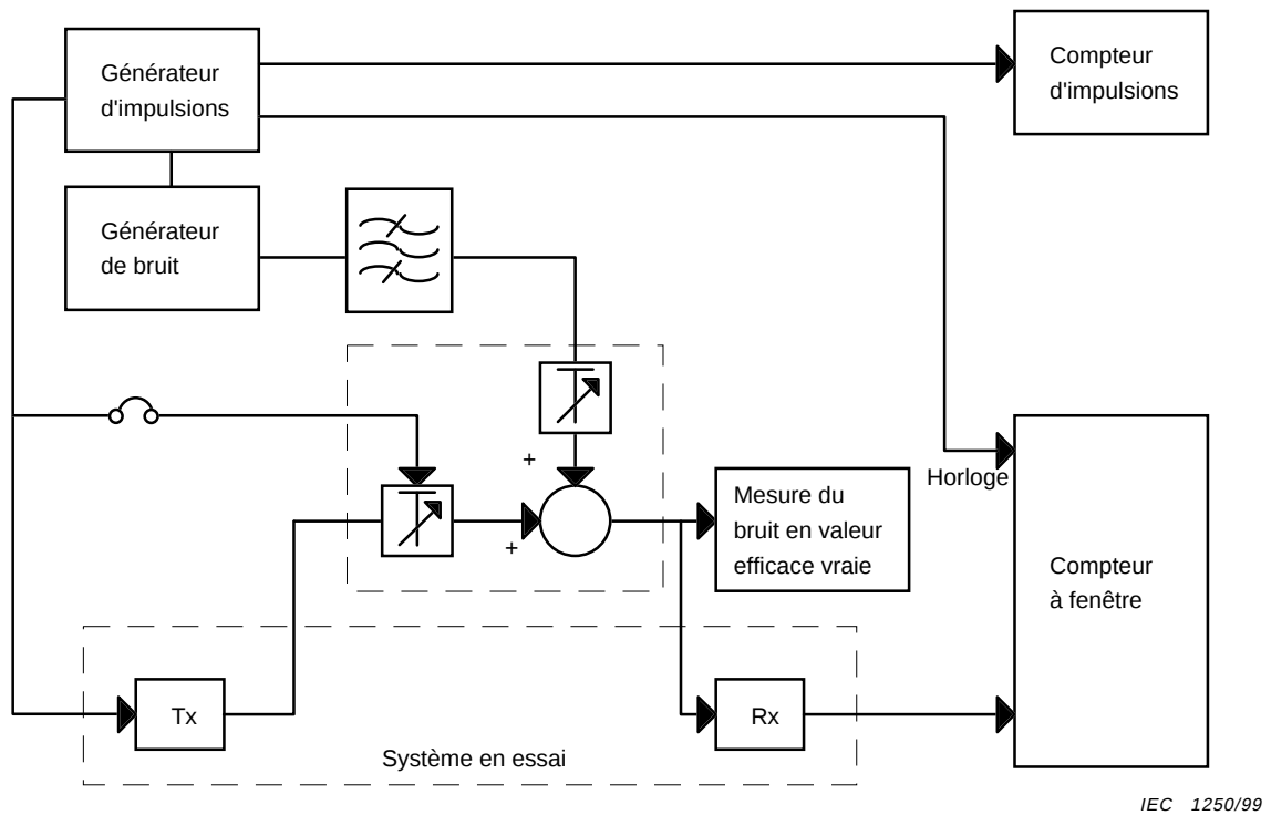
Figure 10 – Montage d'essai pour la mesure de la fiabilité (téléprotection analogique)
