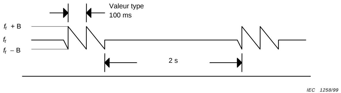
Figure 18 – Ecart de fréquence en fonction du temps pour le montage de la figure 17
