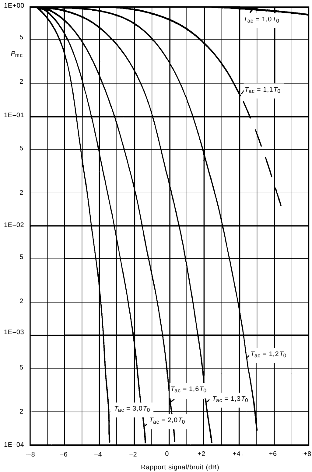
Figure 9 – Exemples de probabilité de commande défailante en fonction du rapport signal/bruit
