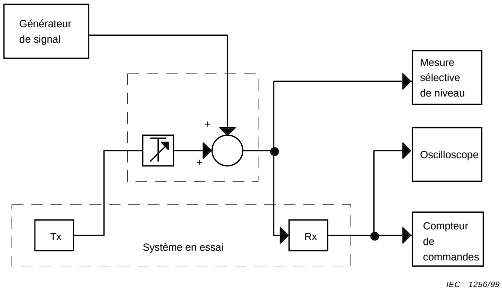
Figure 16 – Montage d'essai pour la mesure des perturbations par fréquences discrètes
