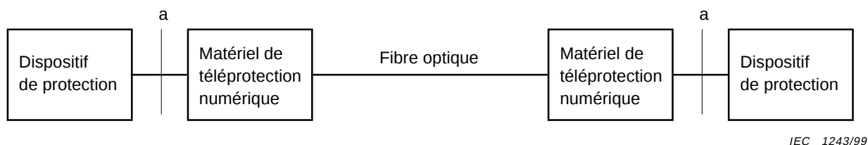
Figure 3 – Téléprotection numérique connectée directement (exemple)
