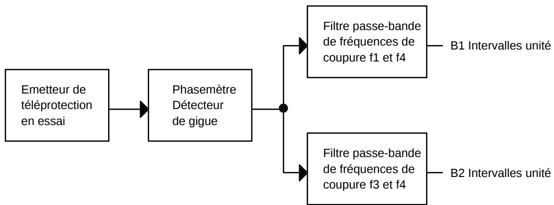
Figure 24 – Montage d'essai pour la mesure de la gigue à la sortie d'un émetteur de téléprotection numérique
