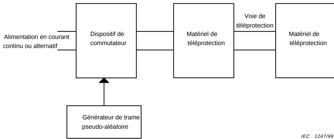
Figure 7 – Circuit pour l'essai des interruptions d'alimentation
