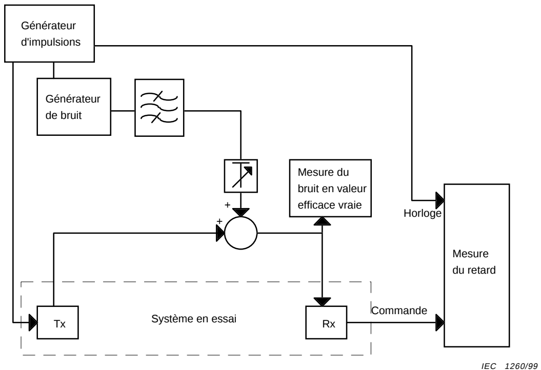
Figure 20 – Montage d'essai pour la mesure du temps de rétablissement pour une téléprotection analogique
