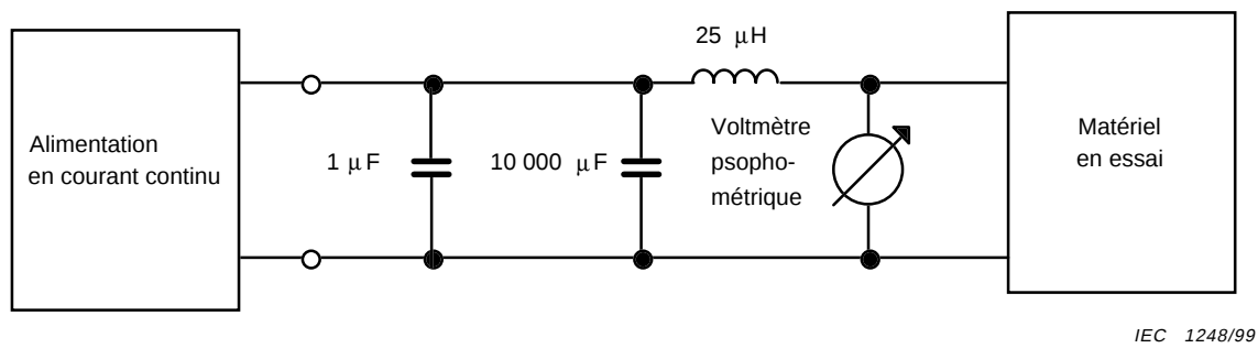
Figure 8 – Circuit d'essai pour la mesure de l'émission de perturbations BF
