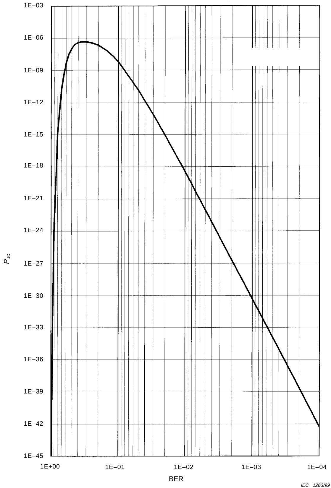
Figure 23 – Exemple de courbes de sécurité pour une téléprotection numérique
