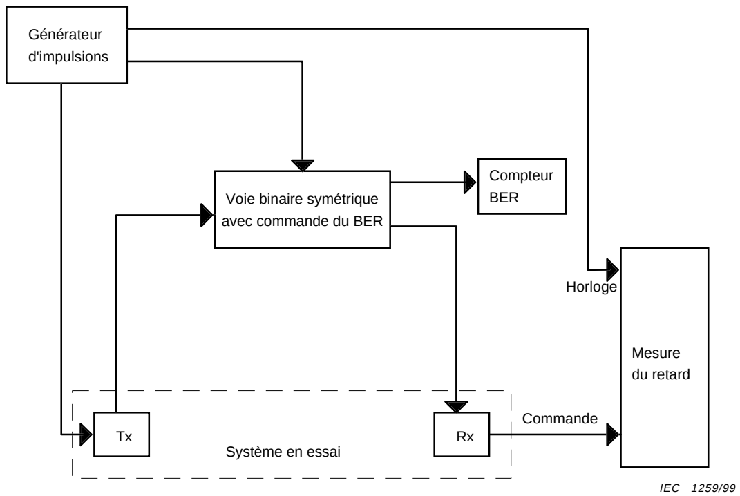
Figure 19 – Montage d'essai pour la mesure du temps de rétablissement pour une téléprotection numérique
