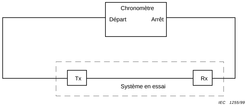
Figure 15 – Montage d'essai pour la mesure du temps de transmission
