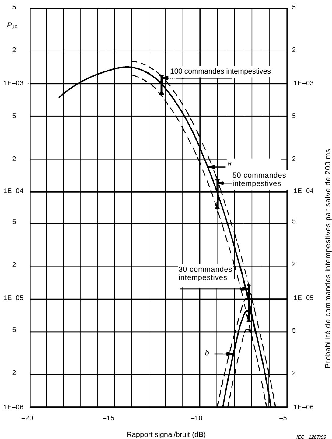
Figure A.2 – Exemples de probabilité de commandes intempestives en fonction du rapport signal/bruit pour un canal de 200 Bd
