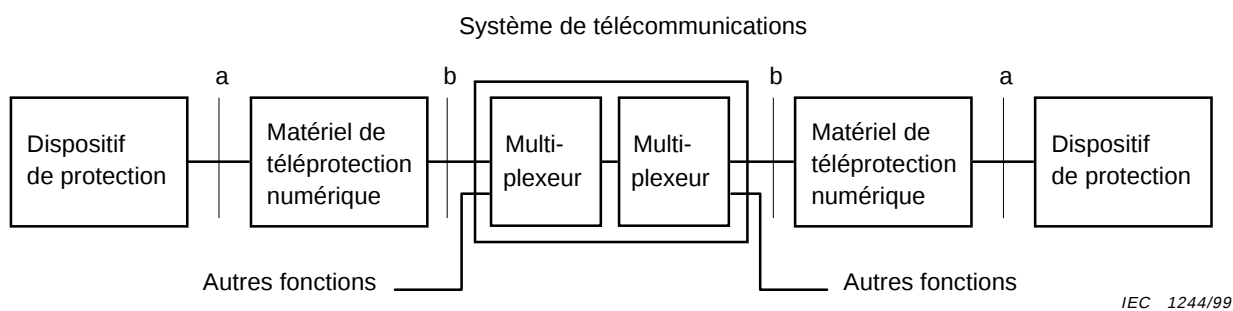
Figure 4 – Téléprotection numérique connectée à travers un système de communication multiplexé
