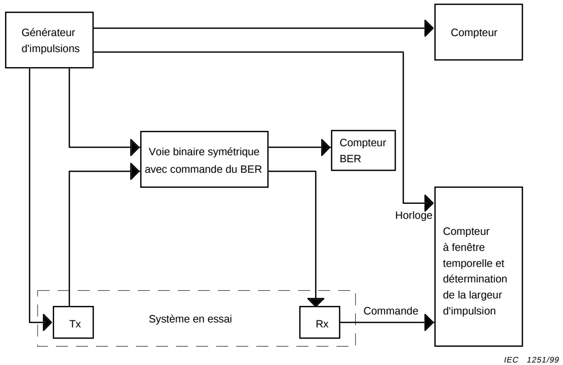
Figure 11 – Montage d'essai pour la mesure de la fiabilité (téléprotection numérique)
