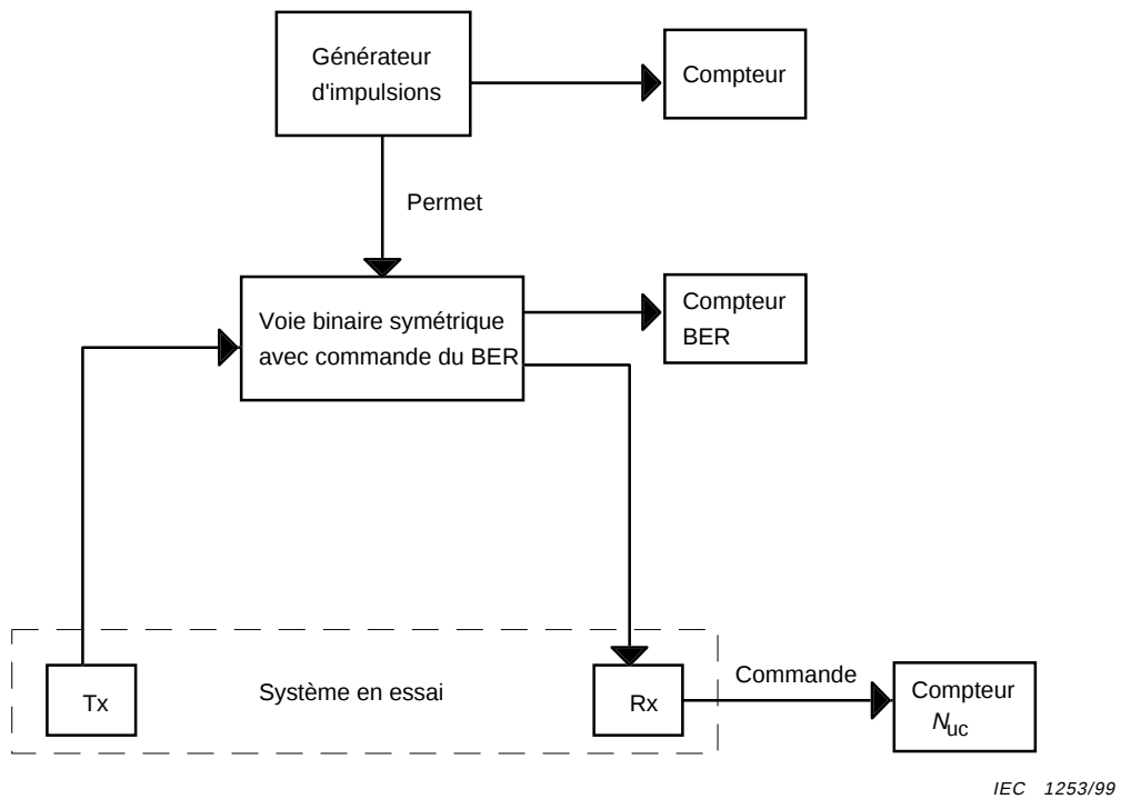
Figure 13 – Montage d'essai pour la mesure de la sécurité (téléprotection numérique)
