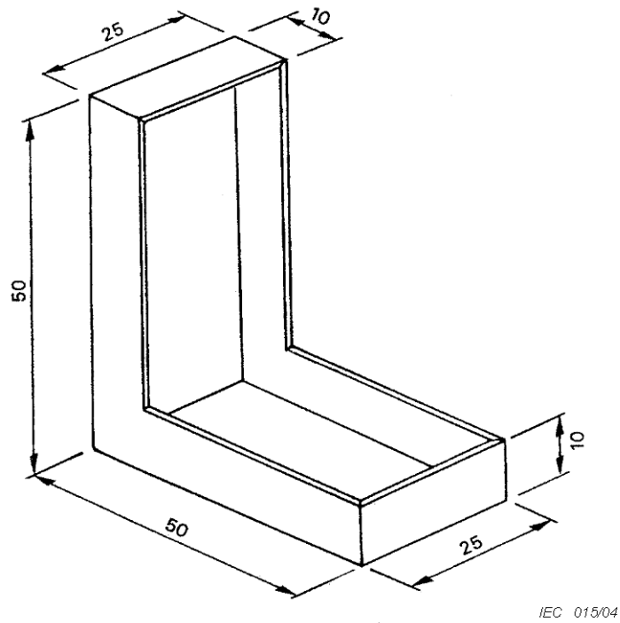
Figure 1 – Boîte angulaire avec deux parties rectangulaires
