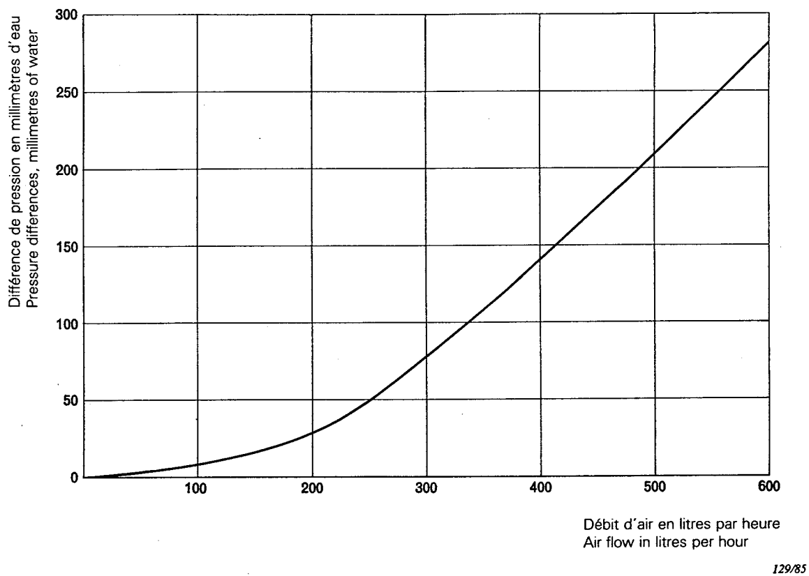
FIG. 2.— Diagramme d'étalonnage du tube capillaire (diamètre: d = 2 mm; longueur: l = 70 mm) du débitmètre pour le contrôle du débit d'air dans les étuves par la méthode 2. Calibration diagram of the capillary tube (diameter: d = 2 mm; length: l = 70 mm) of the flowmeter for air-flow control in air ovens for method 2.
