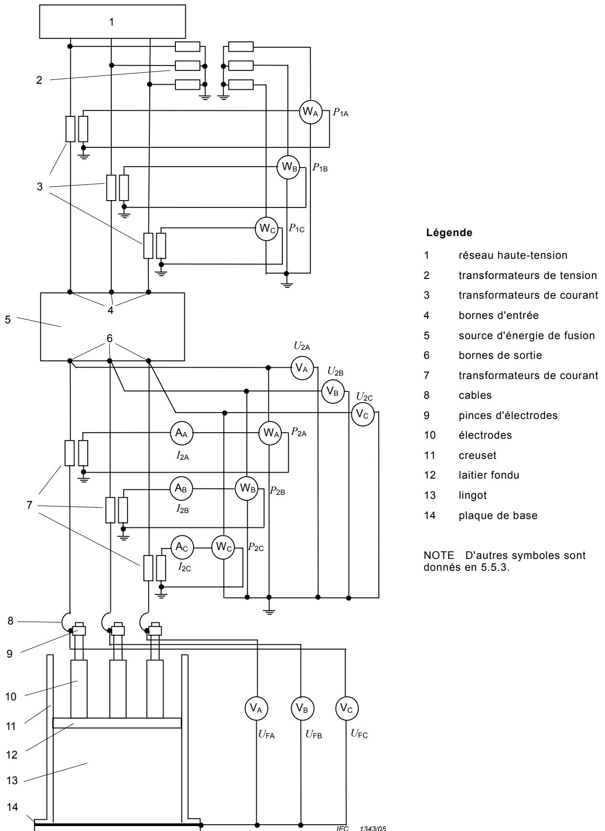
Figure 2 – Exemple d'un circuit triphasé pour un four de refusion sous laitier électroconducteur
