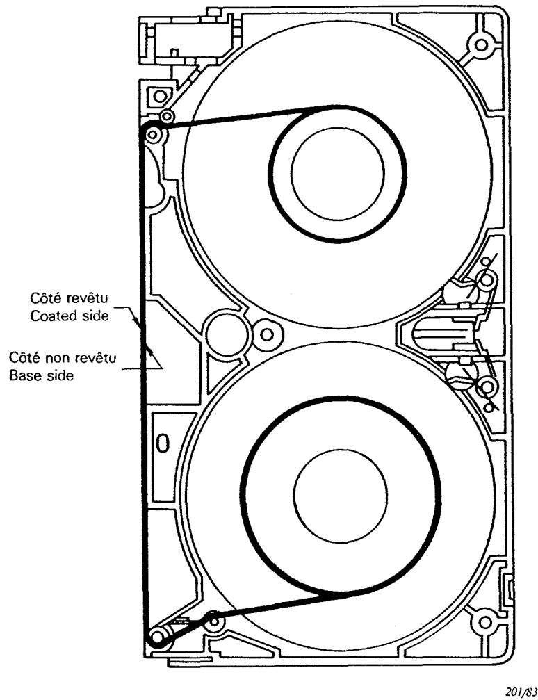
Figure 6 – Enroulement et parcours de la bande Tape winding and tape path
