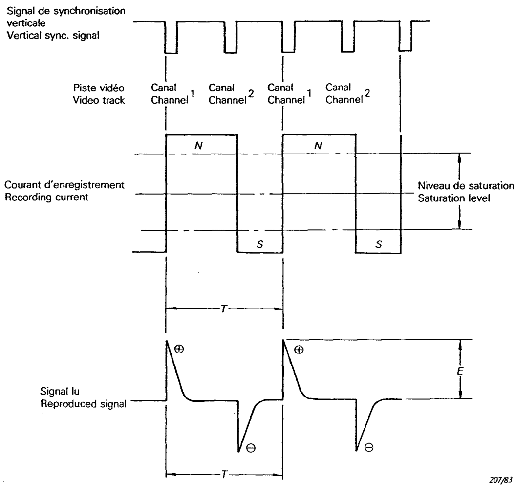
Figure 24 – Forme d'onde et polarité du signal d'asservissement Control signal wave-form and polarity
