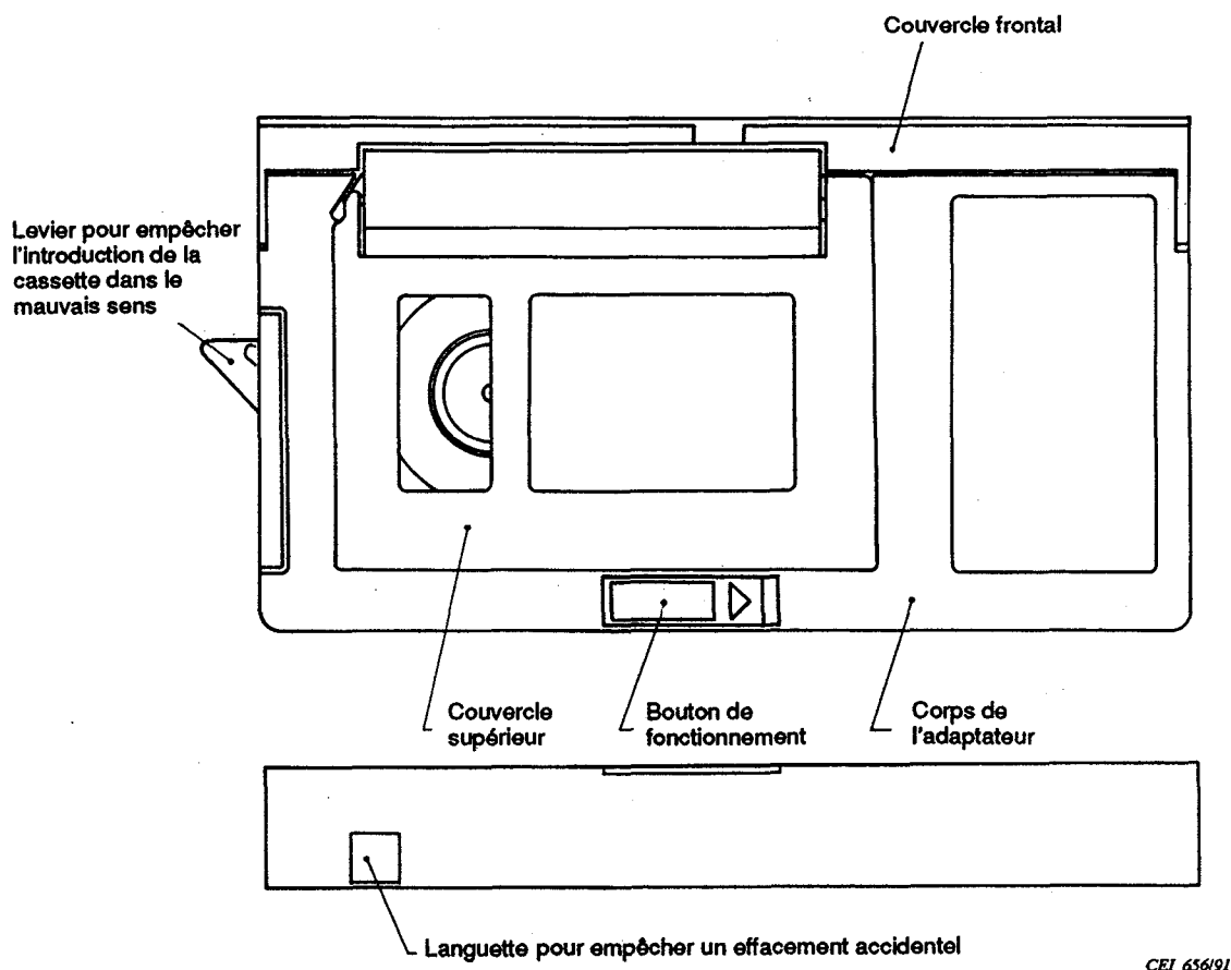
Figure D.1 – Exemple d'adaptateur de cassette vidéo compacte
