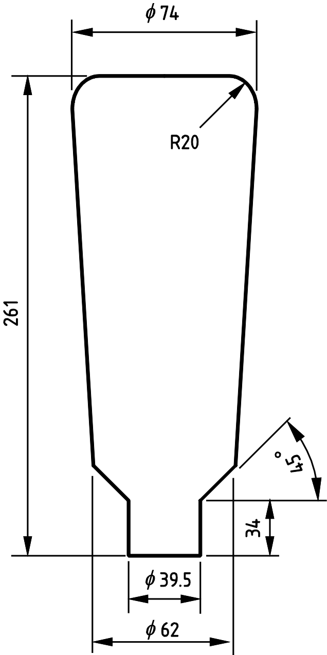
25001: 250 W, tubulaire, culot E40
