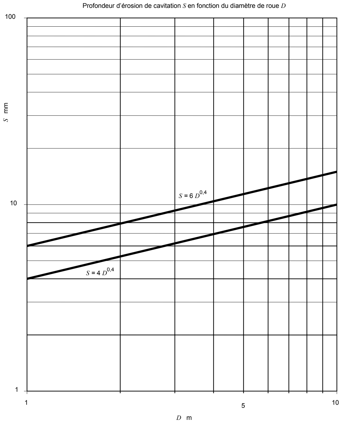
Figure A.1 – Exemples de valeurs maximales admissibles de la profondeur d'érosion de cavitation S sur les roues
