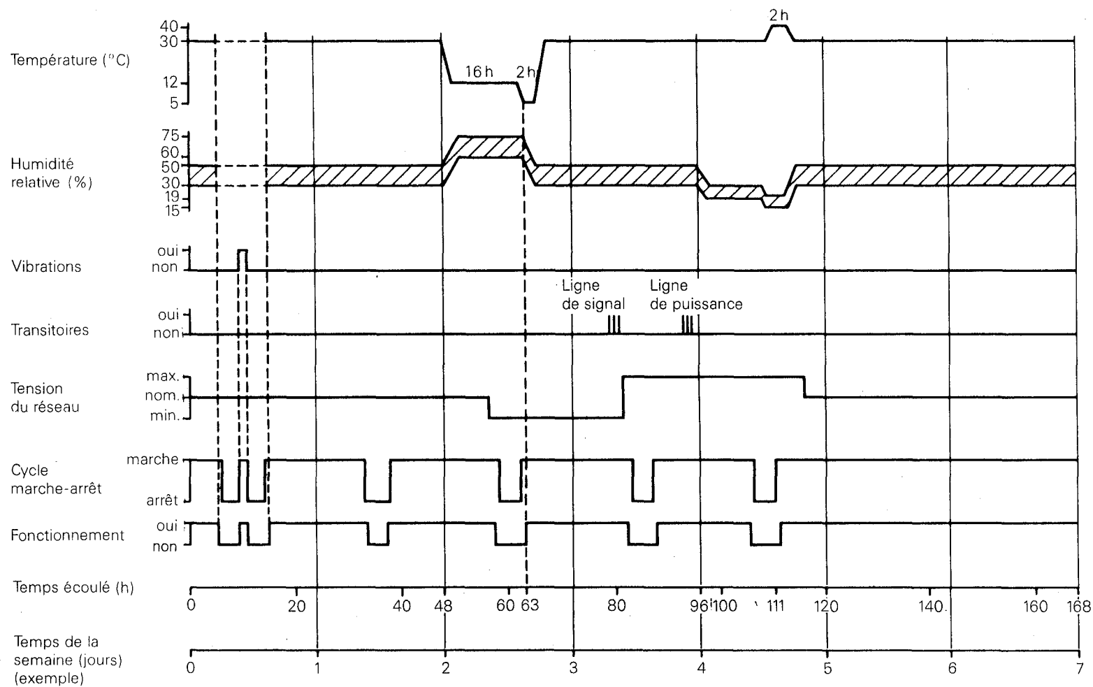
FIG. 2. — Diagramme du cycle d'essai décrit à l'article 6.
