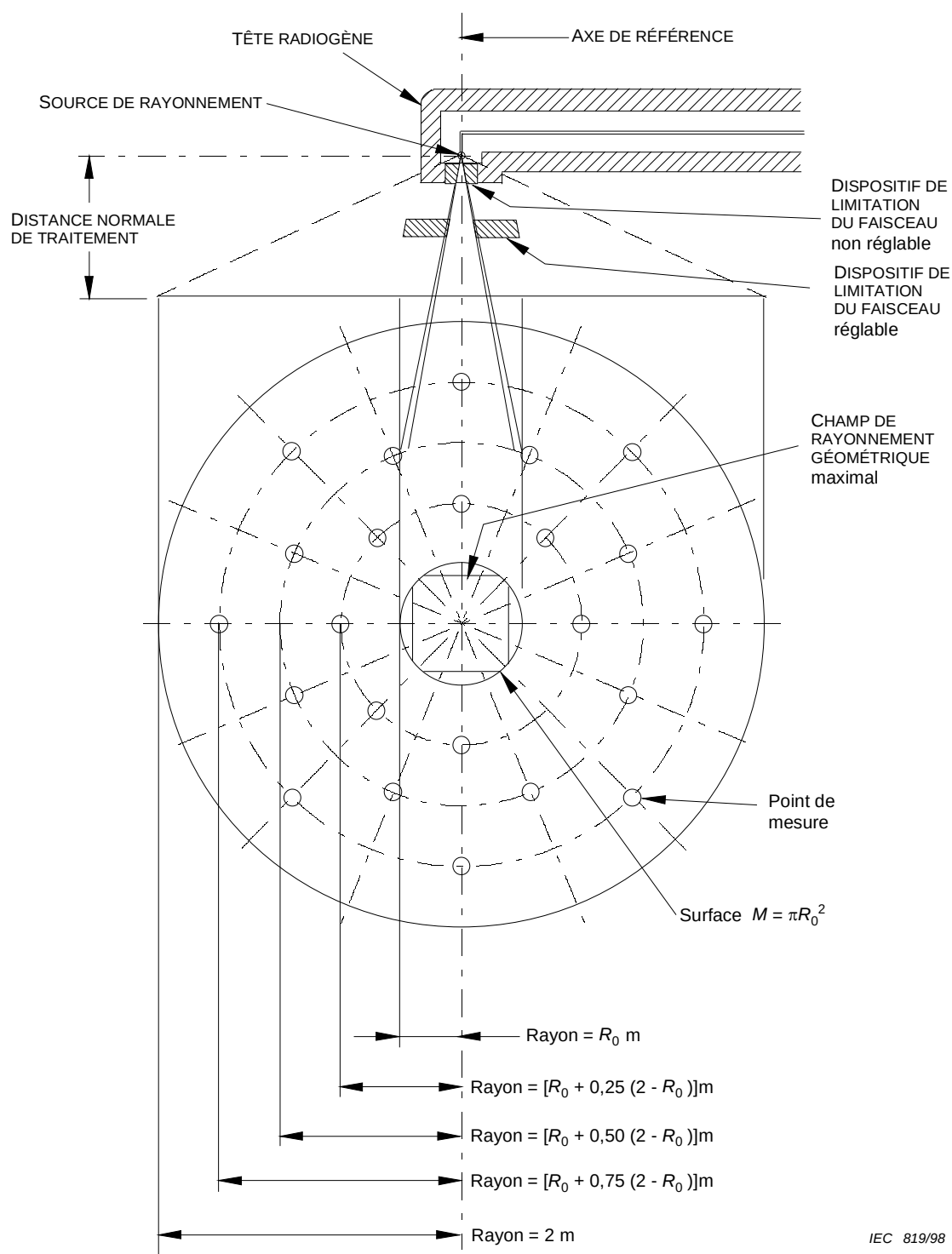
Figure 201.107 – Les 24 points de mesure pour déterminer la valeur moyenne du RAYONNEMENT DE FUITE à l'extérieur de la surface M (201.10.1.2.103.3)
