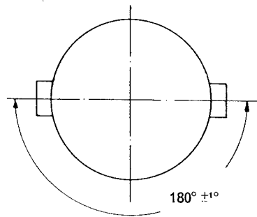
CONNECTEUR DE TYPE B TYPE B CONNECTOR
