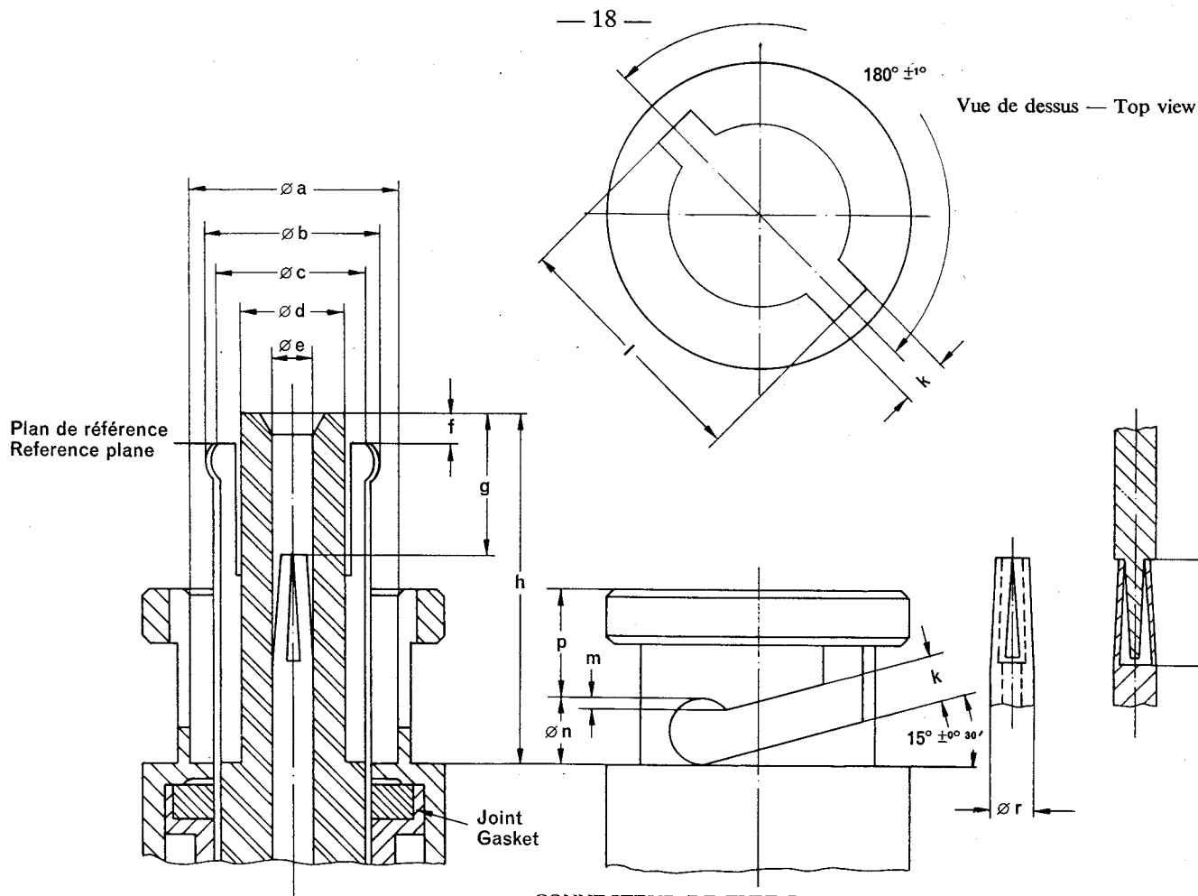
FIG. 10. — Connecteur à douille de contact Socket contact connector
