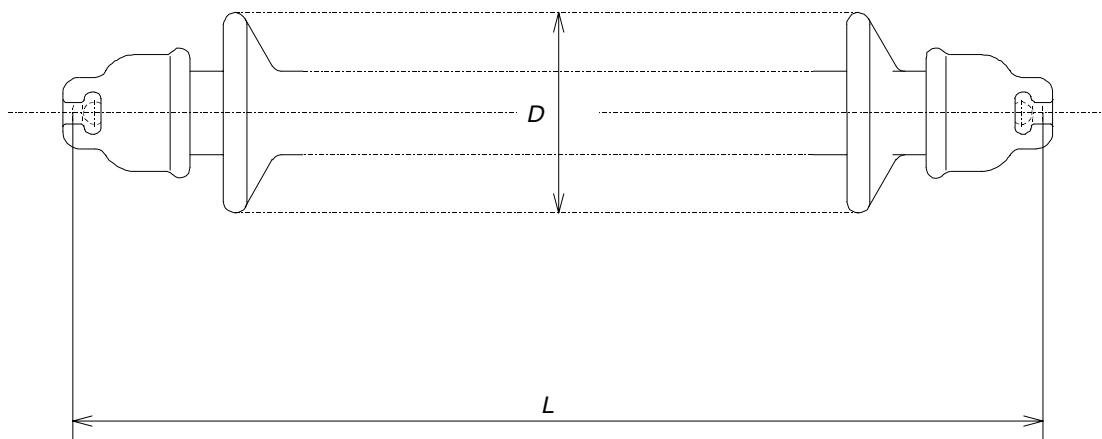
Figure 2 – Élément de chaîne à fût long avec assemblages à logement de rotule, type B
