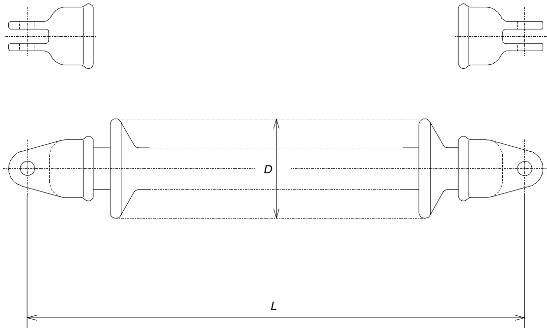
Figure 1 – Élément de chaîne à fût long avec assemblages à chape, type C
