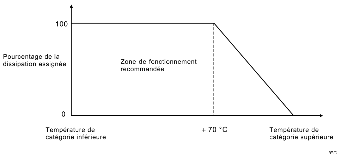
Figure 1 – Courbe de dissipation assignée
