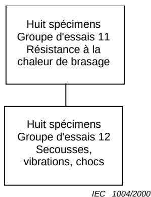
Figure 9 – Programme d'essais des CQC pour le montage
