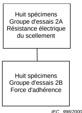
Figure 3 – Programme d'essais des CQC pour le scellement
