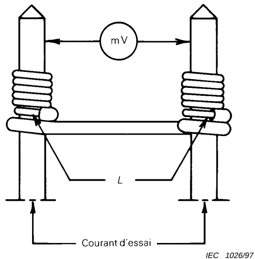
Figure 8b – Connexions enroulées renforcées
