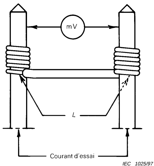
Figure 8a – Connexions enroulées simples
