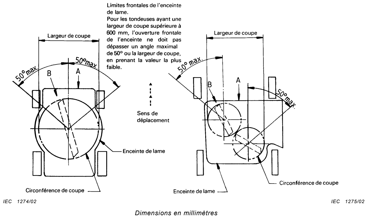
Figure 102 – Limites de l'ouverture frontale pour tondeuses à une seule lame
