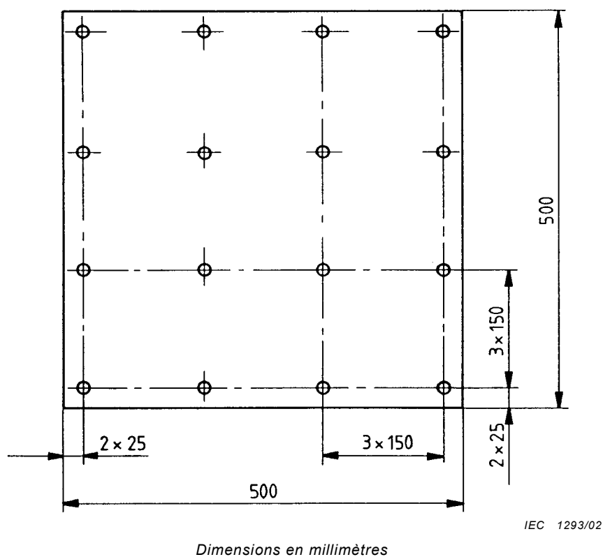
Figure CC.2 – Plan de clouage du support du dispositif d'essai
