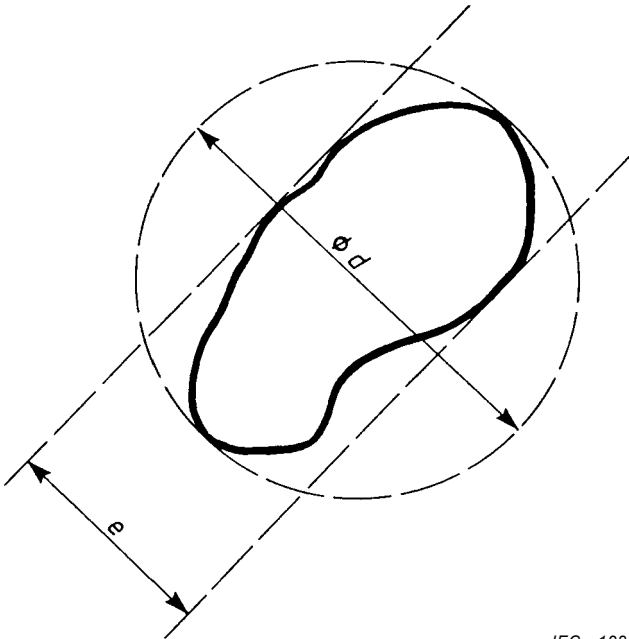
Figure AA.1 – Détermination de l'ouverture nominale
